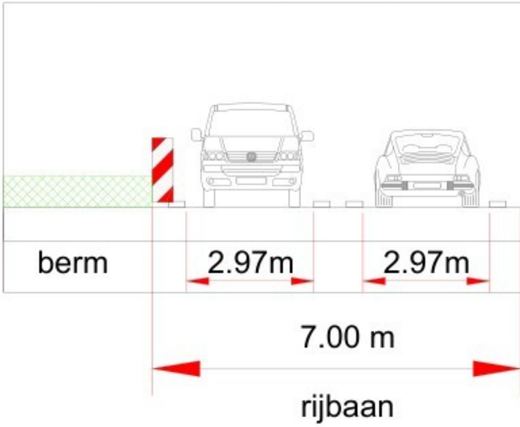
Dwarsdoorsnede A-A
