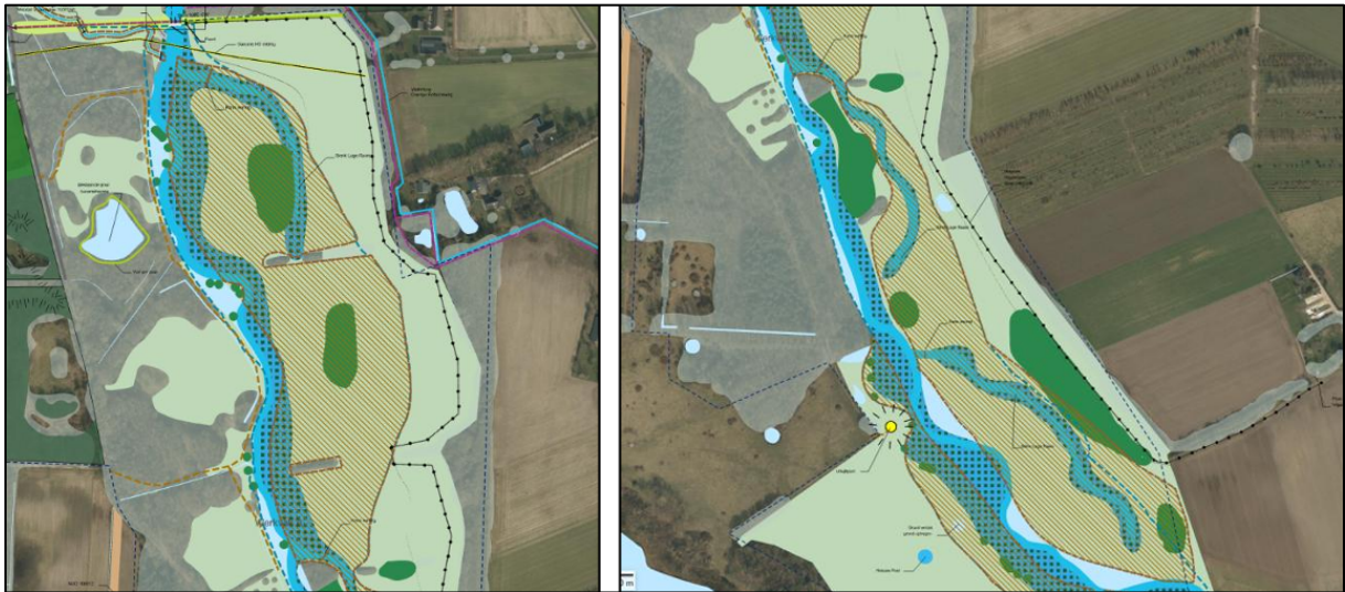
Figuur 3. Werkzaamheden locatie 1. Op de linker afbeelding is het noordelijke deel afgebeeld. Op de rechter afbeelding het zuidelijke deel. De aan te leggen geulen (blauw weergegeven) zijn korte, doodlopende zijgeulen die aansluiten op de bestaande watergang. Ze vormen verlengingen van de watergang, maar hebben geen doorgaande verbinding.
