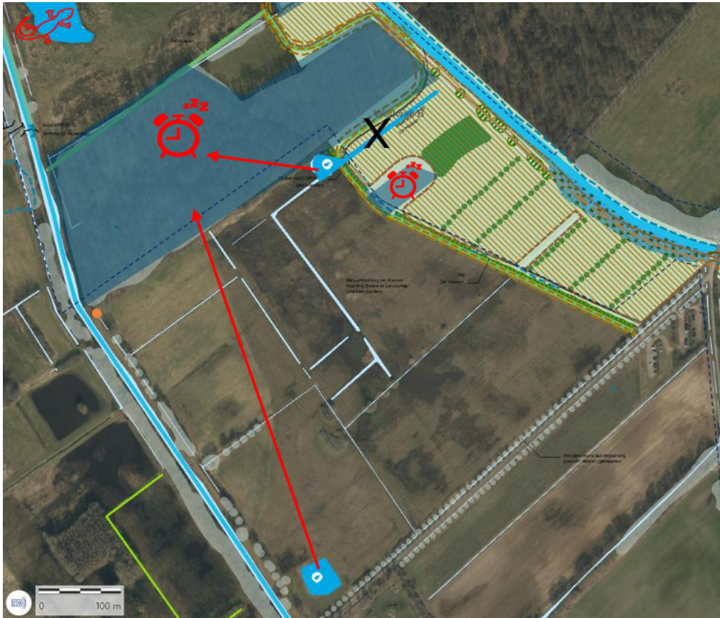
Figuur 5. Werkzaamheden locatie 4 en 5.
