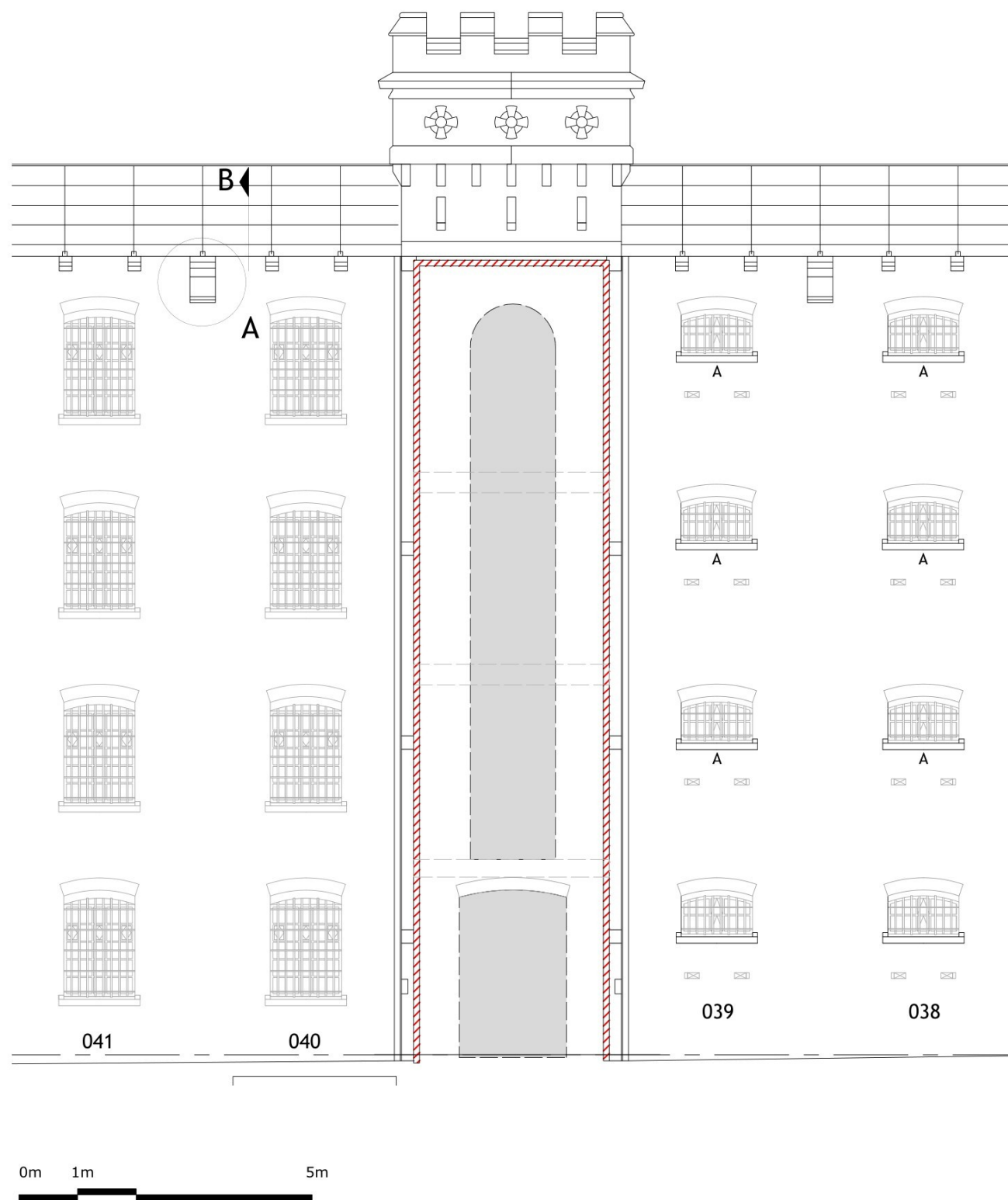
Toren noord - Sloop aansluiting met gebouw A (de Koepelgevangenis)
