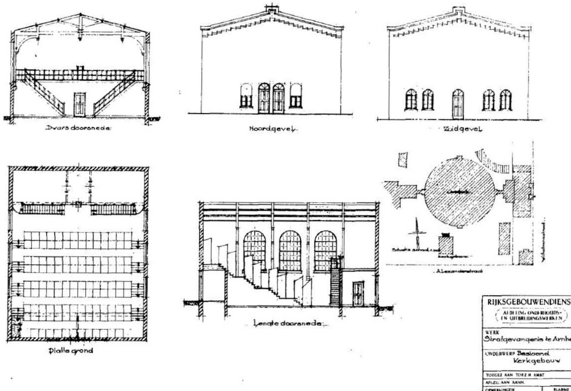
Bouwtekening van de bestaande situatie van de kapel omstreeks 1950
