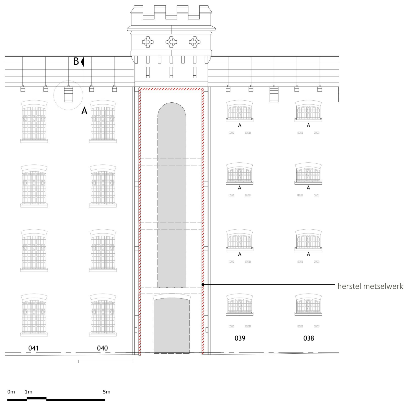
Toren noord - bestaande situatie
