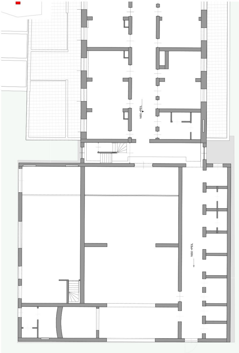
plattegrond - begane grond - bestaande situatie
