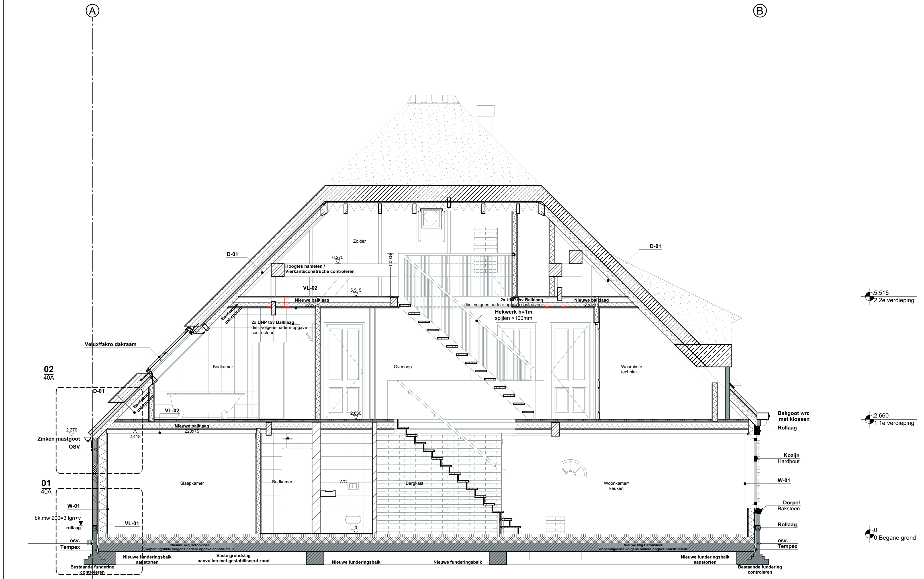
Doorsnede A-A
