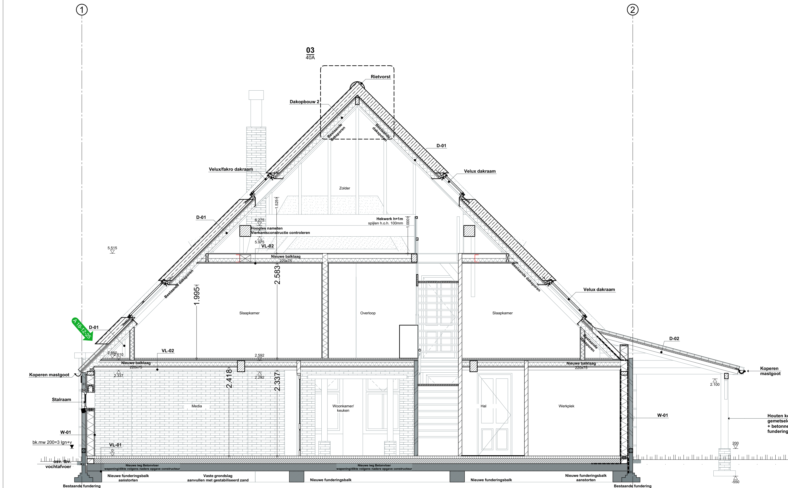
Doorsnede B-B
