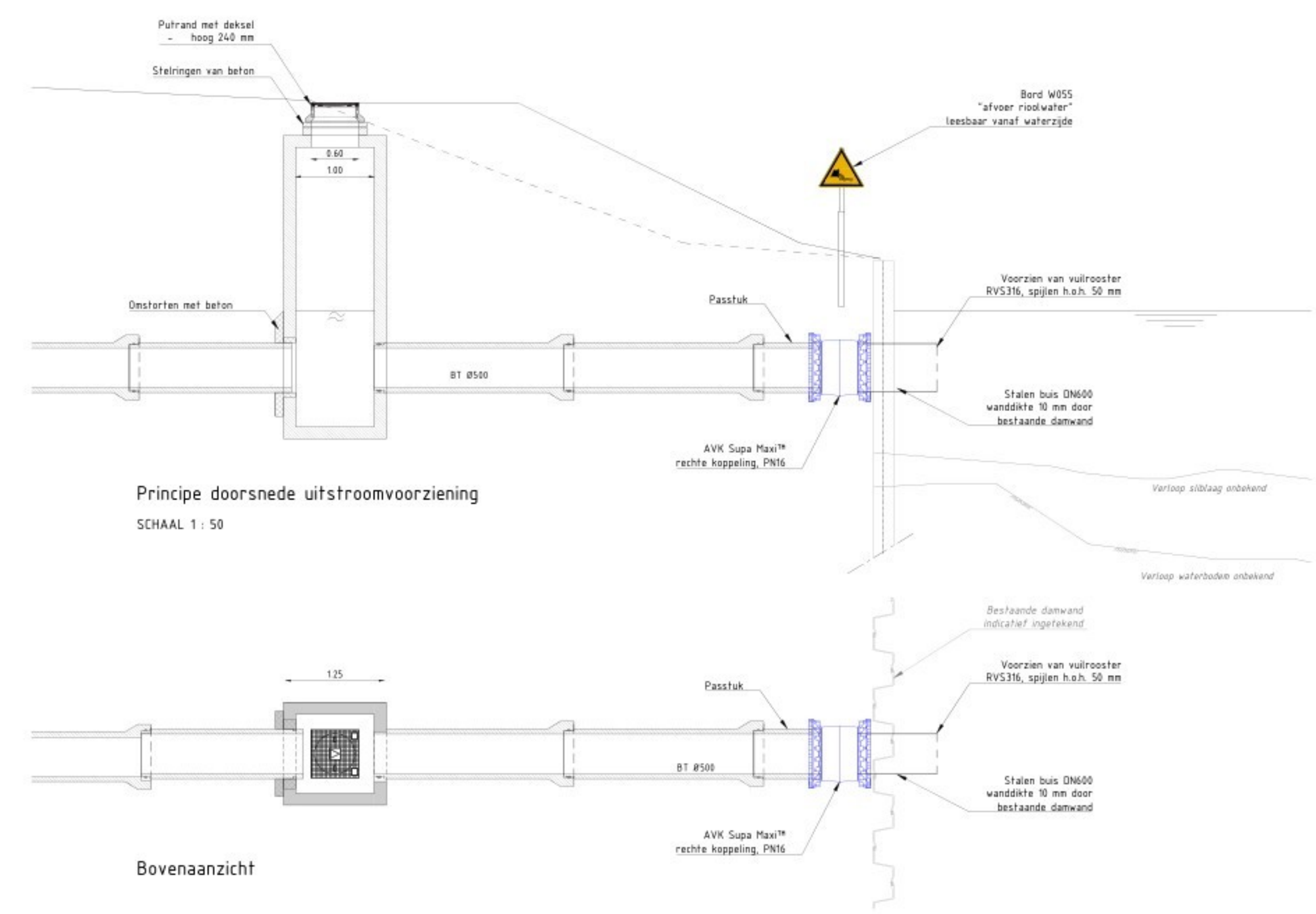
Principe detail kolkaansluiting schaal: 1 : 20
