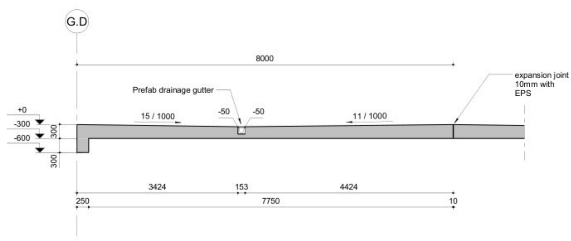
G FB 1 : 50
