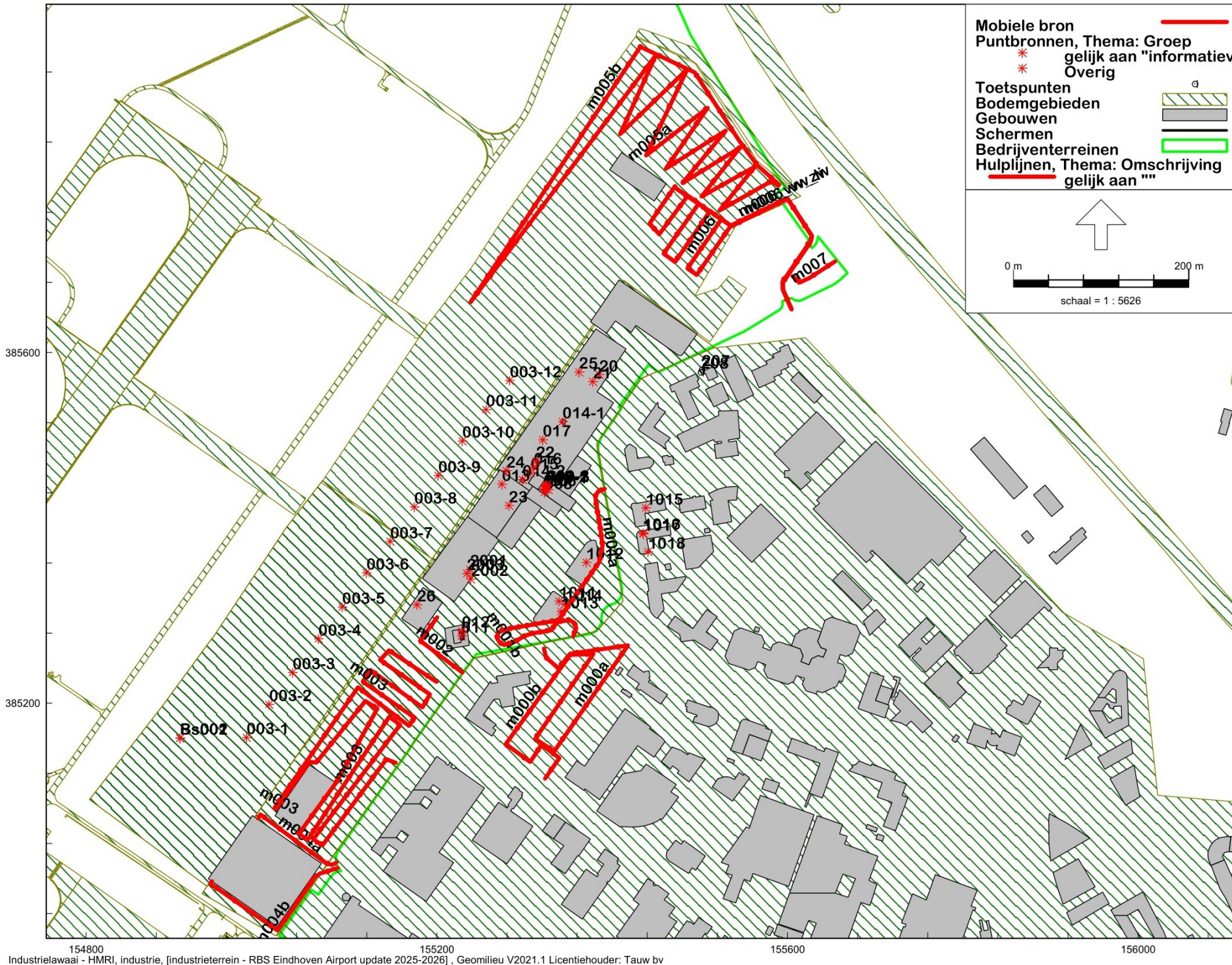
Figuur 1.2 Detail rekemmodel met bronnen Eindhoven Airport
