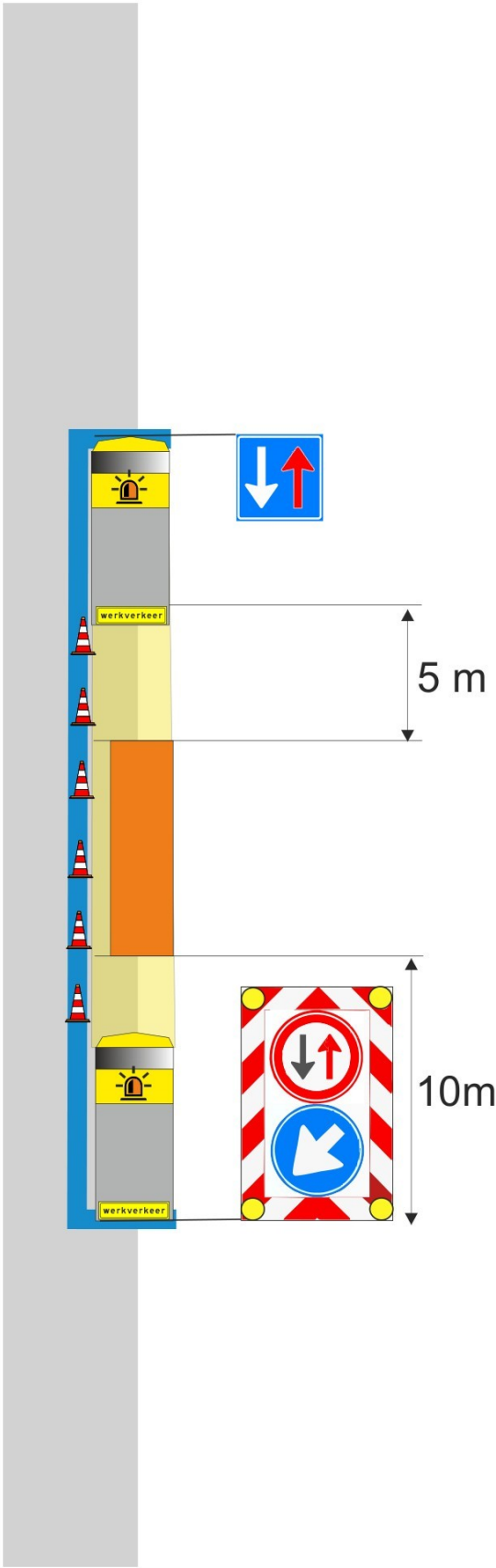
Fig. 96b-1222a: Werken vanaf of op de rijbaan met versmalling van de rijbaan met rijdende afzetting.
