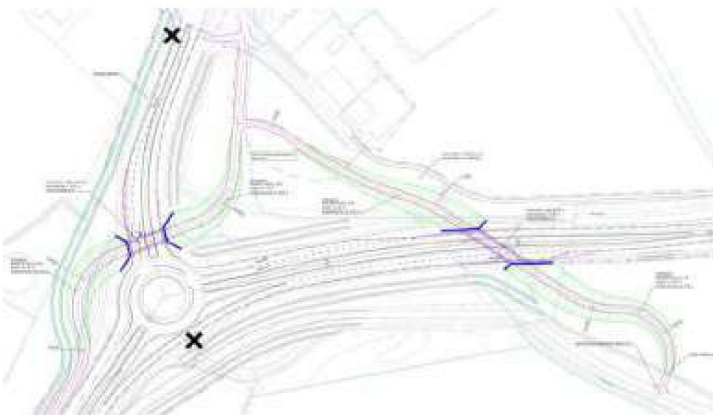
Figuur 3.23 Variant E5 Fietstunnels rotonde West-Om
