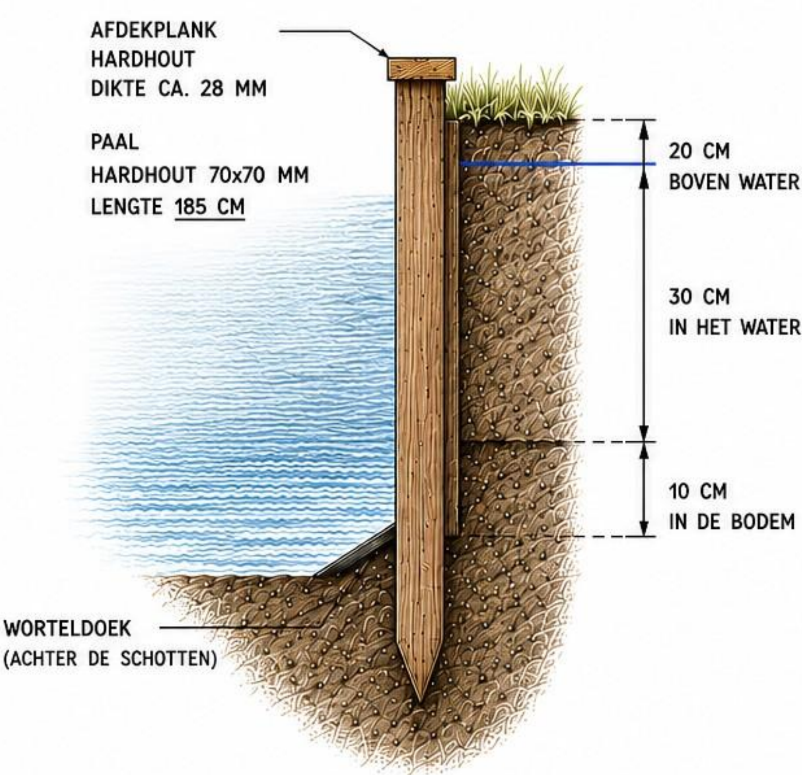
DOORSNEDE
