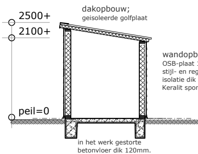
doorsnede
