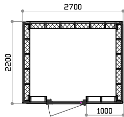
plattegrond
