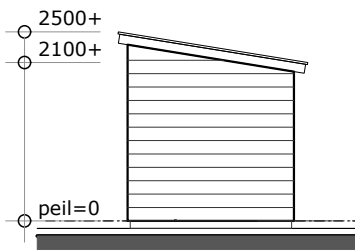
zijgevel
