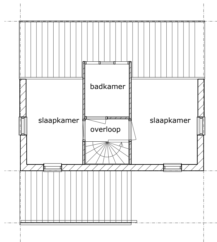
verdieping - gewijzigd
