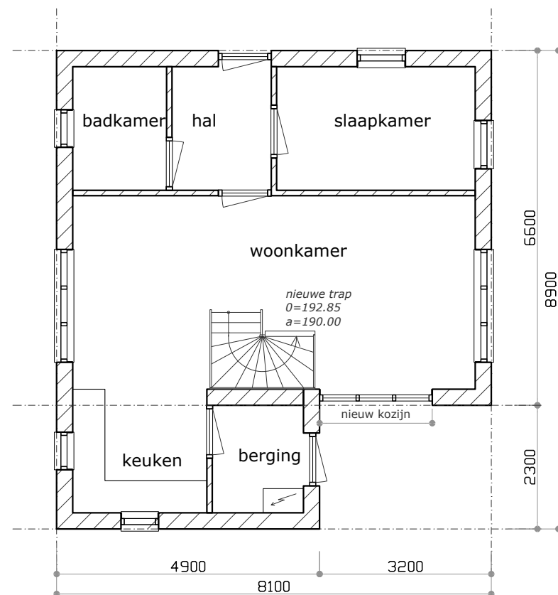
plattegrond - gewijzigd
