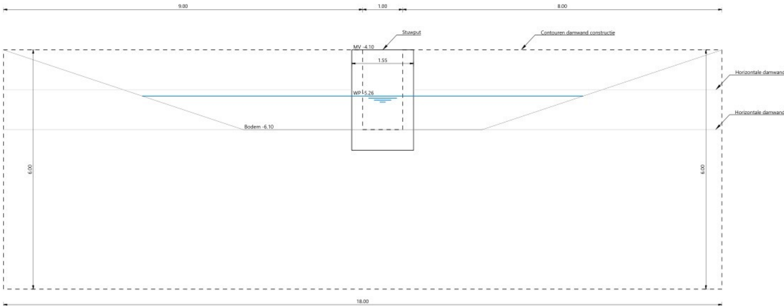
Vooraanzicht stuwput Zwaanplantsoen Schaal 1:50
