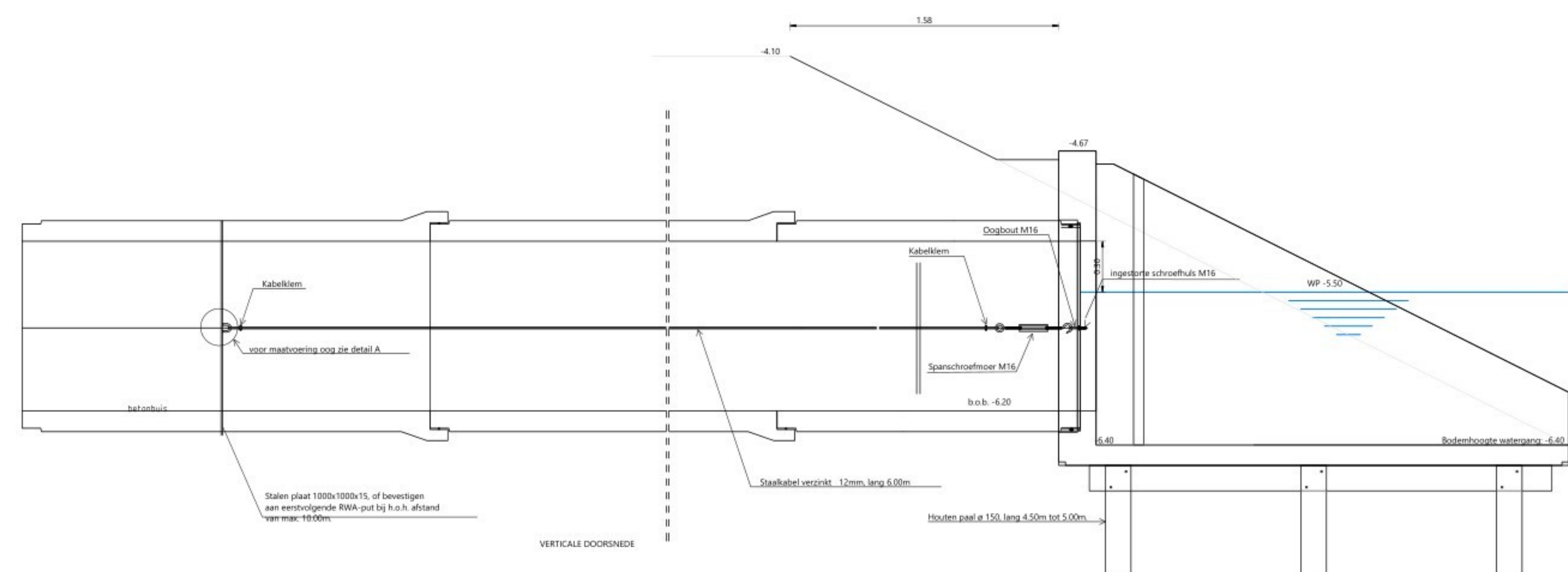
DETAIL UITSTROOMBAK HWA RIOOL BETON Ø1000 Schaal 1:20
