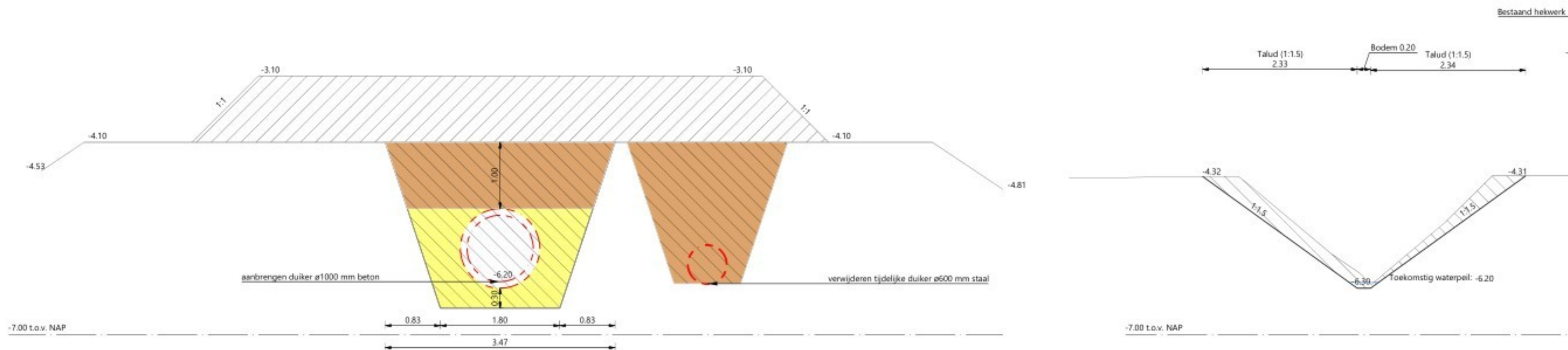
DWARSPROFIEL 6: AANBRENGEN DUIKER Schaal 1:50
