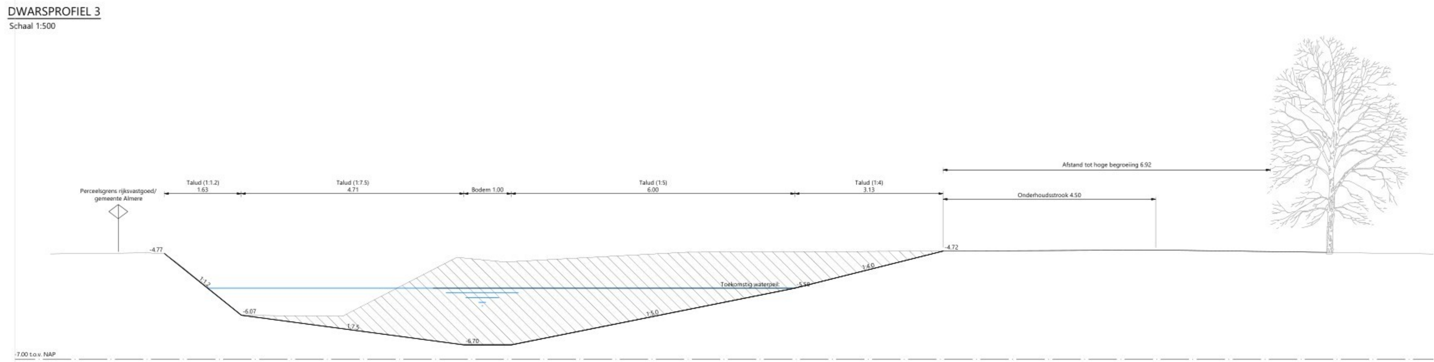
DWARSPROFIEL 4 Schaal 1:500
