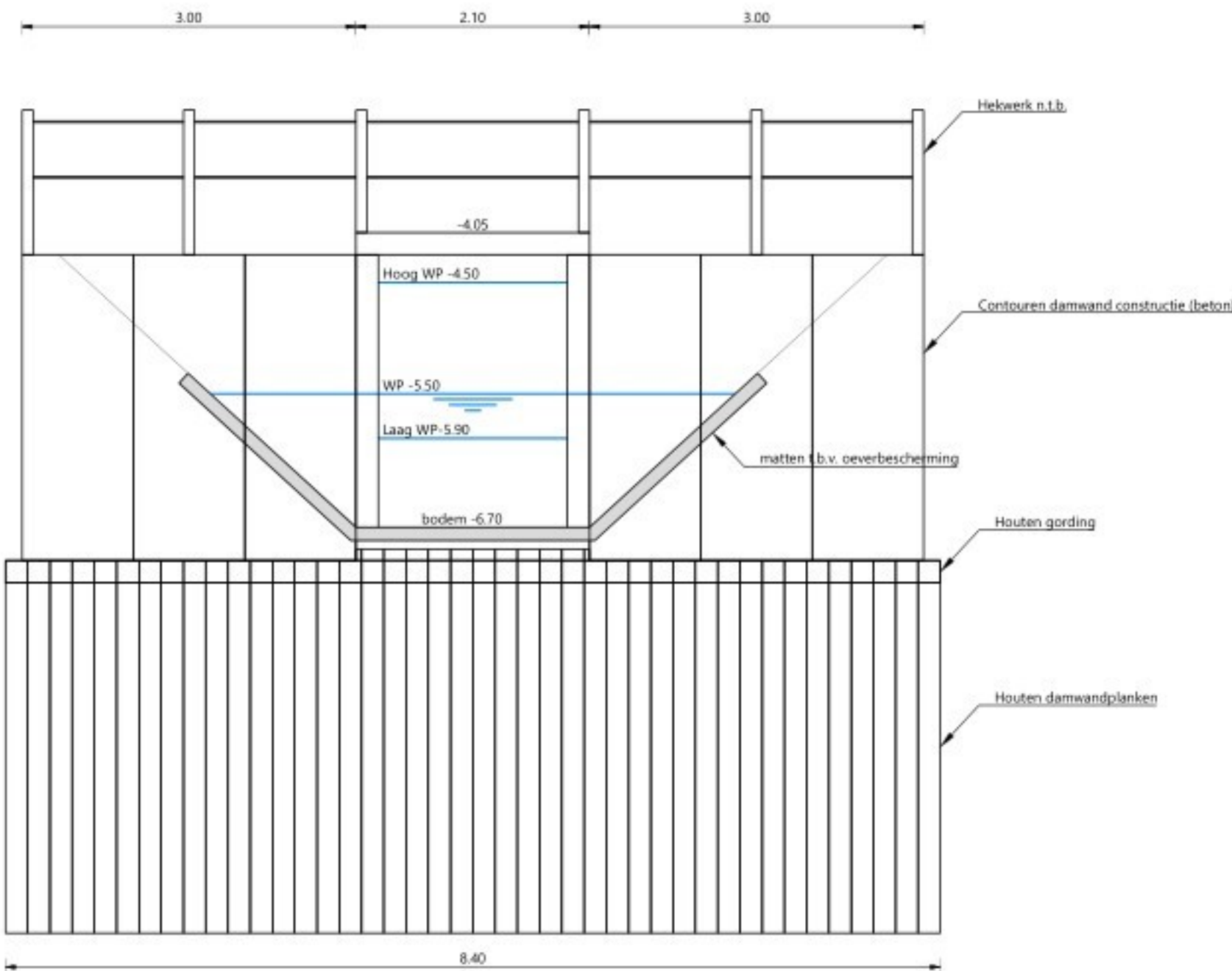
Vooraanzicht stuwput Watersnipweg Schaal 1:50
