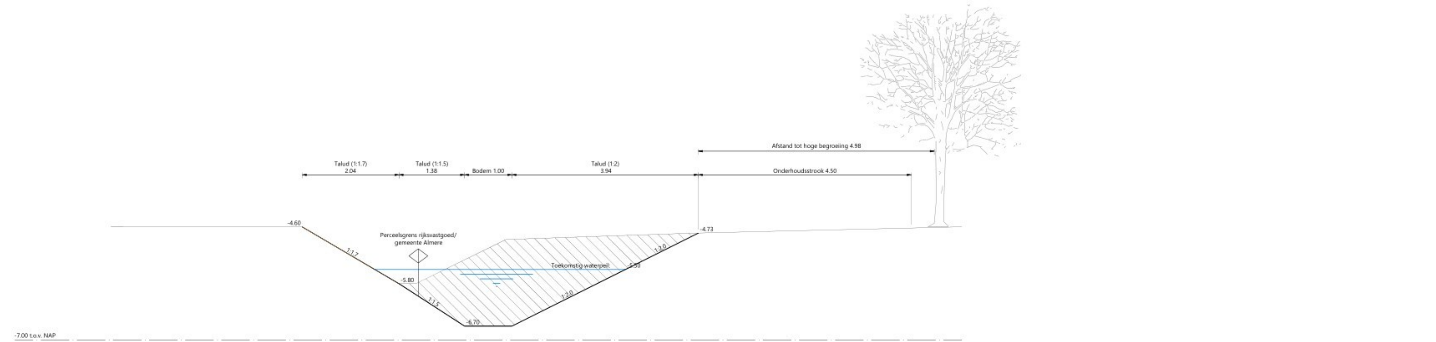
DWARSPROFIEL 1 Schaal 1:500
