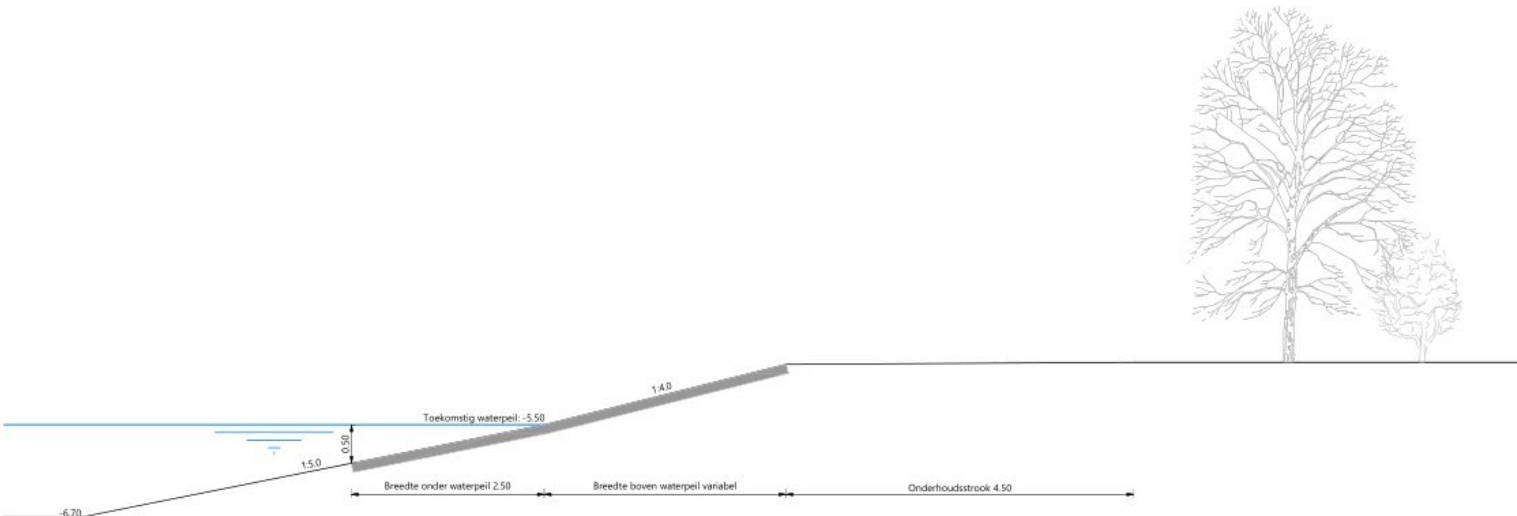
Principeprofiel te water laat plaats maaiboten Schaal 1:50
