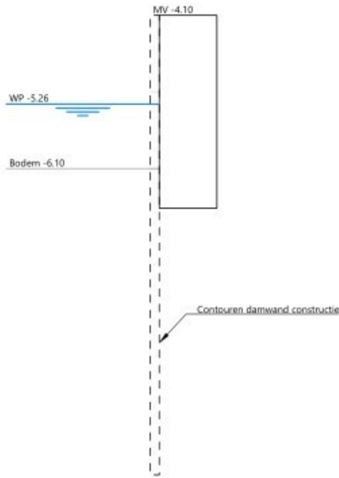
Zijaanzicht stuwput Zwaanplantsoen Schaal 1:50
