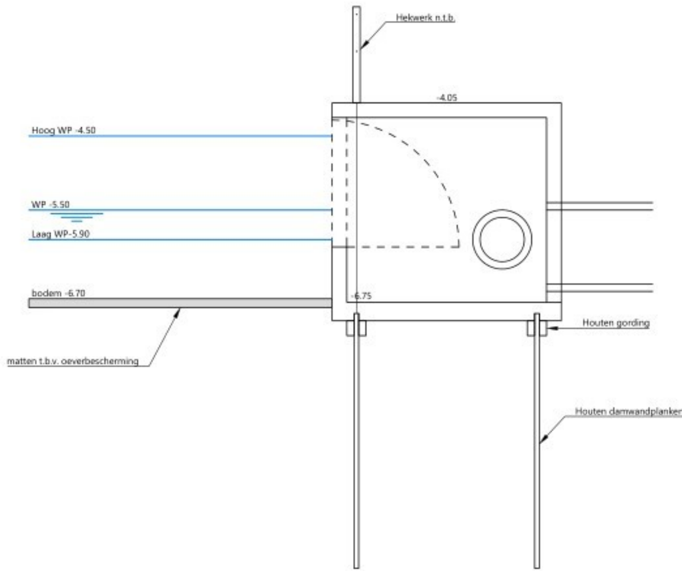
Zijaanzicht stuwput Watersnipweg Schaal 1:50
