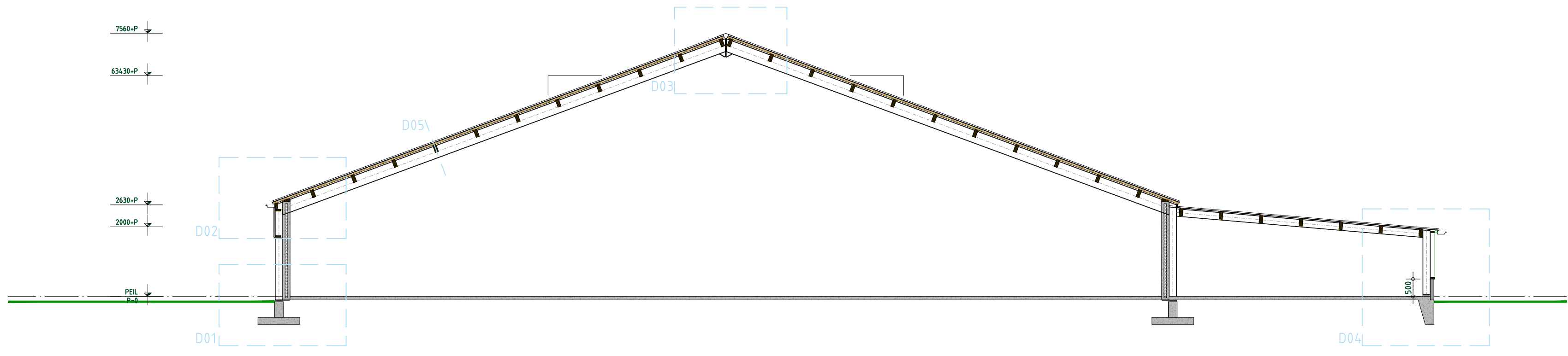
DOORSNEDE AA
