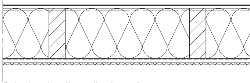
Principedetail verdiepingsvloer schaal: 1:10
