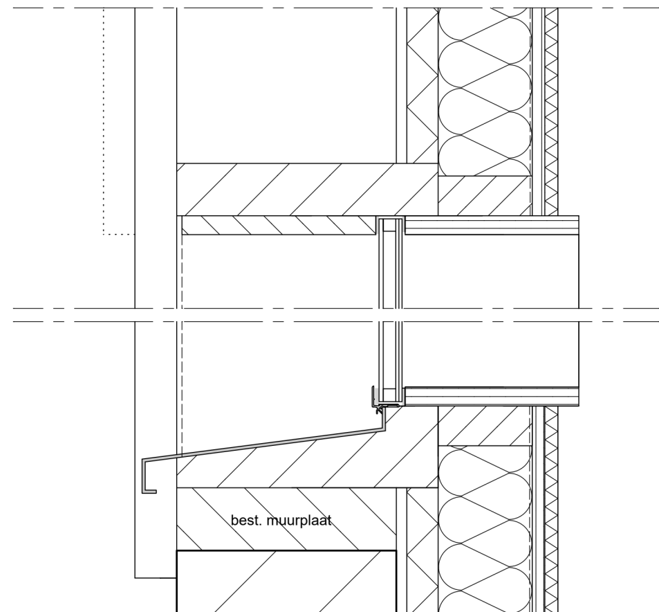
Principedetail lichtstroken schaal: 1:5
