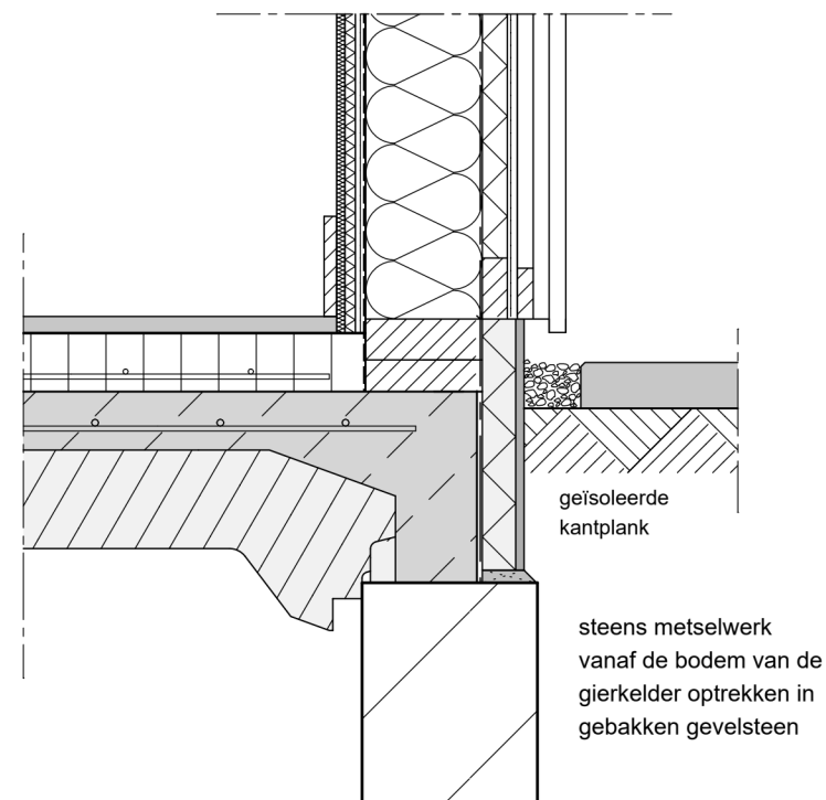
Principedetail 3: hsb-gevels bij entree PS-isolatievloer schaal: 1:10
