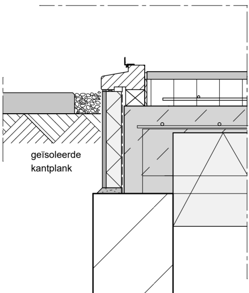
Principedetail 4: t.p.v. glaspui PS-isolatievloer schaal: 1:10
