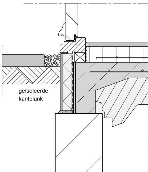
Principedetail 5: entreedeur PS-isolatievloer schaal: 1:10
