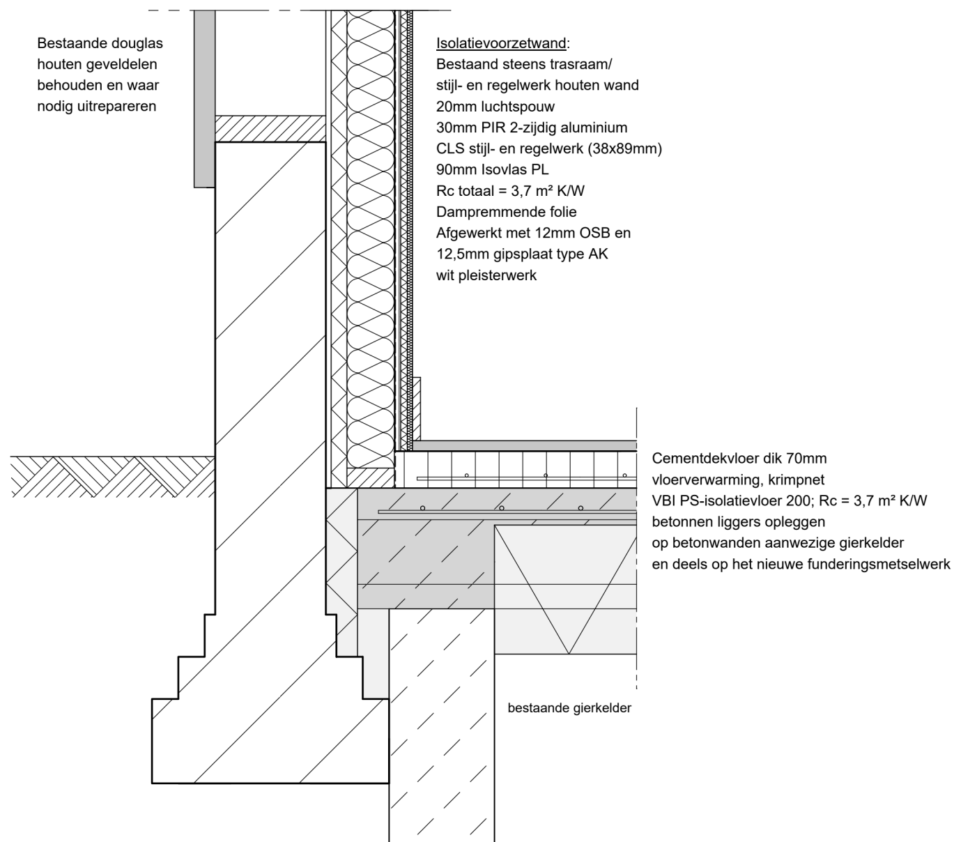
Principedetail 1: isolatievoorzetwand bestaande houten buitengevels bestaand trasraam en girkelder PS-isolatievloer schaal: 1:10
