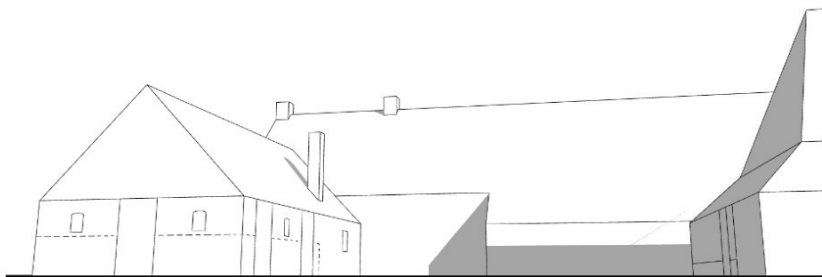
Afb. 33: De waarschijnlijke oorspronkelijke vorm van het kookhuis annex varkenshuis in Sketch-Up® vanuit het zuidwesten.
