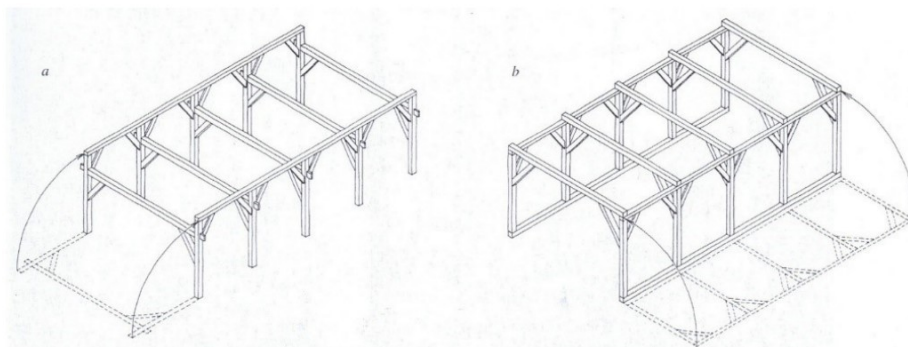
Afb. 13: Gebintconstructies in boerderijen. Links dwarsgebinten (a) en rechts langsgebinten (b).
