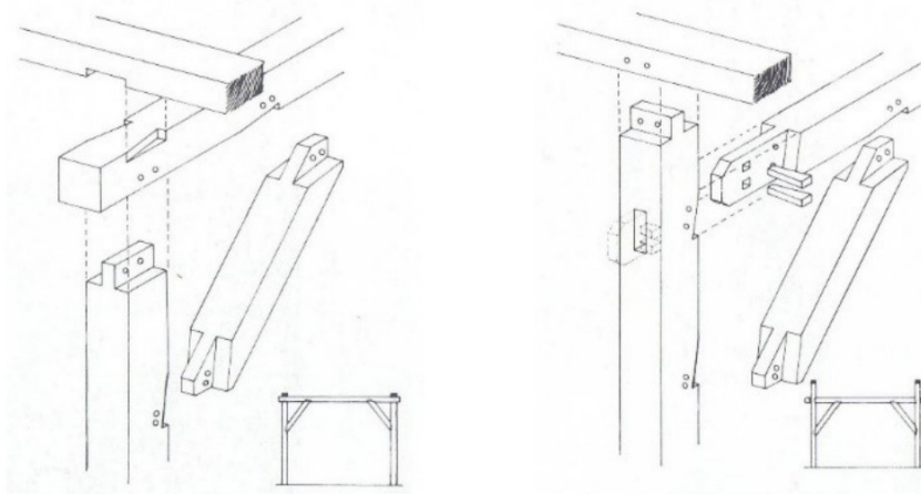
Afb. 15: Verbindingen van gebintconstructies. Links het dekbalkgebint en rechts het ankerbalkgebint.
