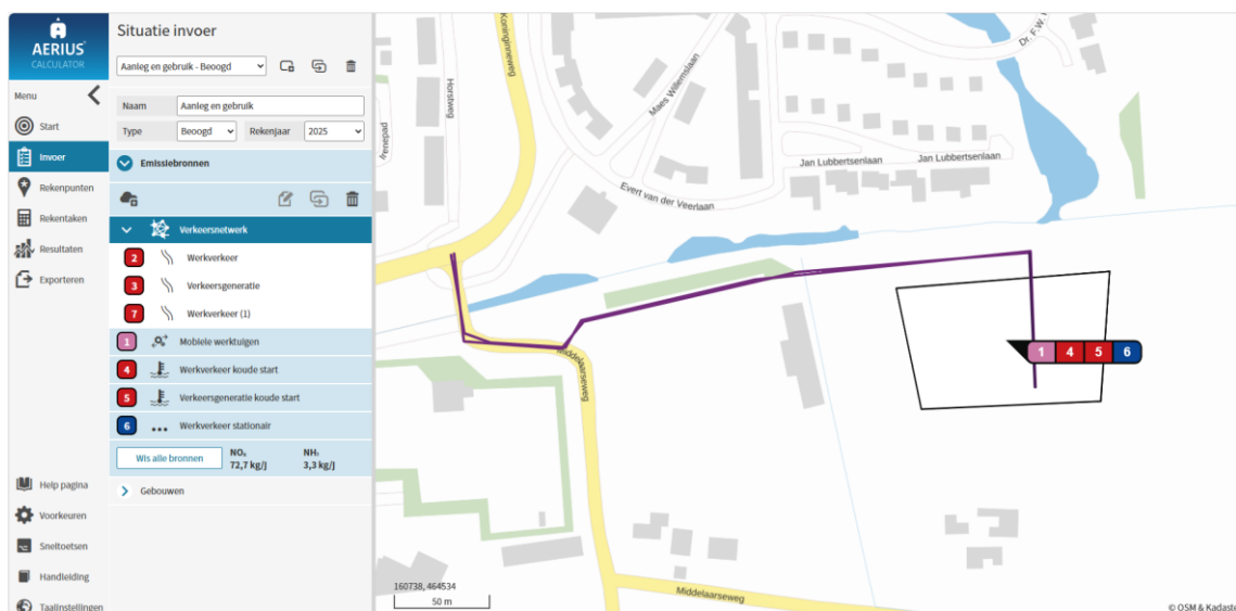
Afbeelding 3 - AERIUS-model
