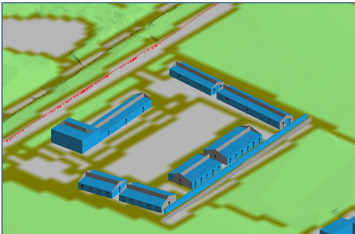
Afbeelding 6. Rekenmodel, 3d-weergave (detail)
