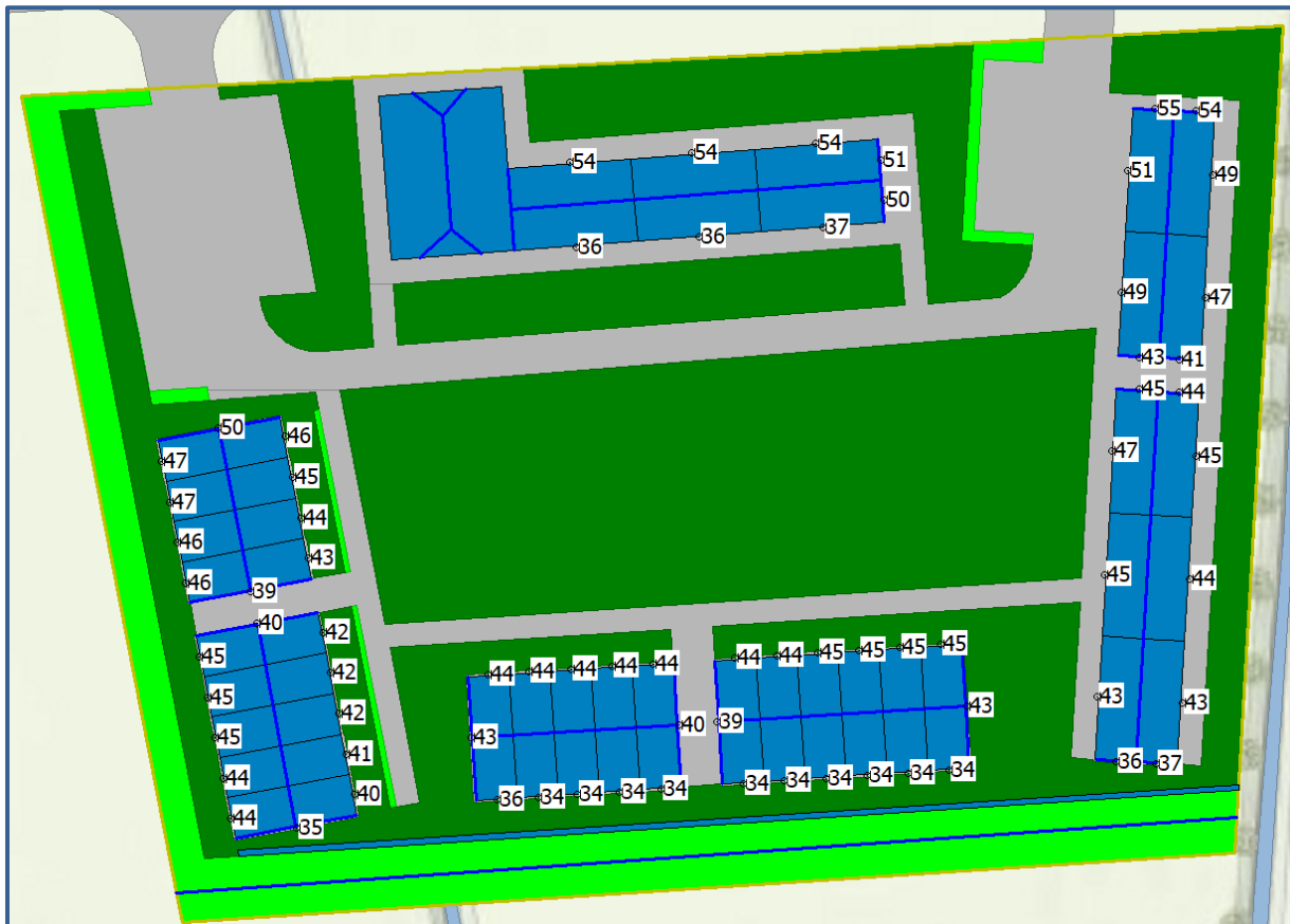
Afbeelding 8. Geluid L_{den} Gemeentewegen Berekend geluid op een hoogte van 1,8 meter
