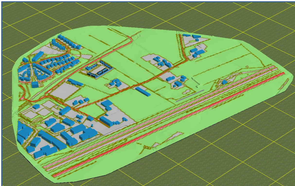
Afbeelding 5. Rekenmodel, 3d-weergave (overzicht)
