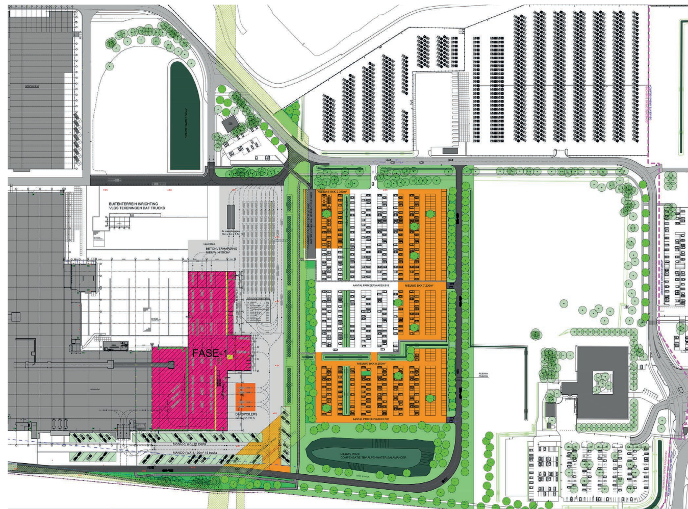
Afbeelding 1.4 nieuwe situatie uitbreiding truckfabriek en parkeerplaats d.d. 12 januari 2026
