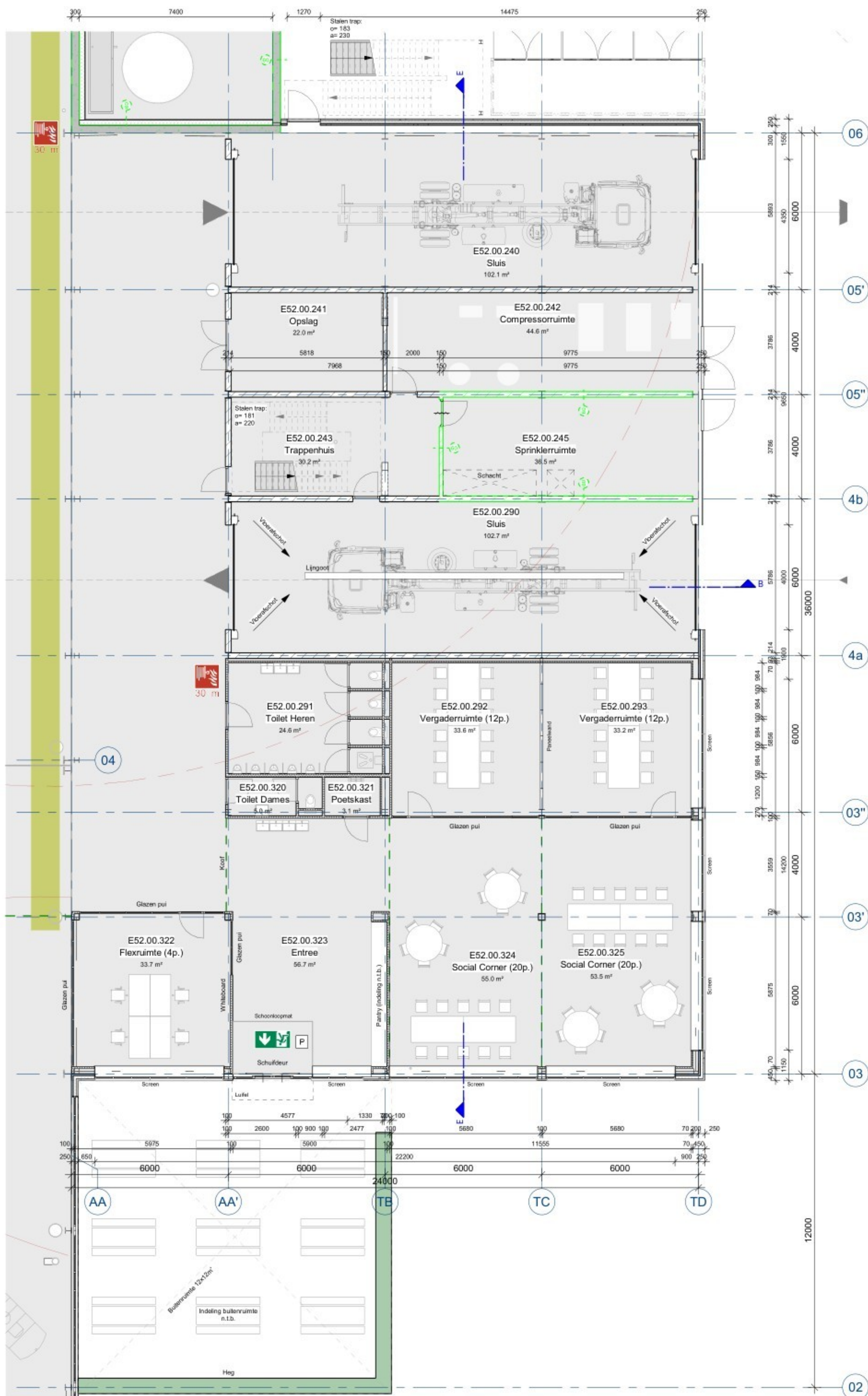
BEGANEGROUND TECHNIEKRUIMTE
