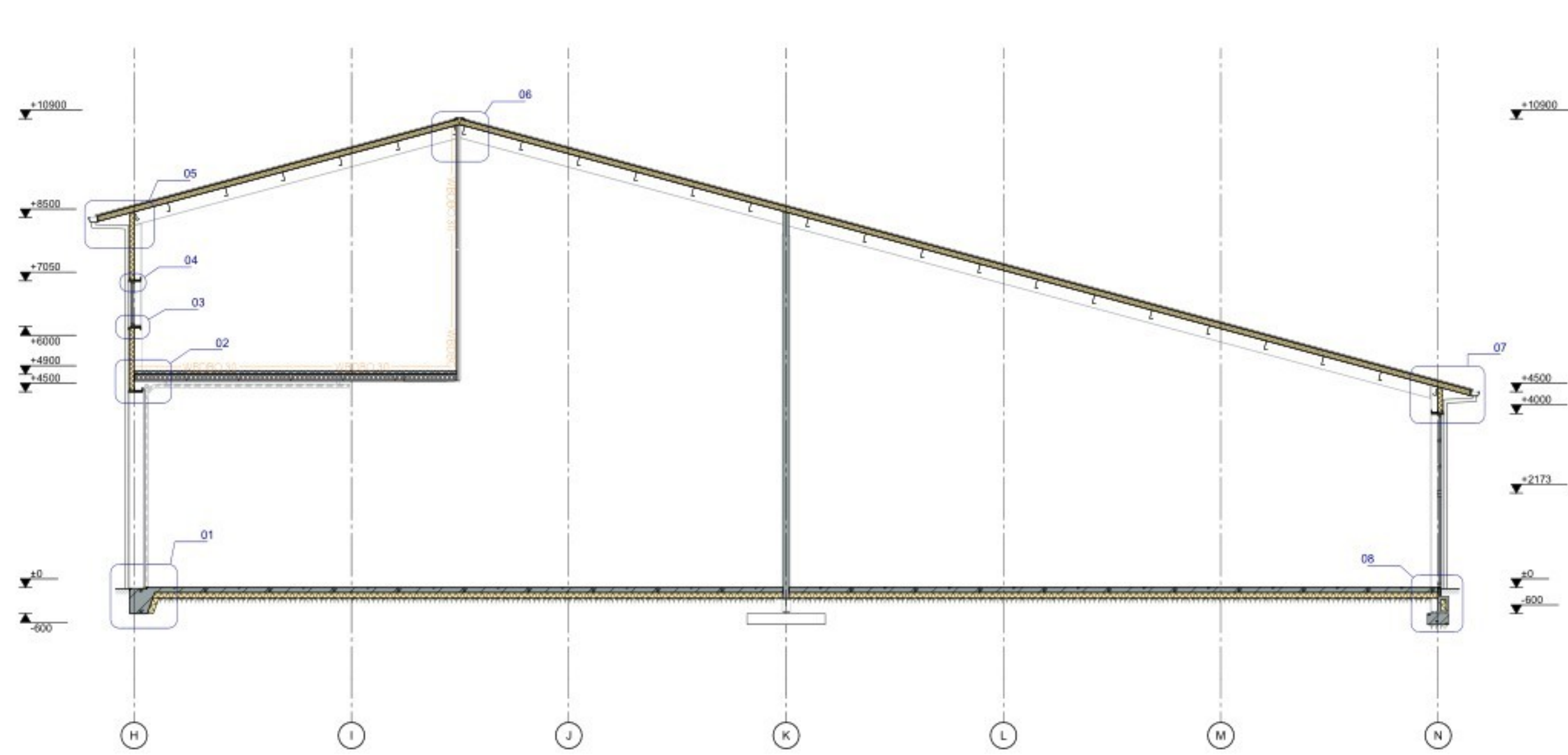
Doorsnede A
