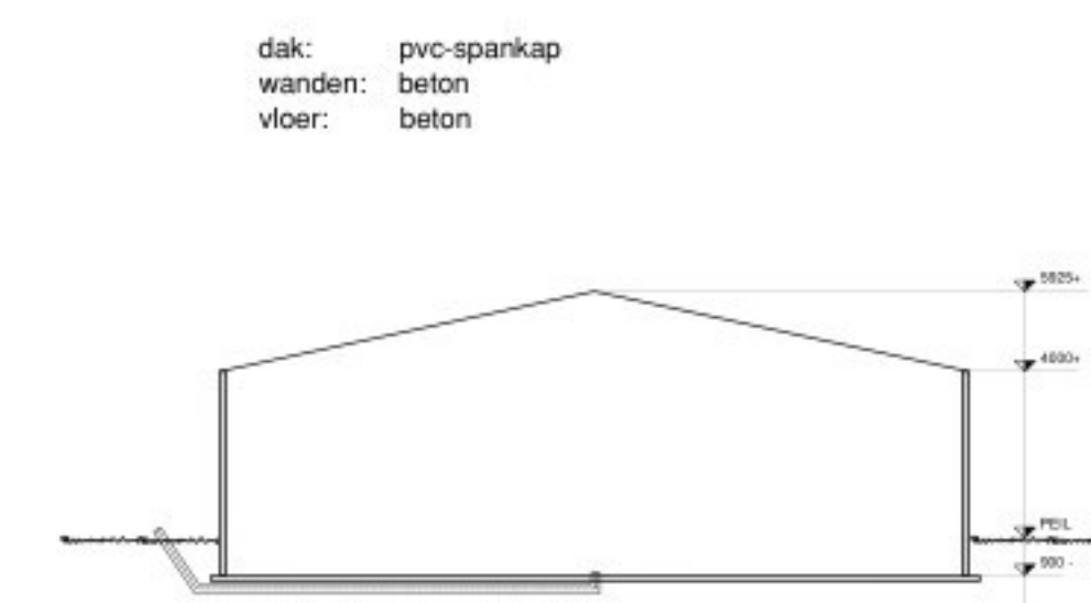
DOORSNEDE H - H
