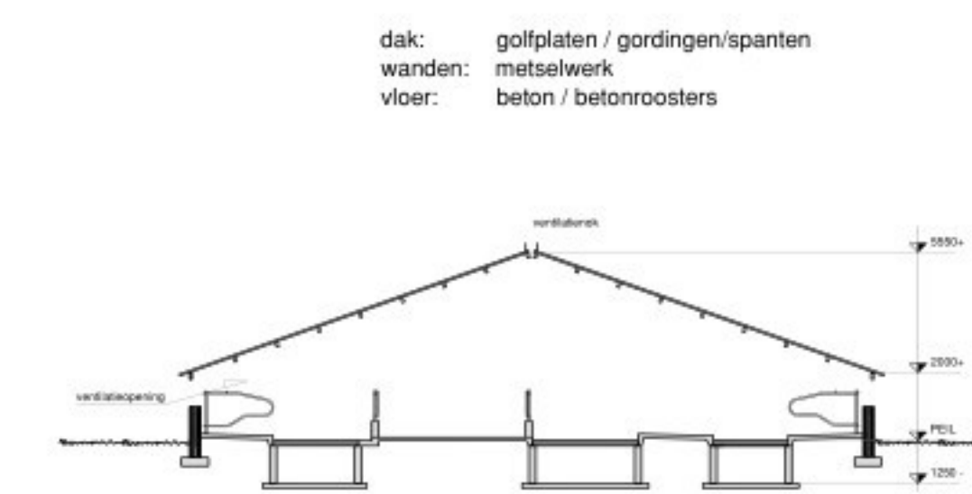
— DOORSNEDE F - F
