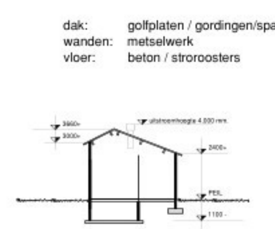
DOORSNEDE E - E
