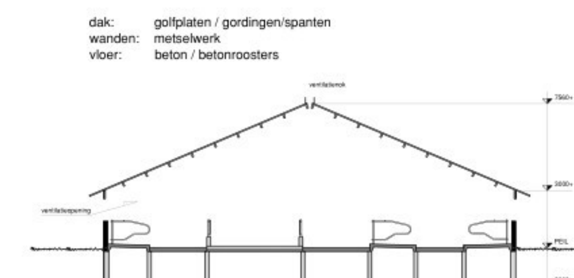
— DOORSNEDE G - G
