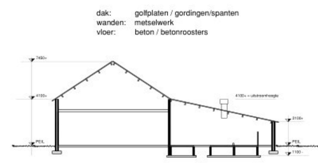
DOORSNEDE B - B
