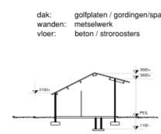
DOORSNEDE D - D
