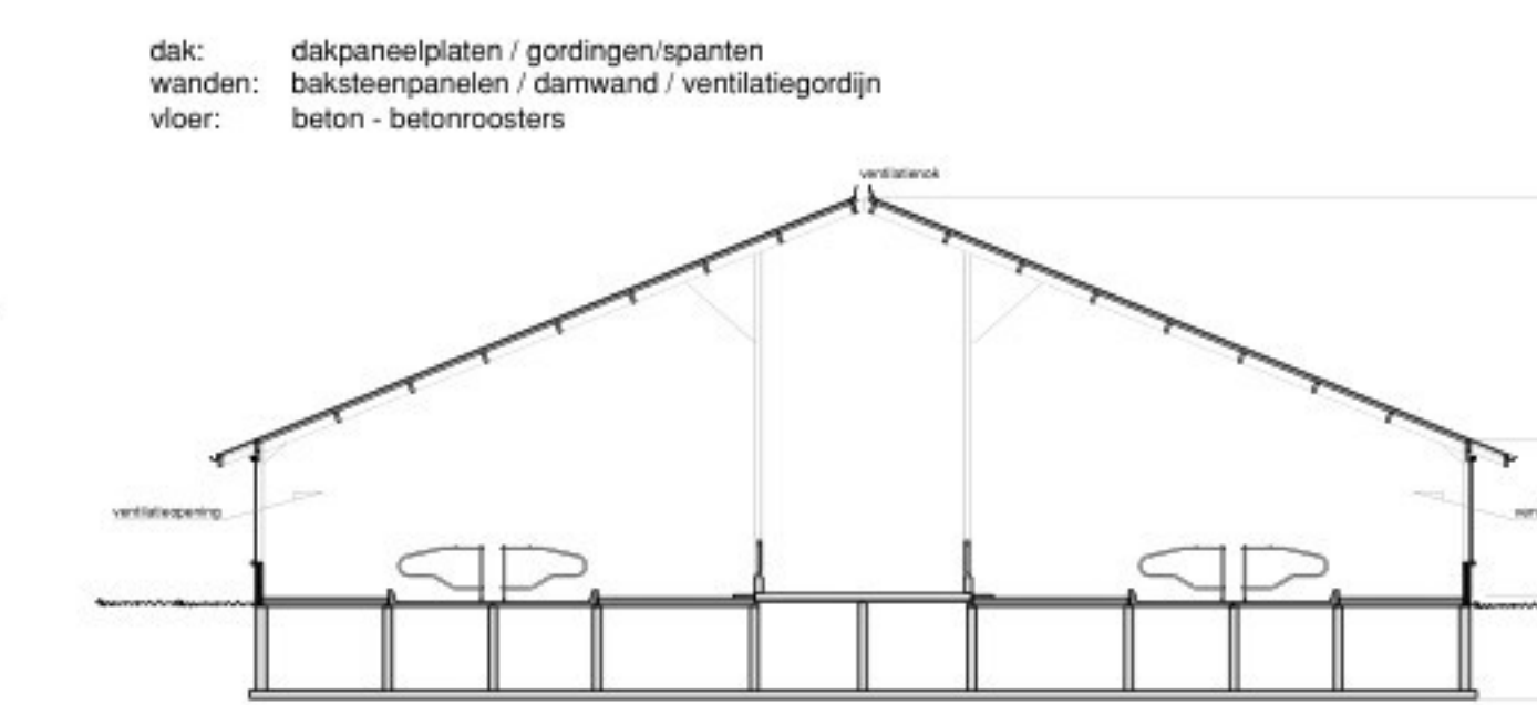
DOORSNEDE K - K
