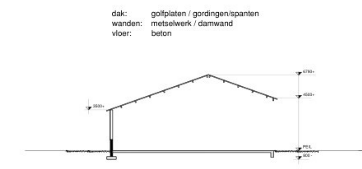
DOORSNEDE J - J
