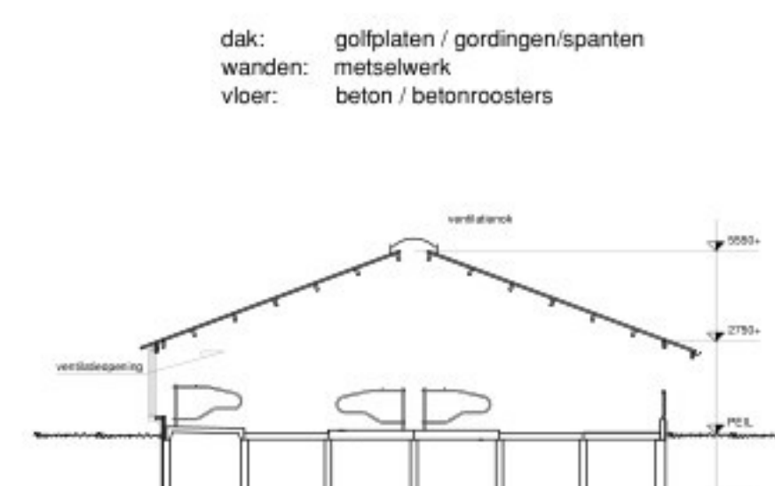
DOORSNEDE C - C
