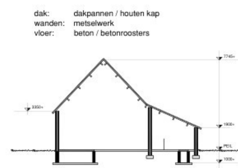
DOORSNEDE A-A
