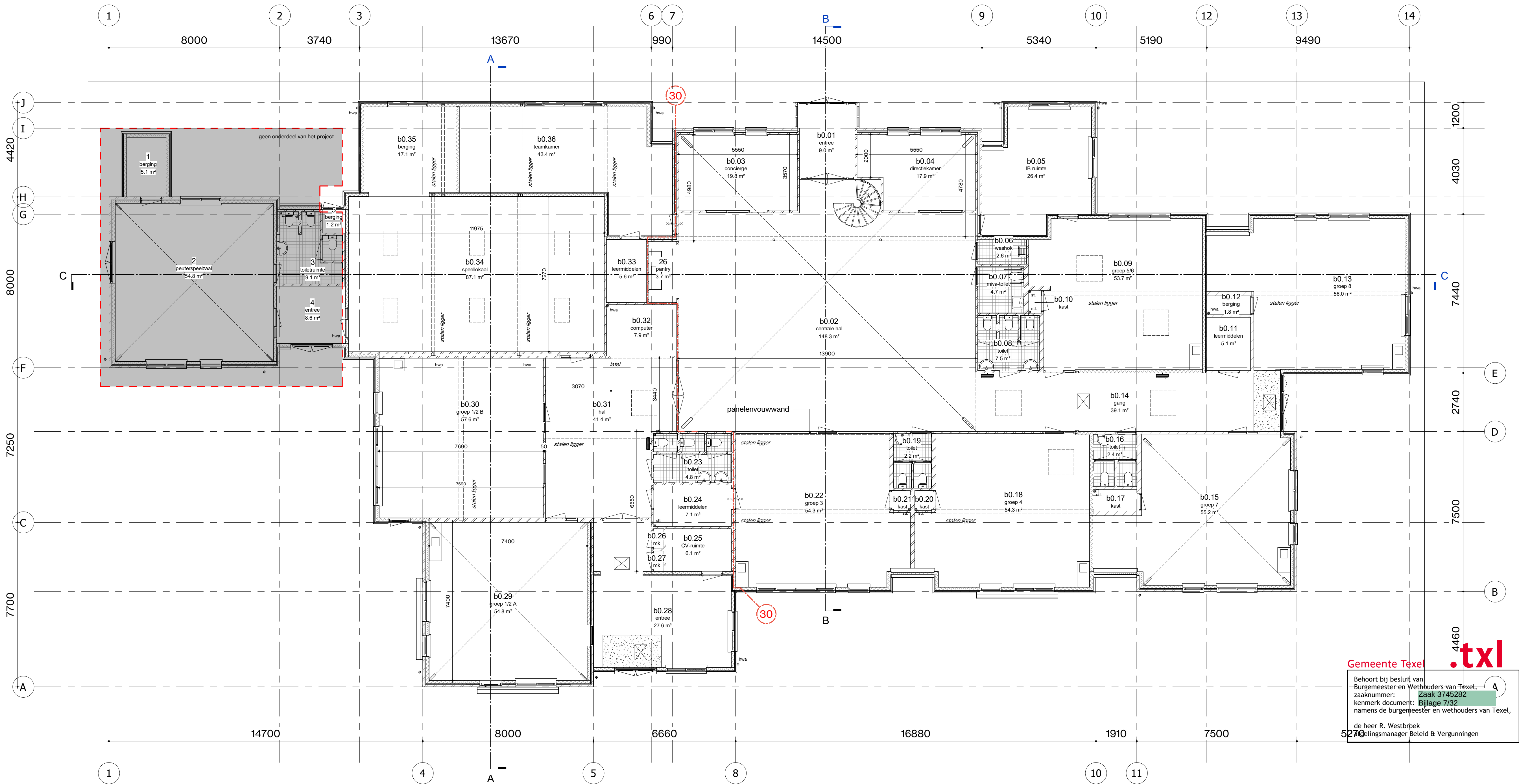
Begane grond
