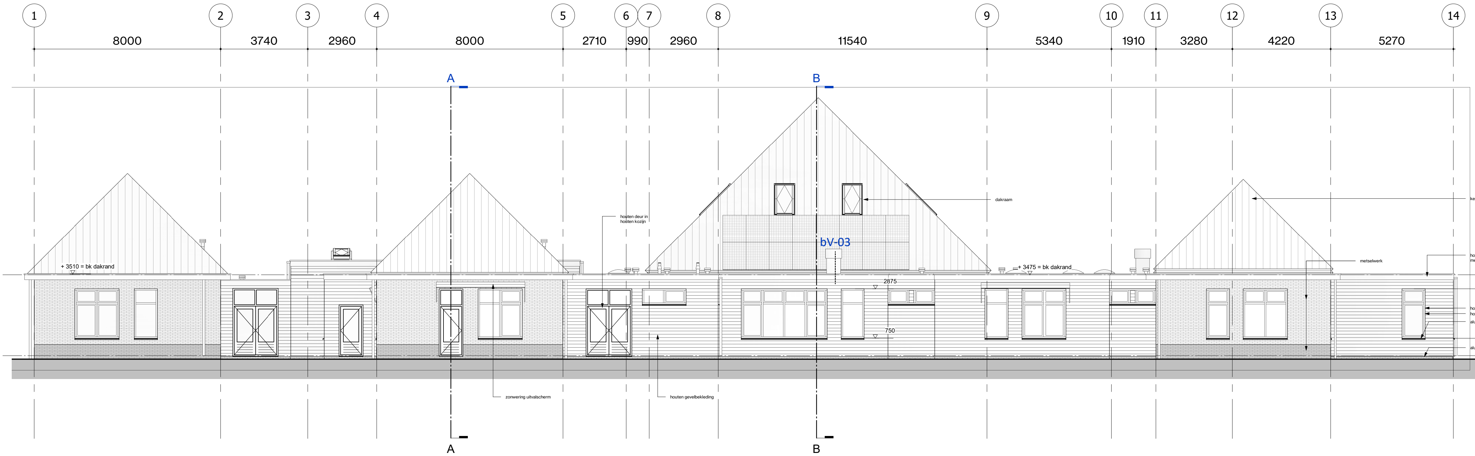
Vooraanzicht - Oostgevel
