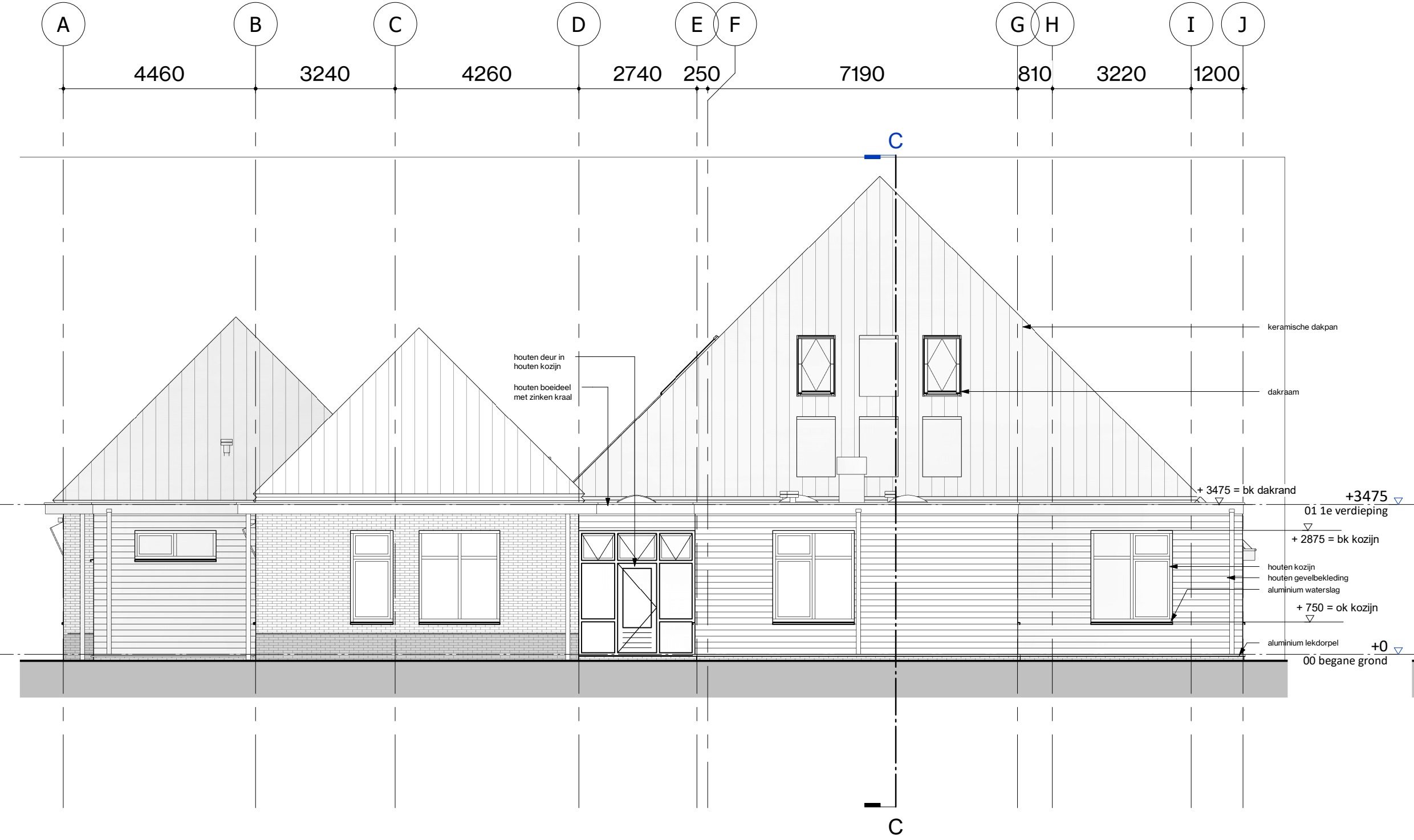
Rechterzij aanzicht - Noordgevel
