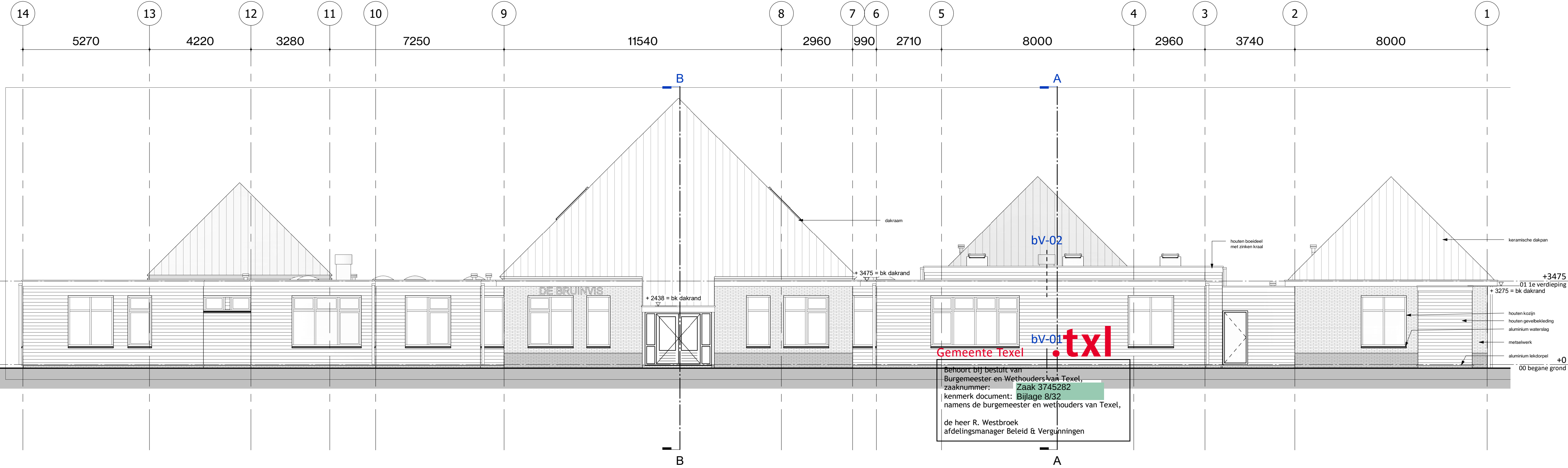
Achterzij aanzicht - Westgevel
