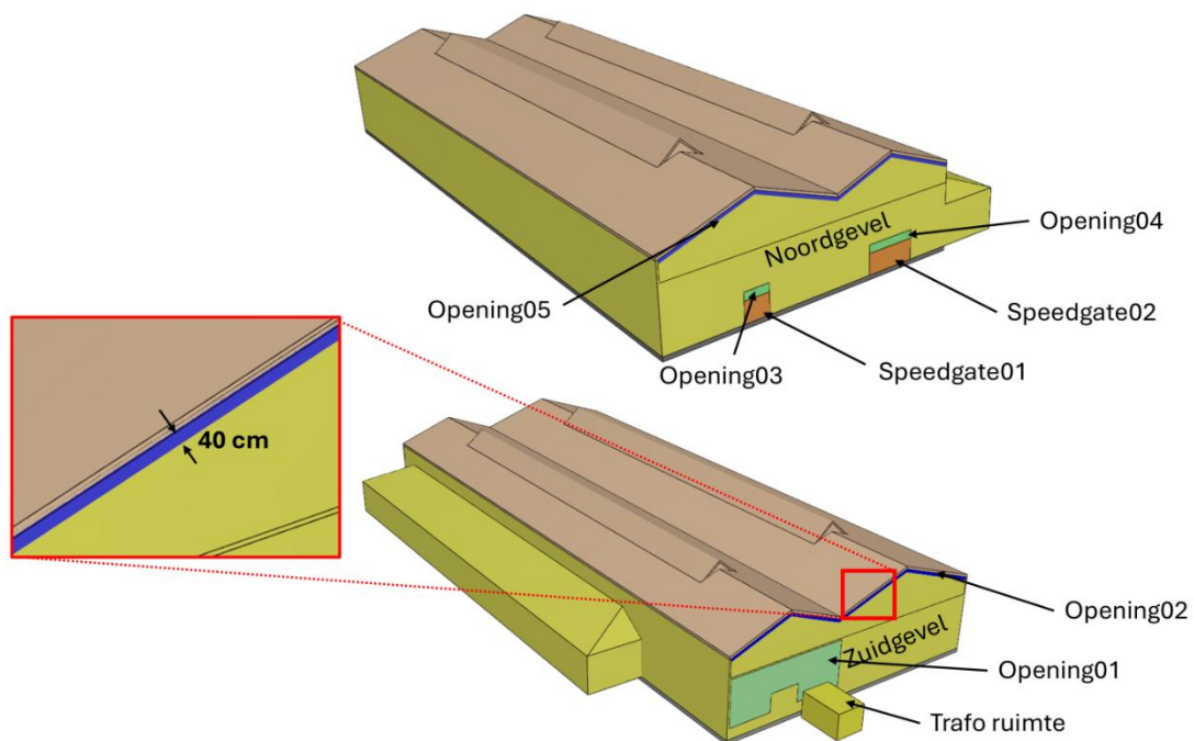
Figuur 14: Overzicht van de locaties voor optie 2 waar het ventilatiedebiet in en uit de garage is gemeten.
