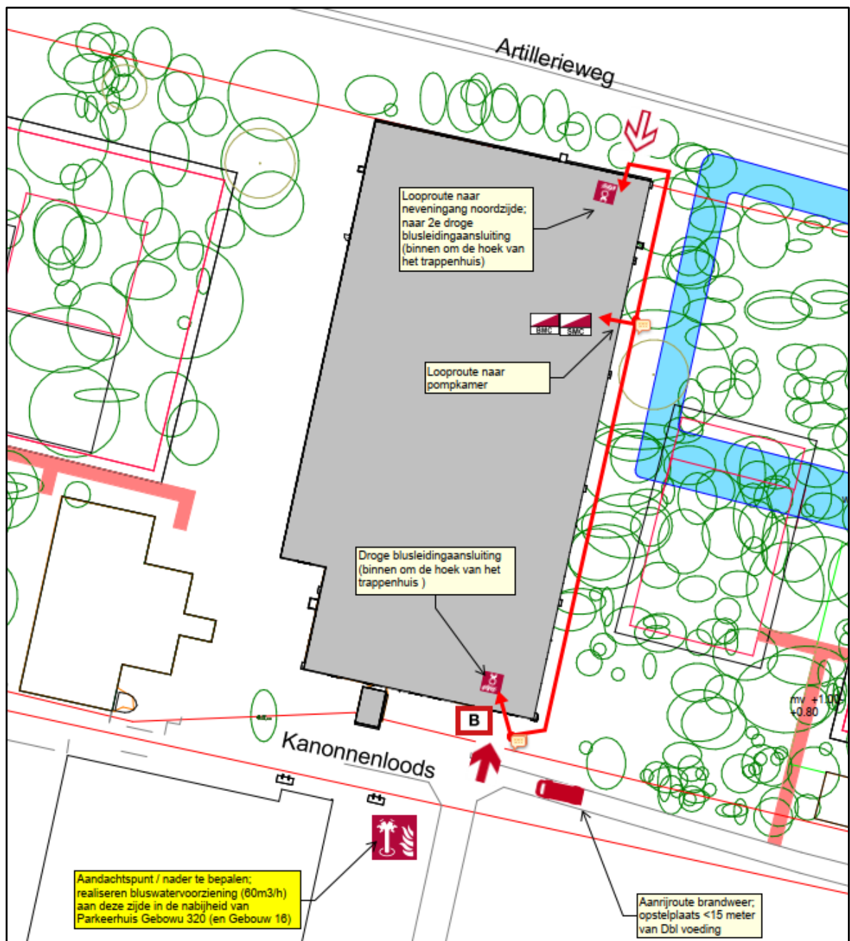
Figuur 3: Situatie brandweerinzet
