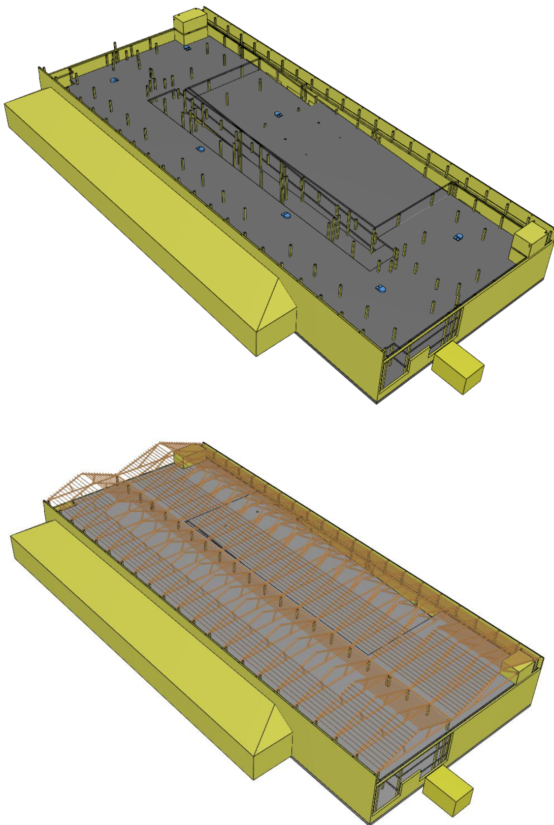
Figuur 4: Weergave van het 3D CFD-model; in het bovenste figuur is de verdiepingsvloer van laag 3 verborgen om laag 2 te laten zien, in het onderste figuur worden alle vloeren getoond.
