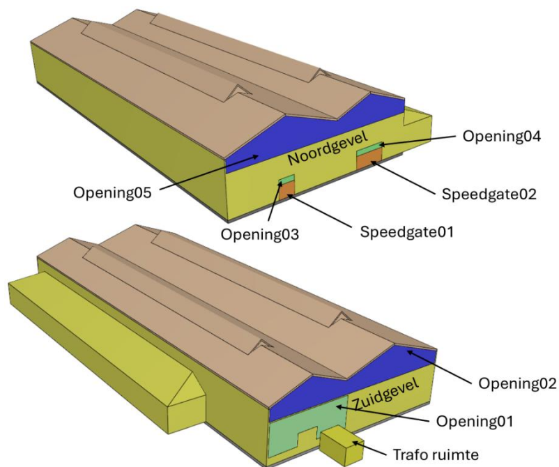
Figuur 5: Overzicht van de locaties voor optie 1 waar het ventilatiedebiet in en uit de garage is gemeten.
