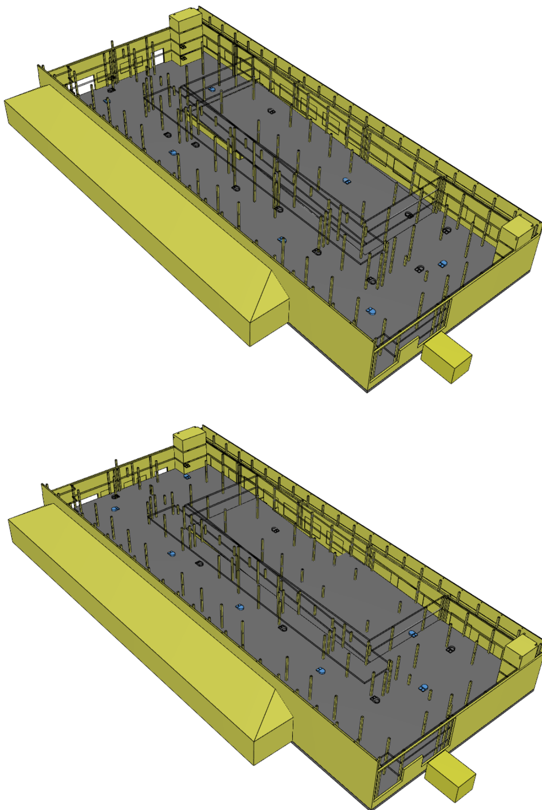
Figuur 3: Weergave van het 3D CFD-model; in het bovenste figuur zijn de verdiepingsvloeren van lagen 1, 2 en 3 verborgen om de Begane grond te laten zien, in het onderste figuur wordt de 1 e verdieping getoond.
