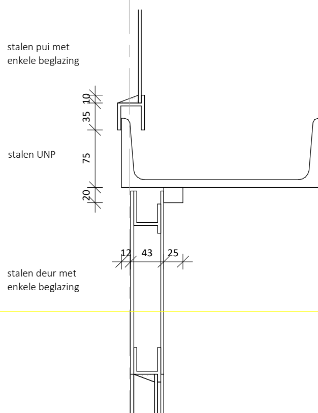
BT_DE_04A 1 : 5 - bestaand
