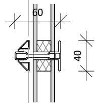
OV_DE_04A 1 : 5 - nieuw
