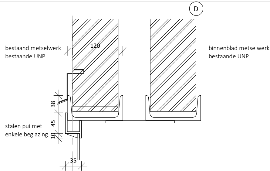
BT_DE_04 1 : 5 - bestaand
