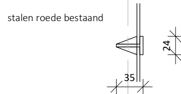
BT_DE_04A 1 : 5 - bestaand
