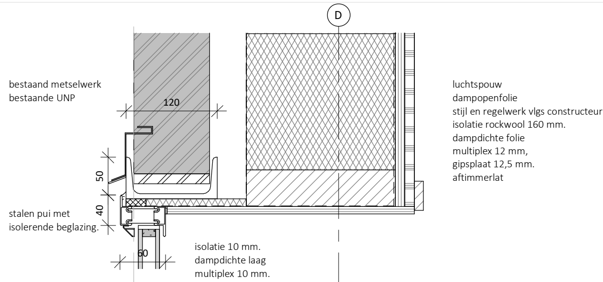
OV_DE-04 1 : 5 - nieuw
