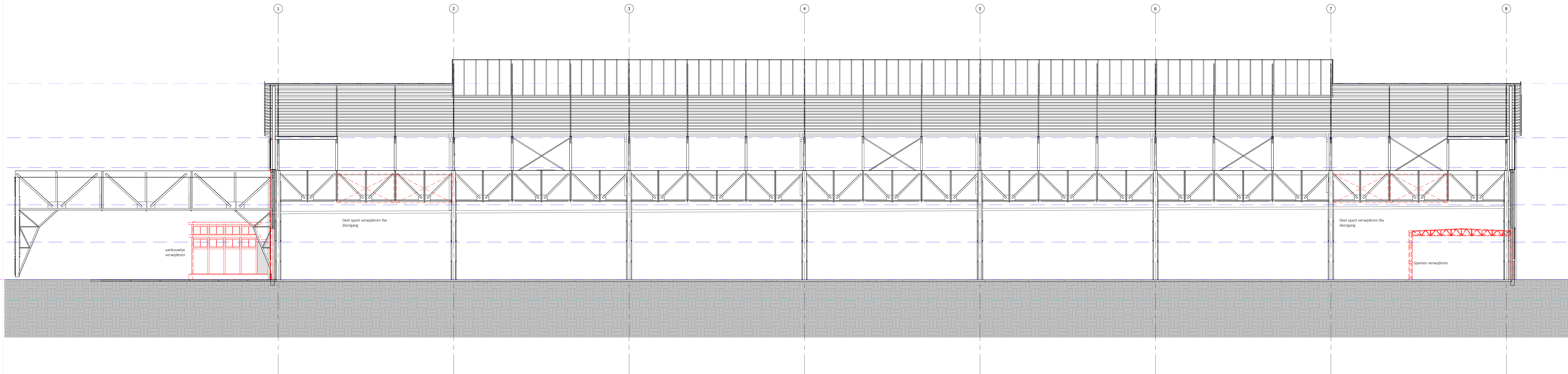
Doorsnede A-A 1 : 100 - nieuw
