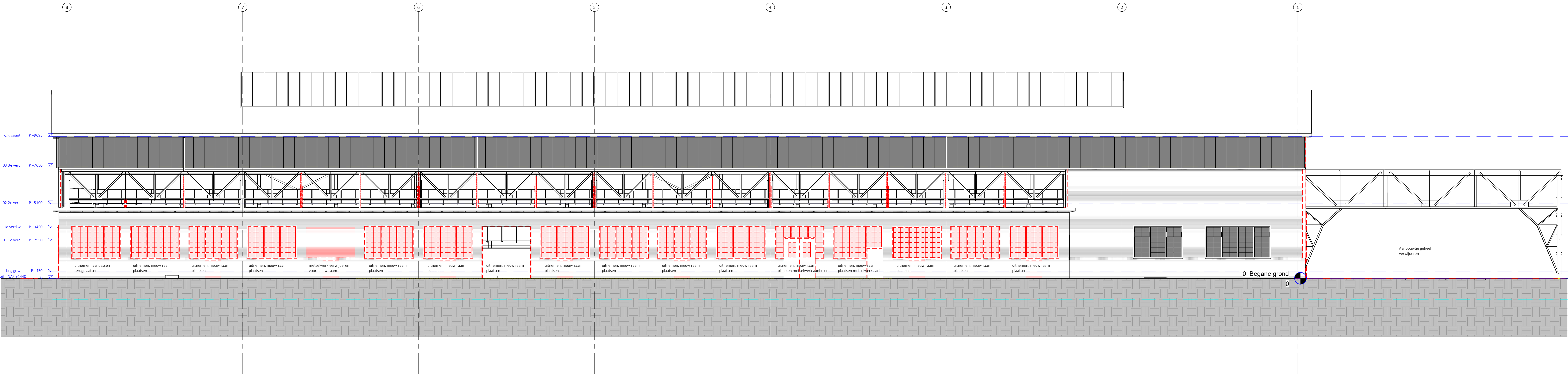
OV-SL_westgevel 1:100 - nieuw
