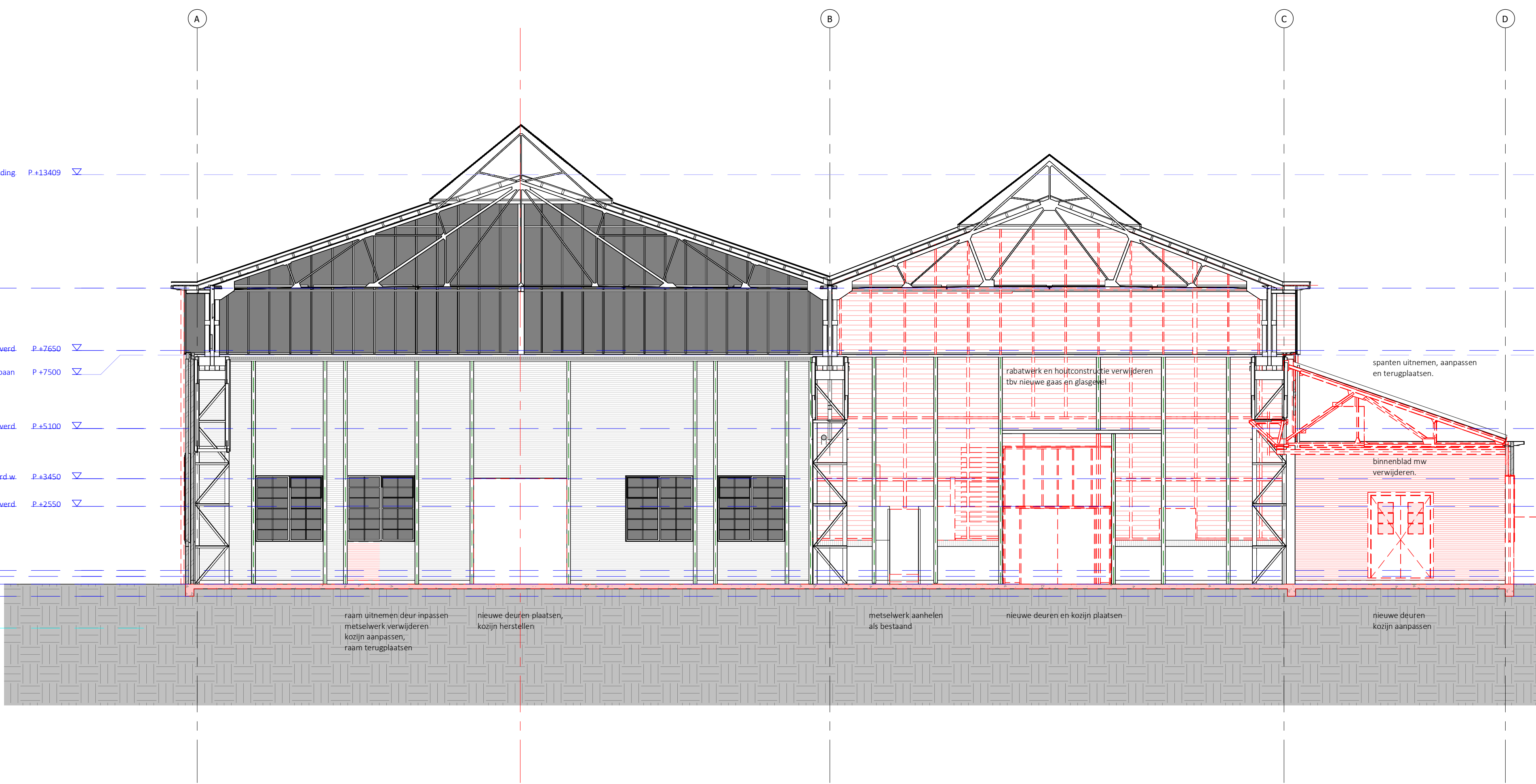
Doorsnede D-D 1 : 100 - nieuw
