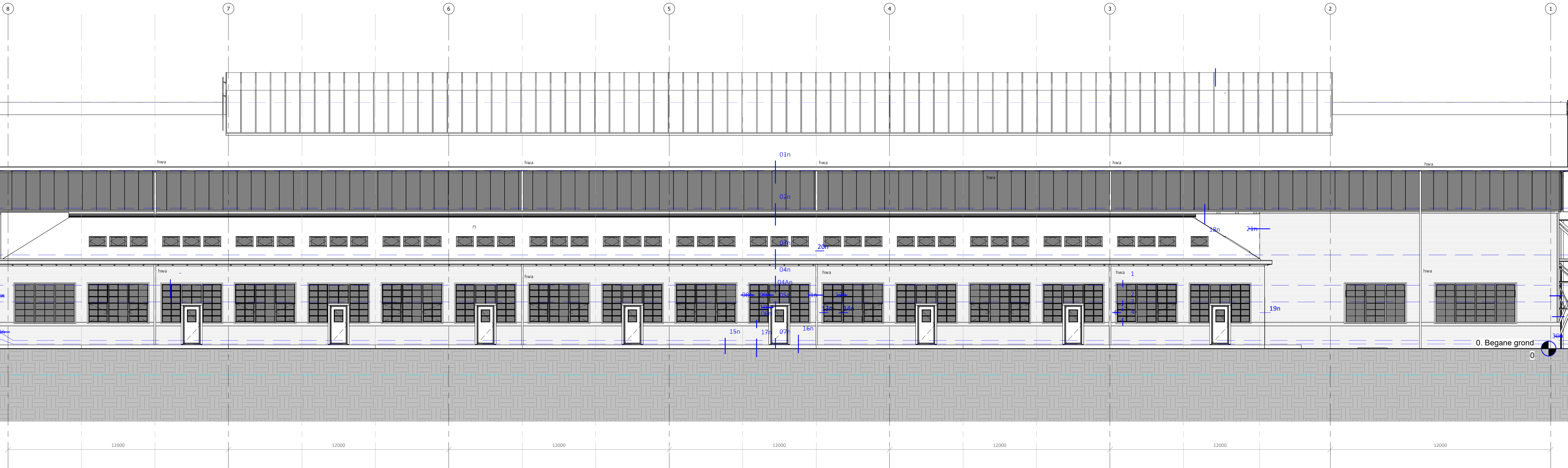
Westgevel 1 : 100 - nieuw
