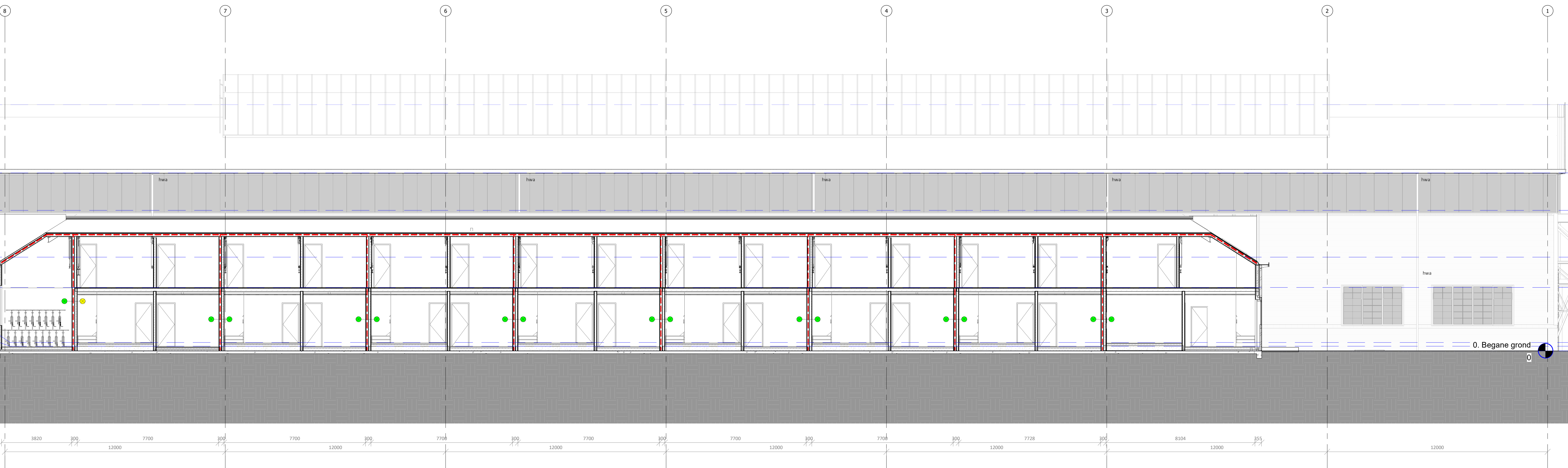
Doorsnede B-B 1 : 100 - nieuw
