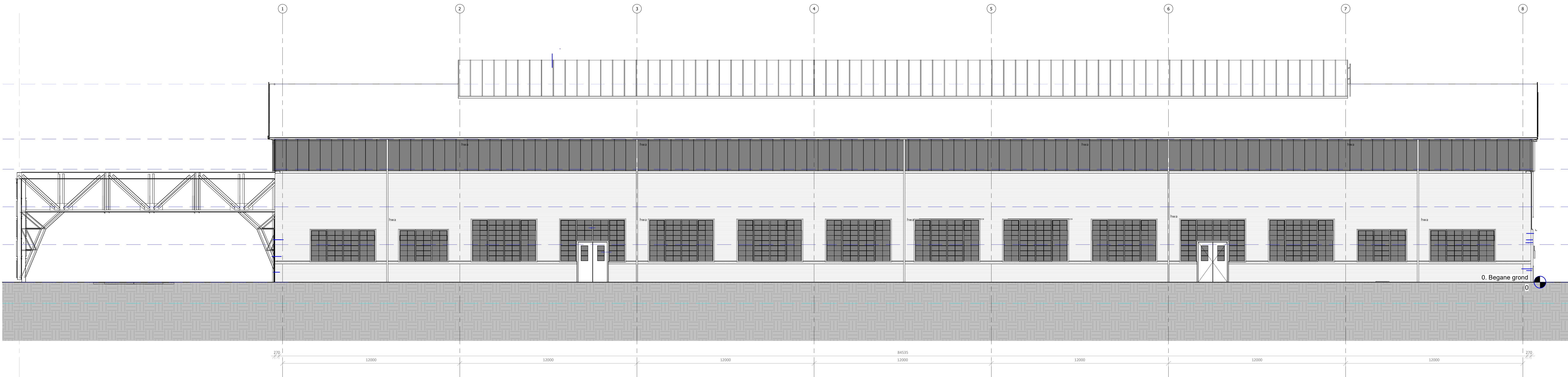
Oostgevel 1 : 100 - nieuw
