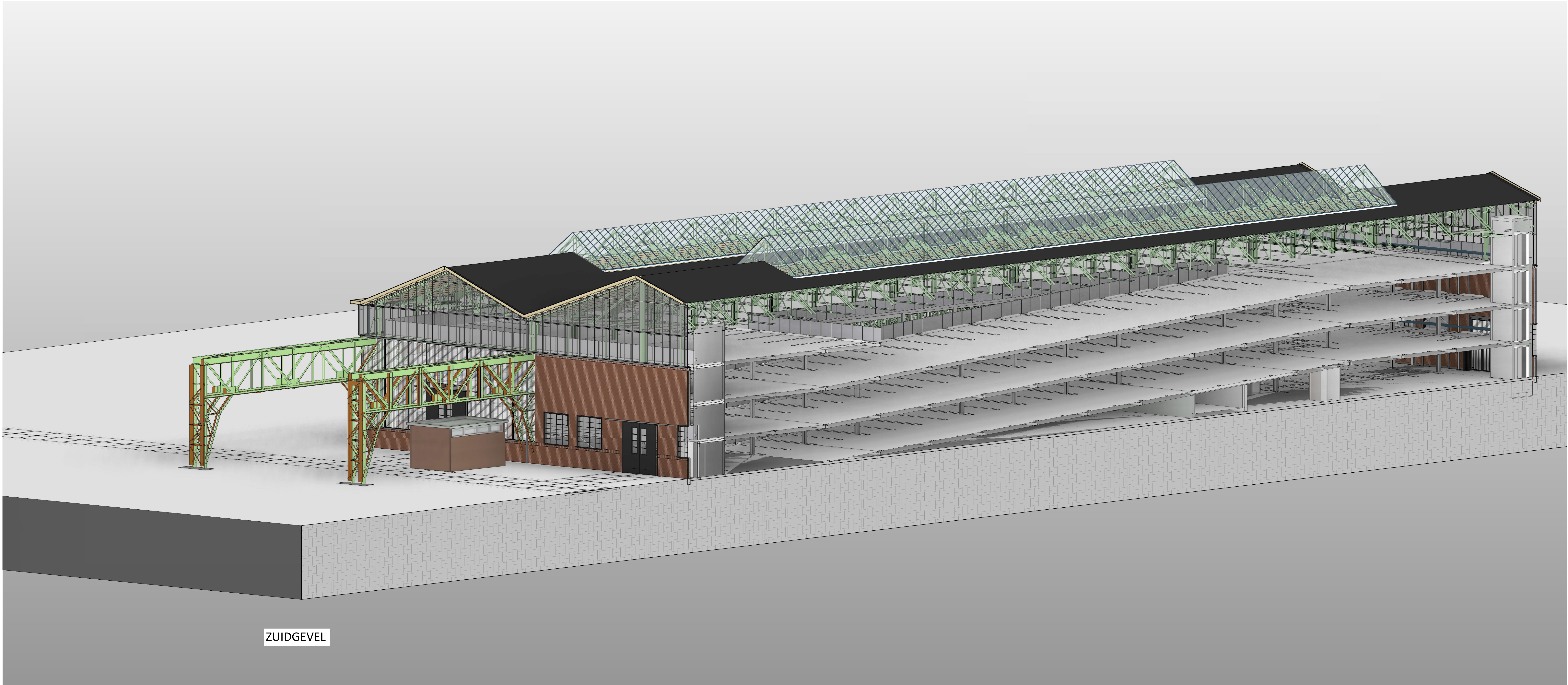
OV_3D impressie garage 1 - nieuw
