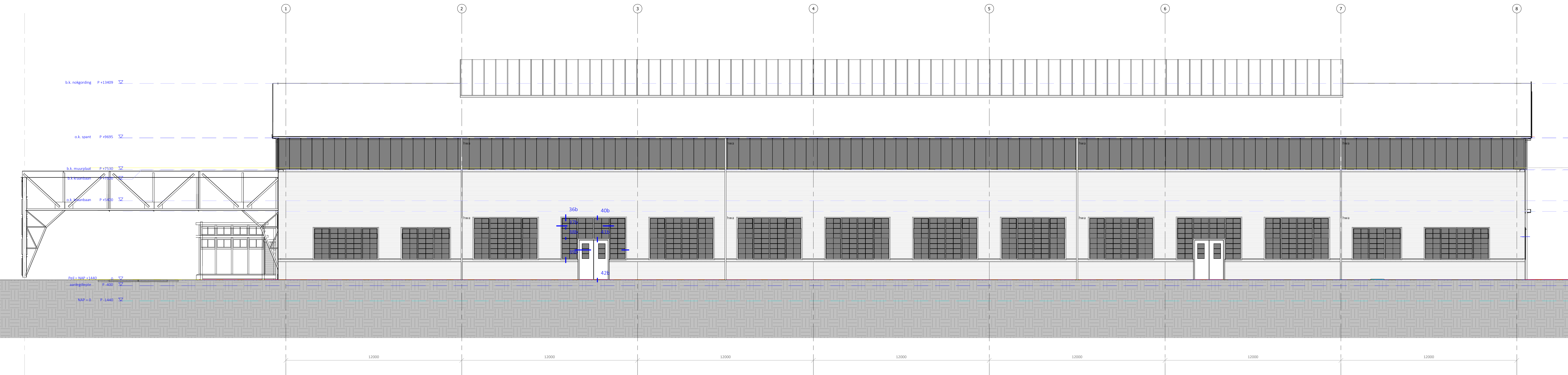
Oostgevel 1 : 100 - bestaand
