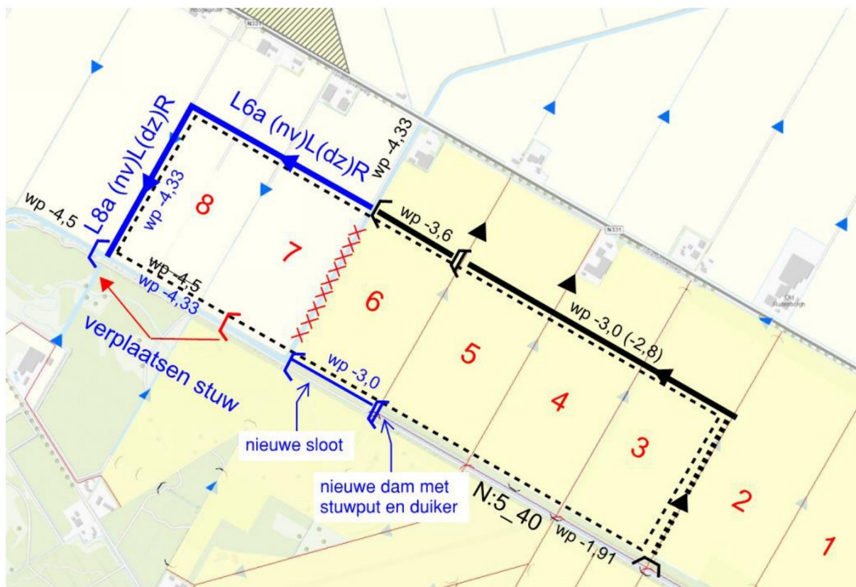
Figuur 16 – omleggen Voorstertocht (schematisch)
