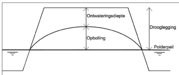
Figuur 12 –Drooglegging en ontwatering (bron: Waterkader)
