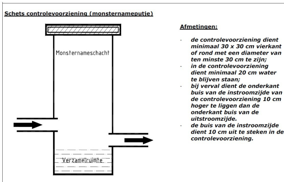
Figuur 26 – schets controlevoorziening (monsternameputje)
