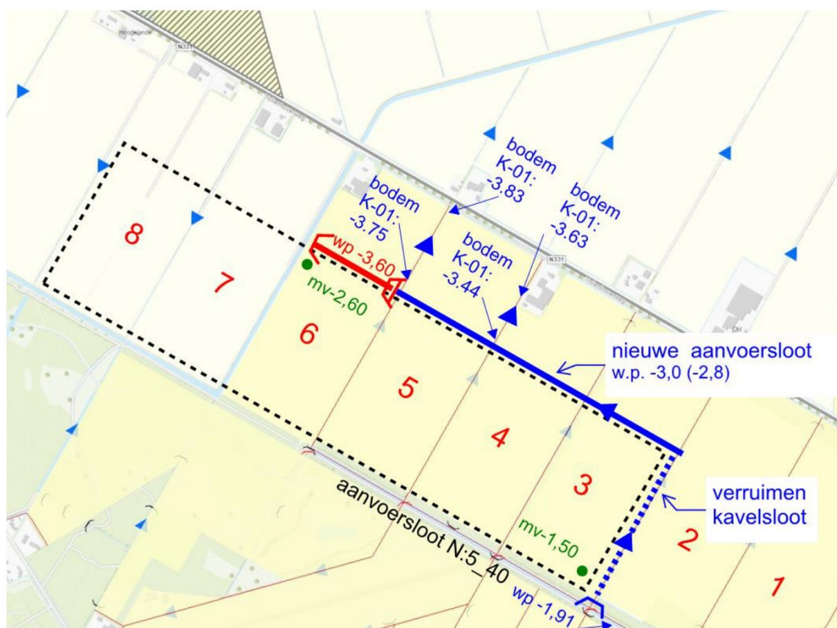
Figuur 15 – Nieuwe aanvoersloot (schematisch in blauwe lijnen)
