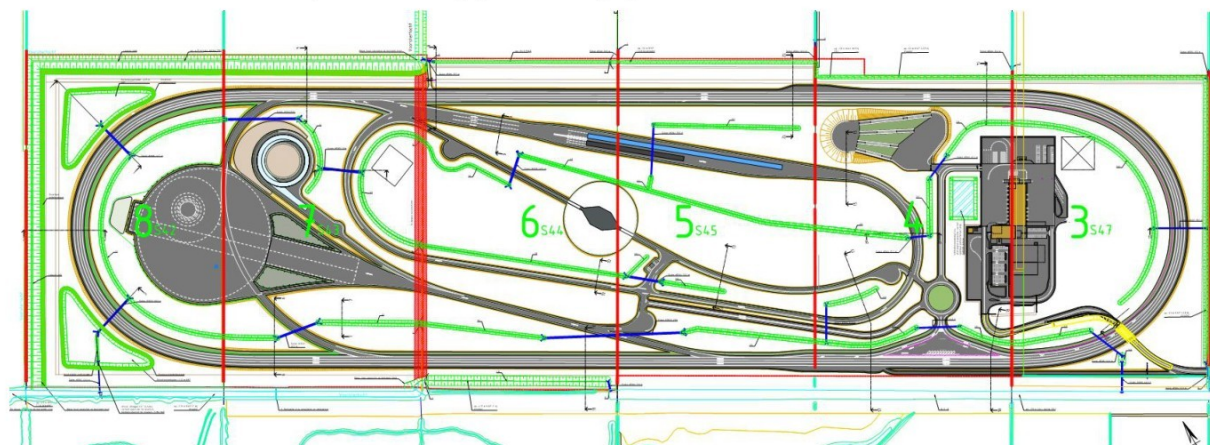
Figuur 27 – Concept referentie ontwerp watergangen d.d. 11-10-2022 (fragment tekening 19508-RO-O-0001 (tussenversie))
