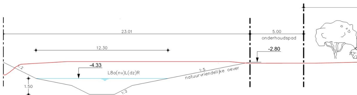
Figuur 31 – Voorstertocht langs westzijde kavel 8; profiel L8a(nv)L(dz)R
