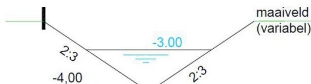
Figuur 28 profiel nieuwe aanvoersloot langs oost- en noordzijde
