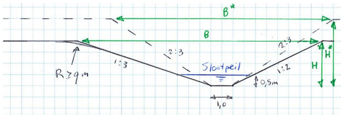
Figuur 33 – schematisch profiel bermsloten
