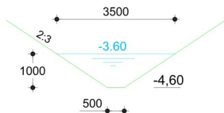
Figuur 32 profiel neuesloot langs noordzijde kavel 6
