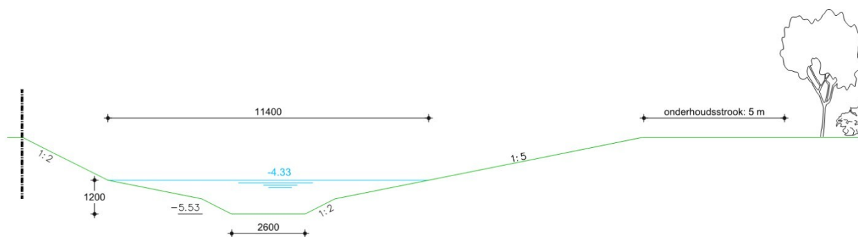
Figuur 30 – Voorstertocht langs noordzijde kavel 7 en 8; profiel L6a(nv)L(dz)R
