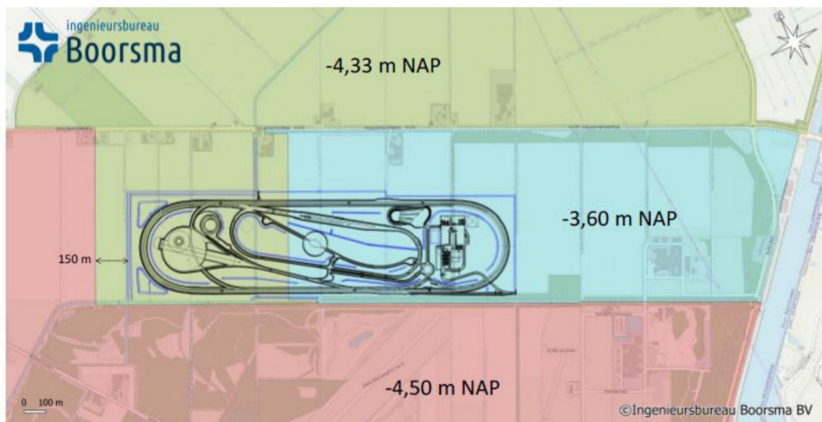
Figuur 18 – toekomstig peilbesluit na realisatie MITC-basis (indicatief)
