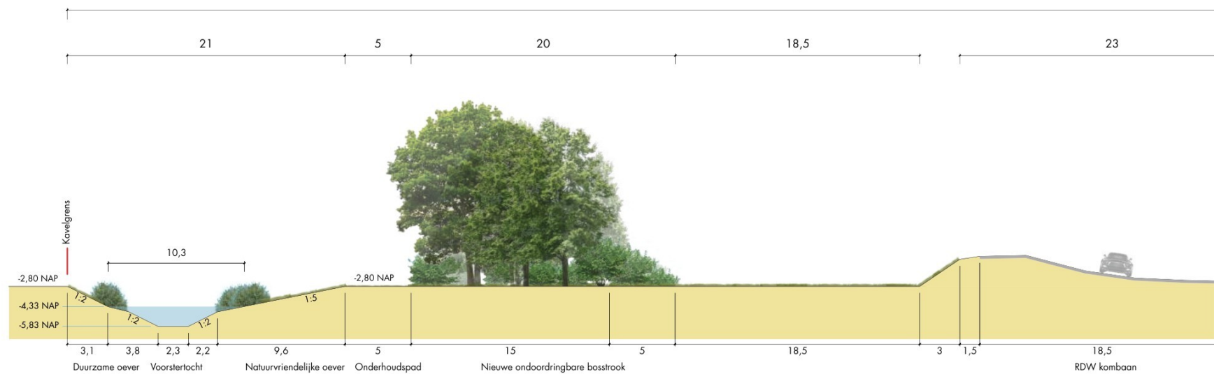
Afb. 42: Lengte doorsnede
