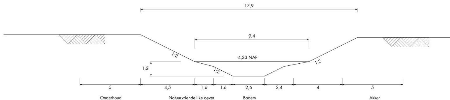
Afb. 20: Profiel L6a
