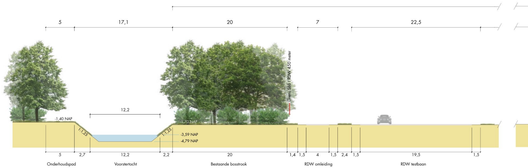
Afb. 40: Dwarsdoorsnede - kavel 5&6
