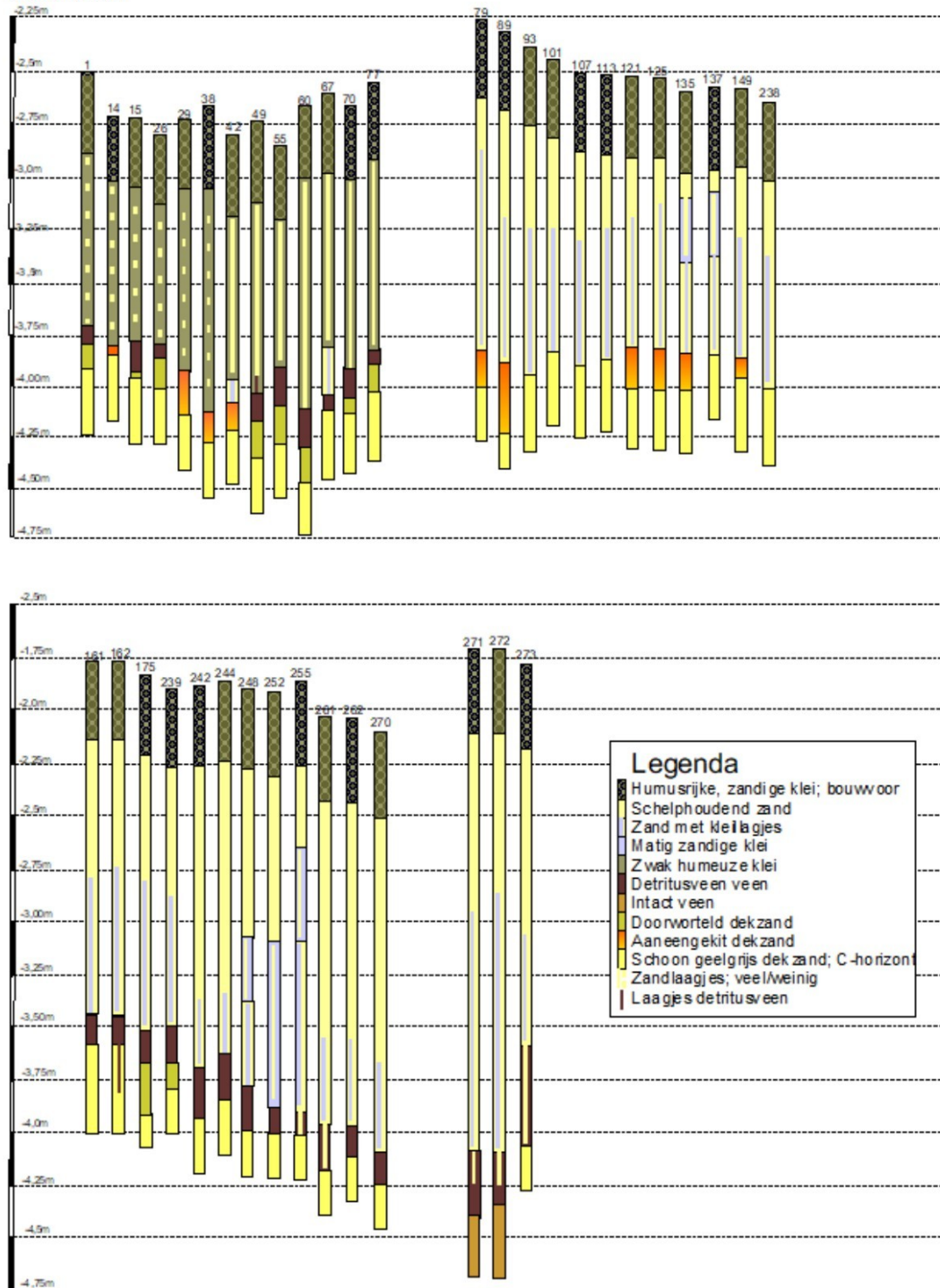
Figuur 9: Marknesse, Vollenhovevweg: De resultaten van het booronderzoek in de vorm van drie zuidwest-noordoost gerichte boorprofielen en een boorprofiel door het meest zuidwestelijke deel van het plangebied (boringen 271 tot en met 273).
