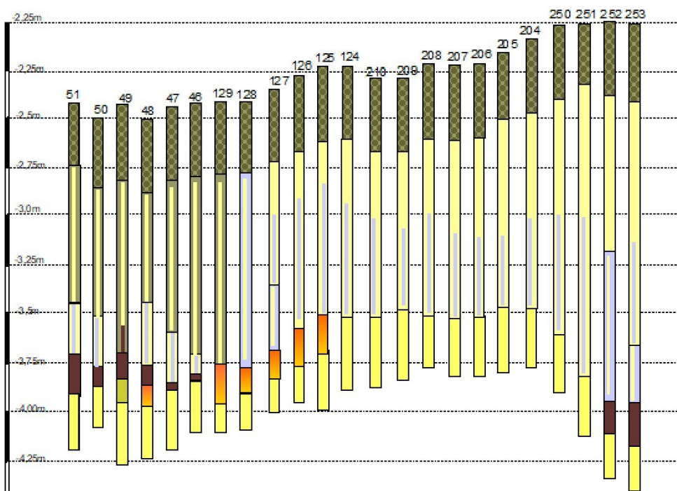
Figuur 7: Marknesse, Vollenhovevweg: De resultaten van het booronderzoek op het noordelijke deel van het plangebied in de vorm van twee noordwest-zuidoost gerichte boorprofielen.
