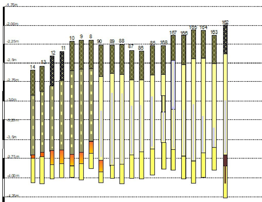
Figuur 8: Marknesse, Vollenhoverweg: De resultaten van het booronderzoek op het zuidelijke deel van het plangebied in de vorm van twee noordwest-zuidoost gerichte boorprofielen.
