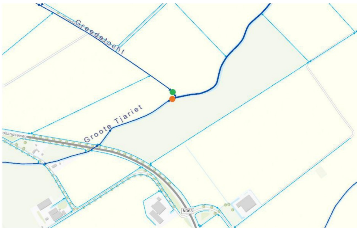
Figuur 1: De groene stip geeft globaal de locatie weer van de te vervangen stuw. De oranje stip geeft globaal de locatie weer van het aan te leggen gemaal met damwand.
