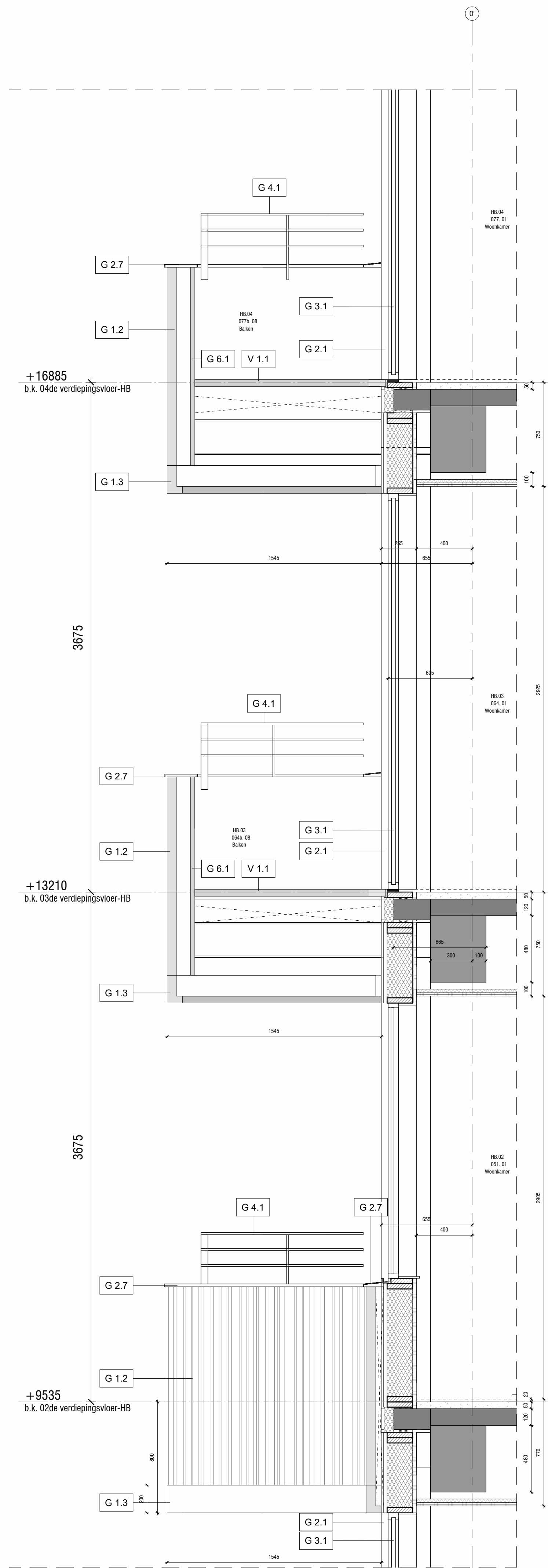
1 Doorsnede 1.1 1 : 20
