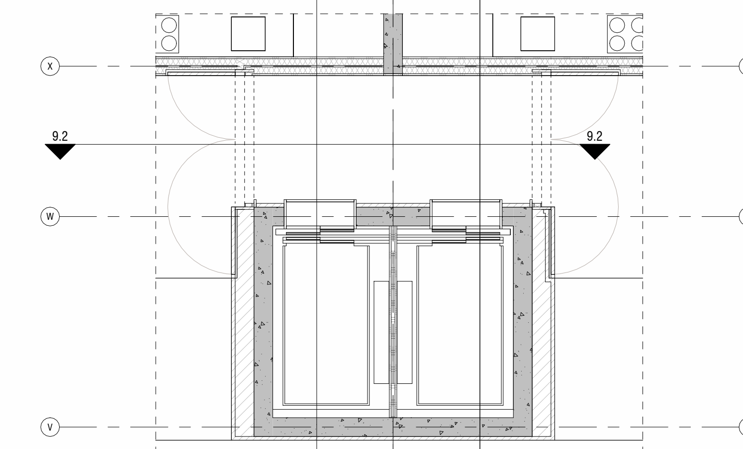
5 05 verdieping stijnpunt liften 1 : 50
