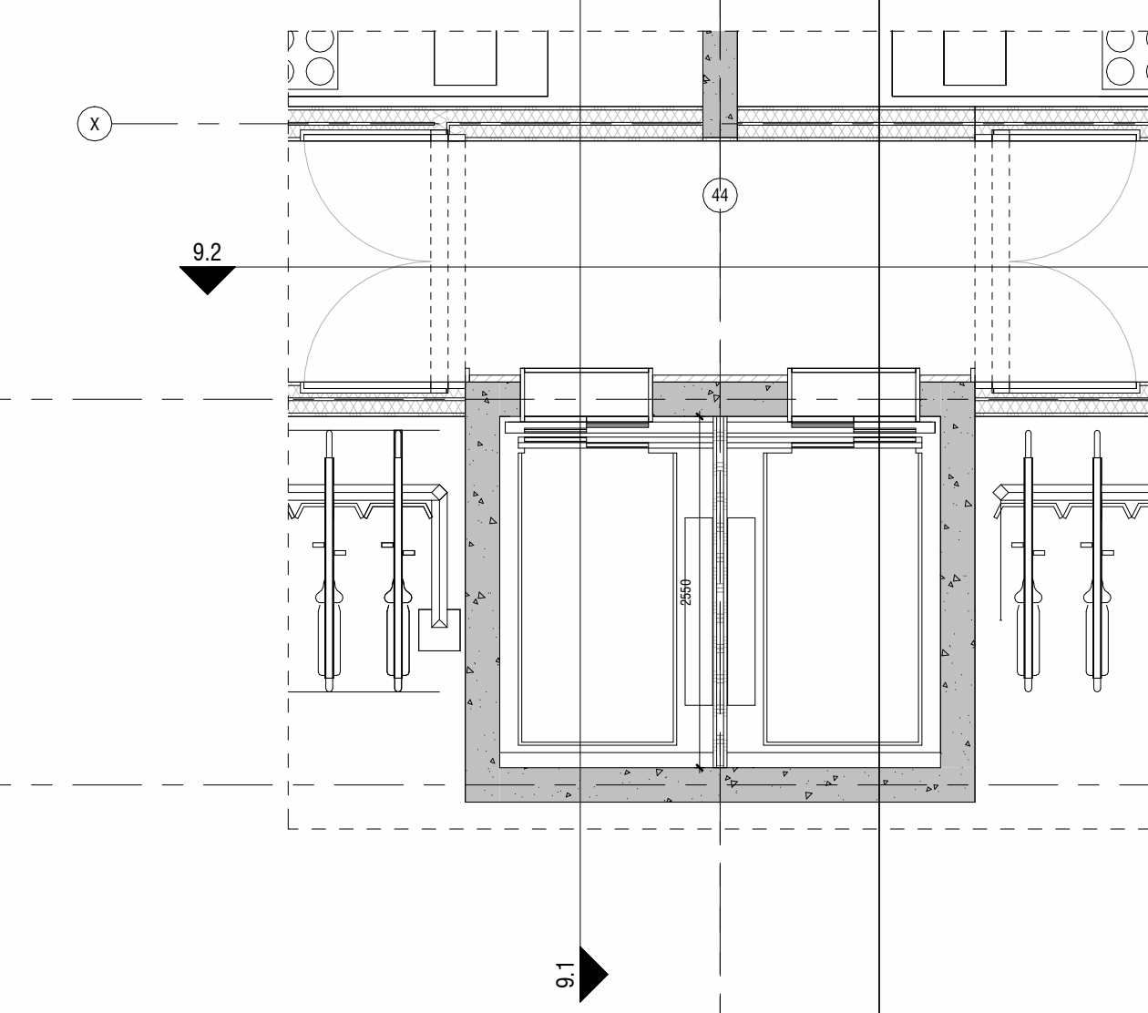
3 begane grond stijnpunt liften 1 : 50
