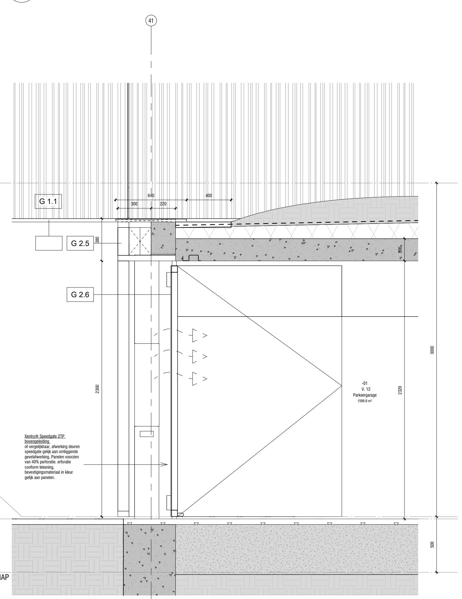
1 Doorsnede 7.1 1 : 20
