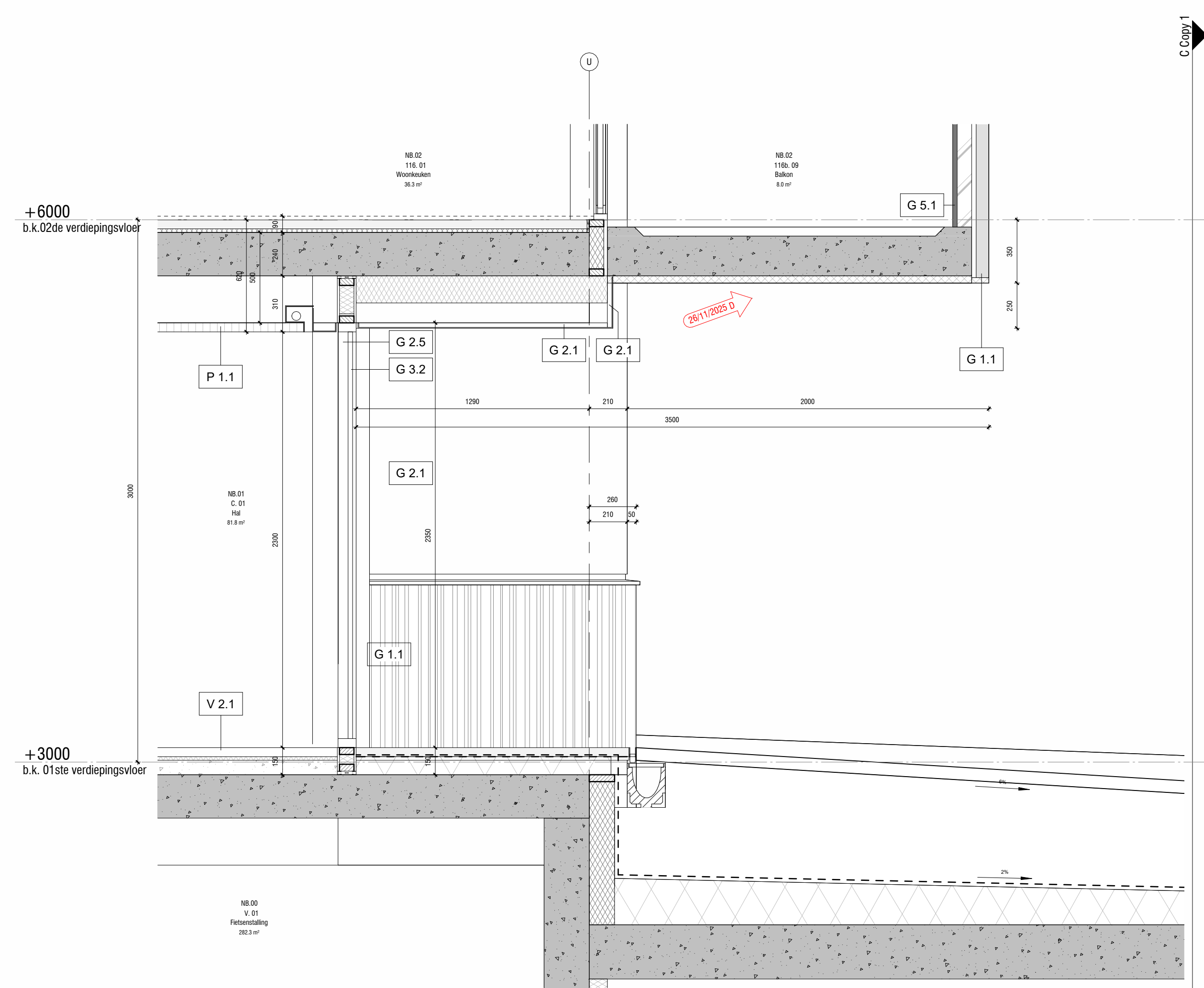
1 Doorsnede 4.1 1 : 20
