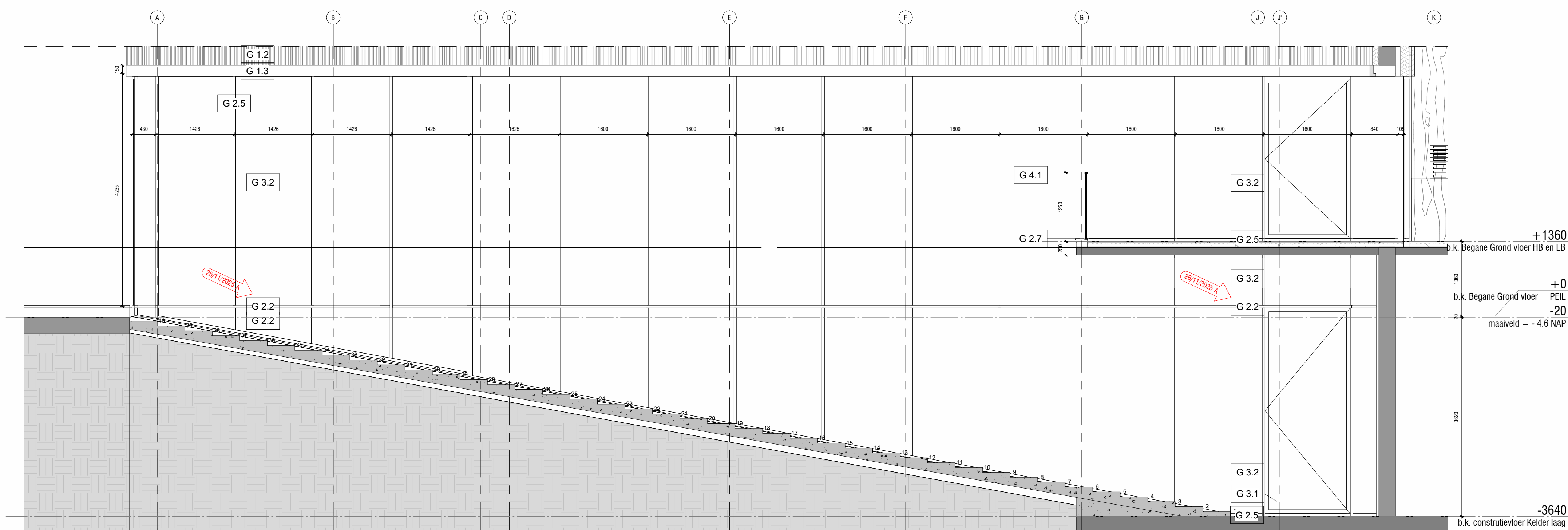
1 Gevelfragment 10.1 1:50
