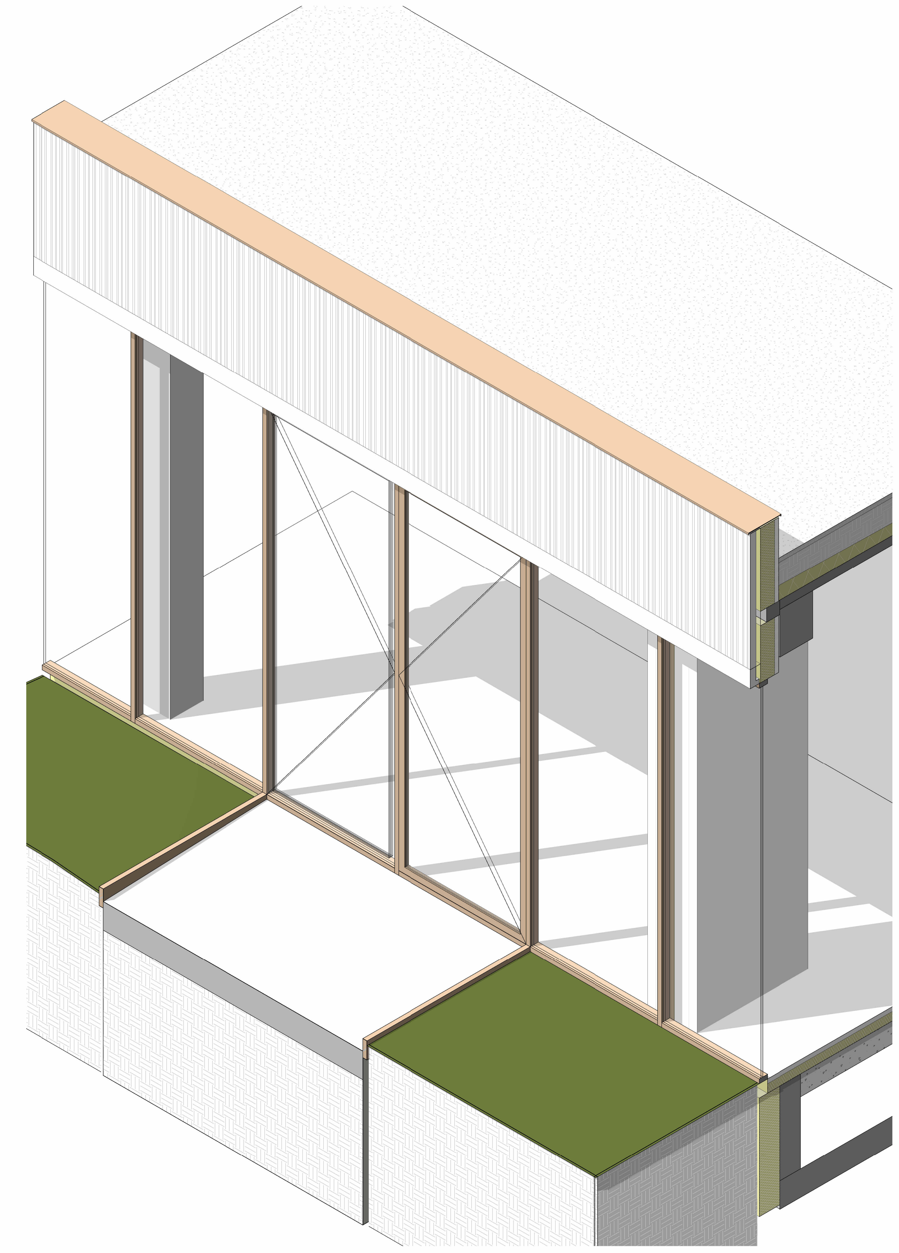
4 Axonometrie
