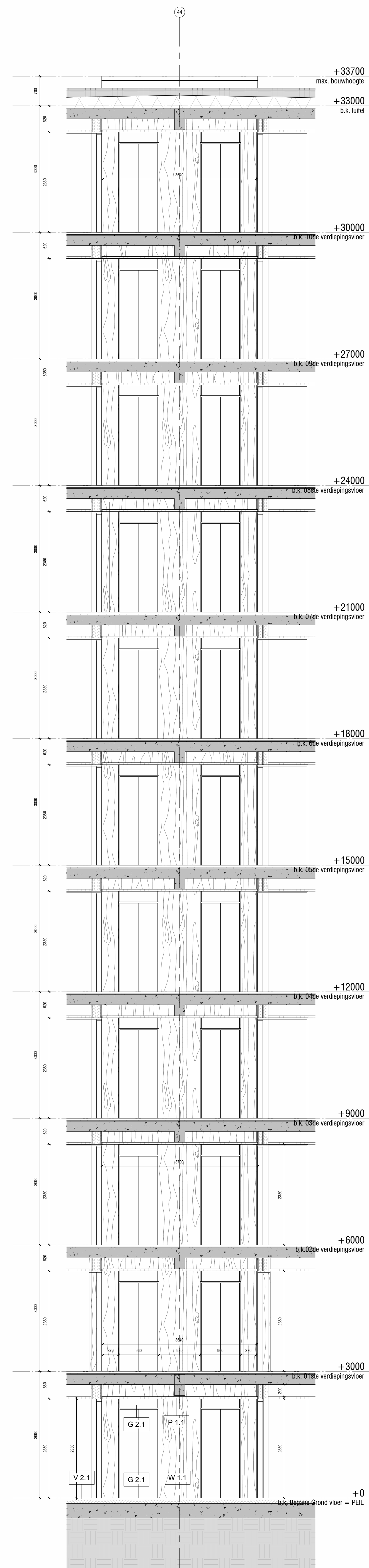
6 Doorsnede 9.2 1 : 50
