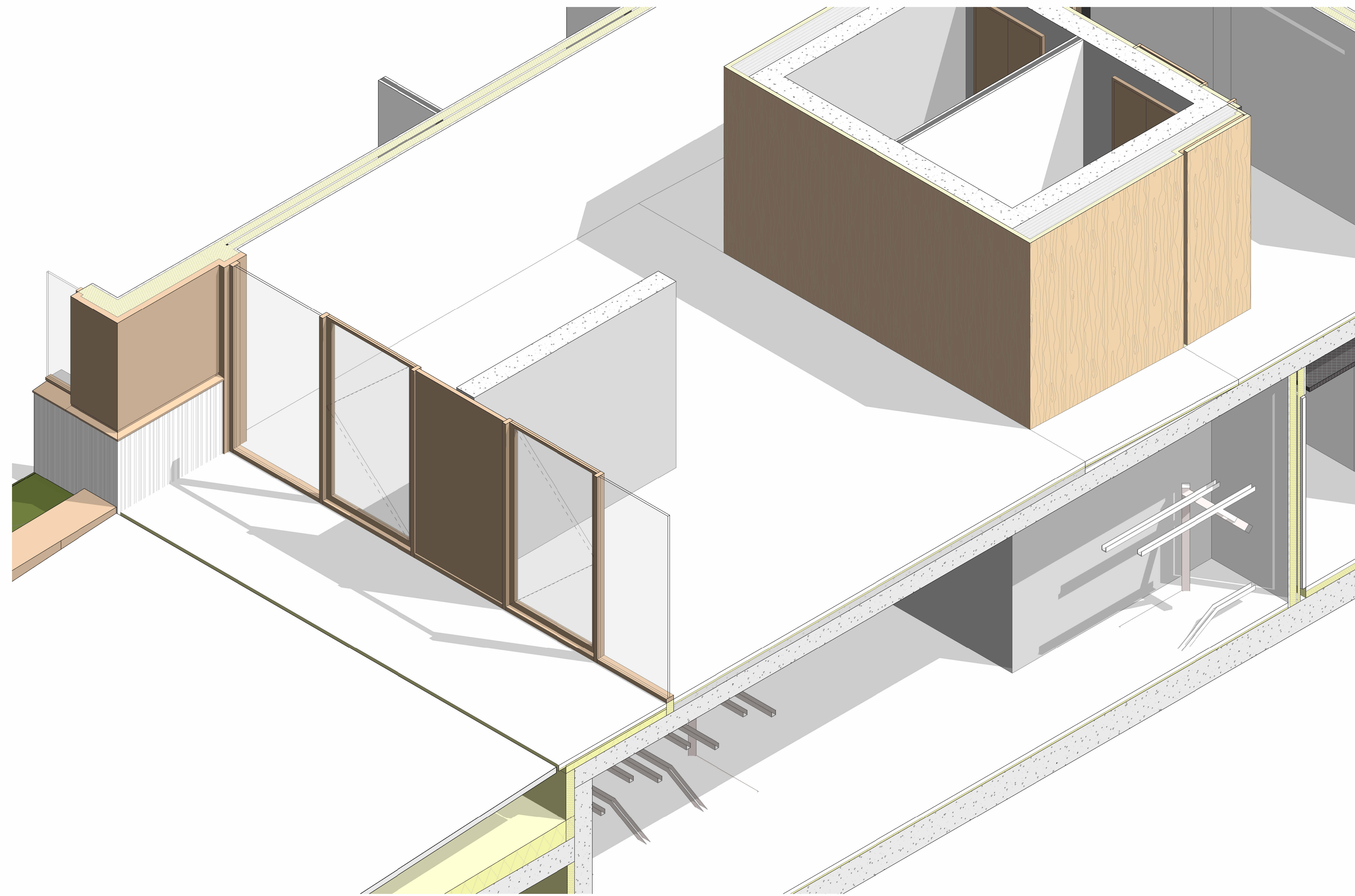
3 Axonometrie
