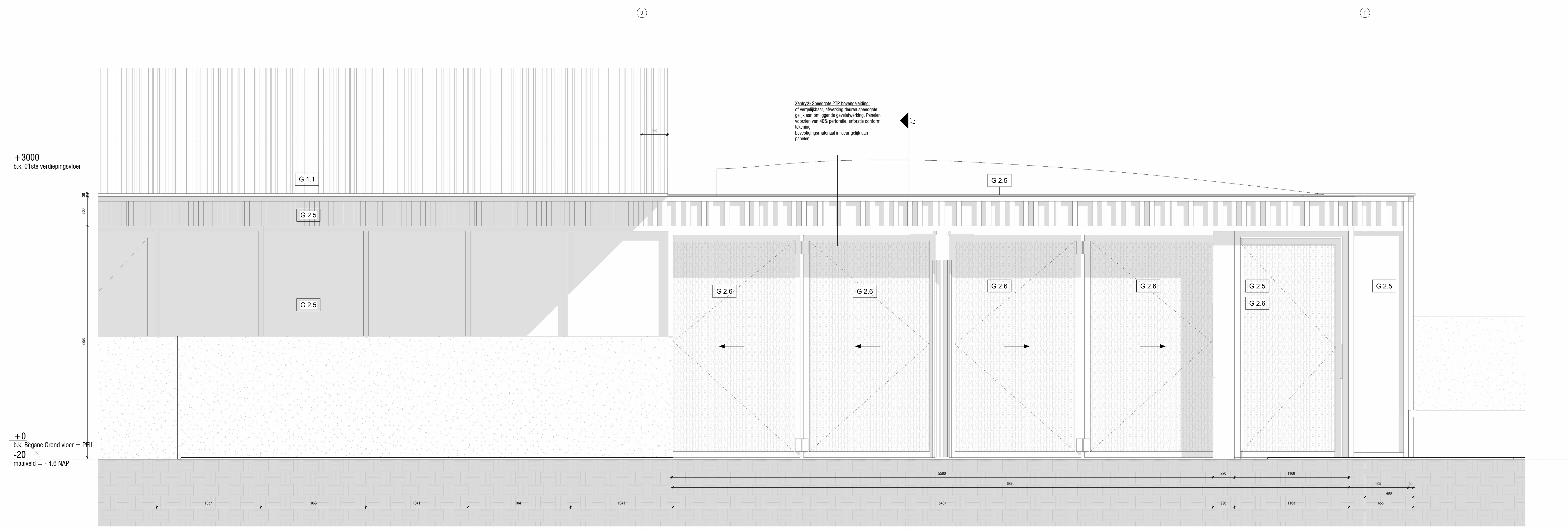
3 Gevelfragment 1 : 20
