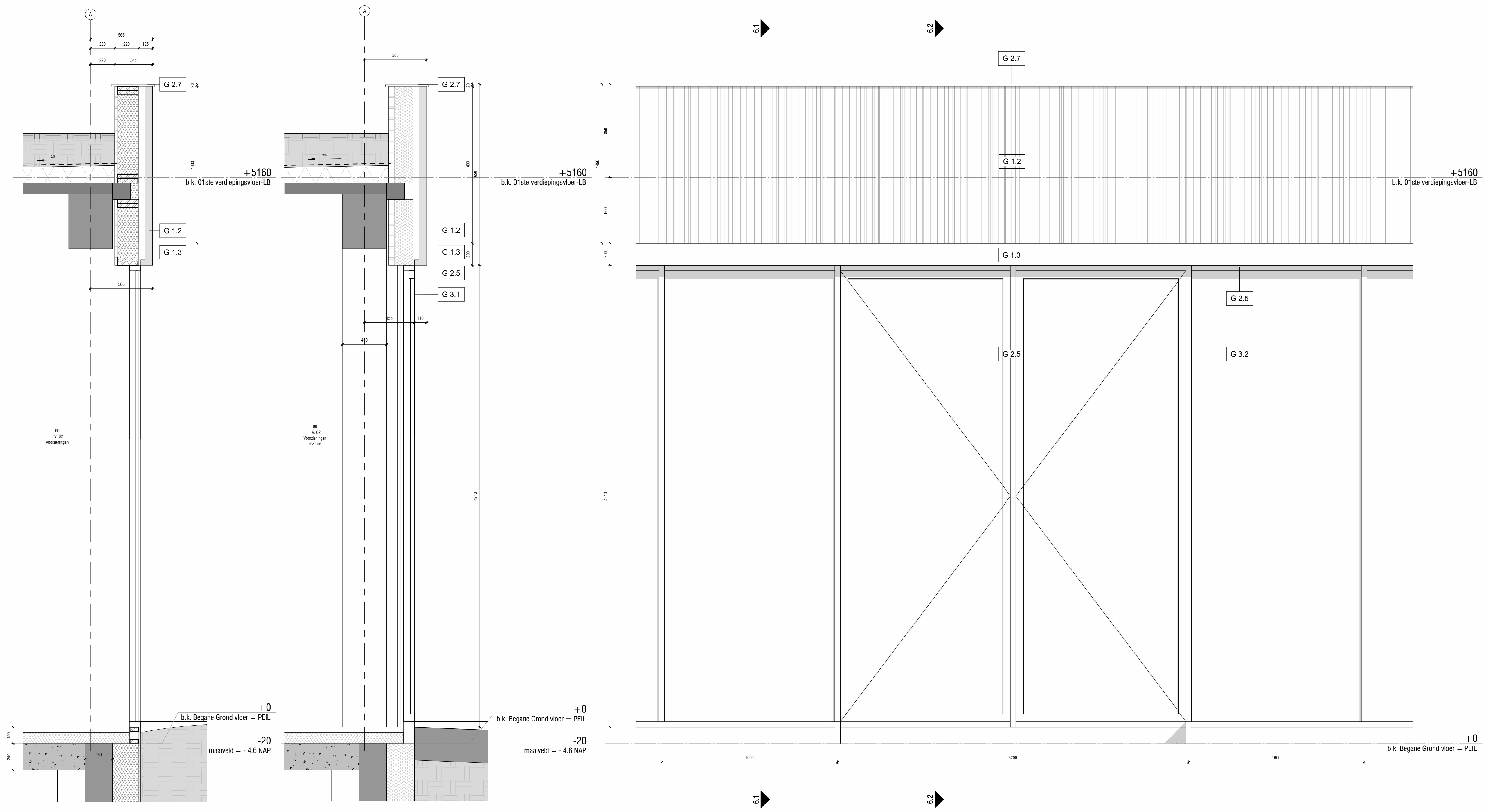
1 Doorsnede 6.1 1 : 20
