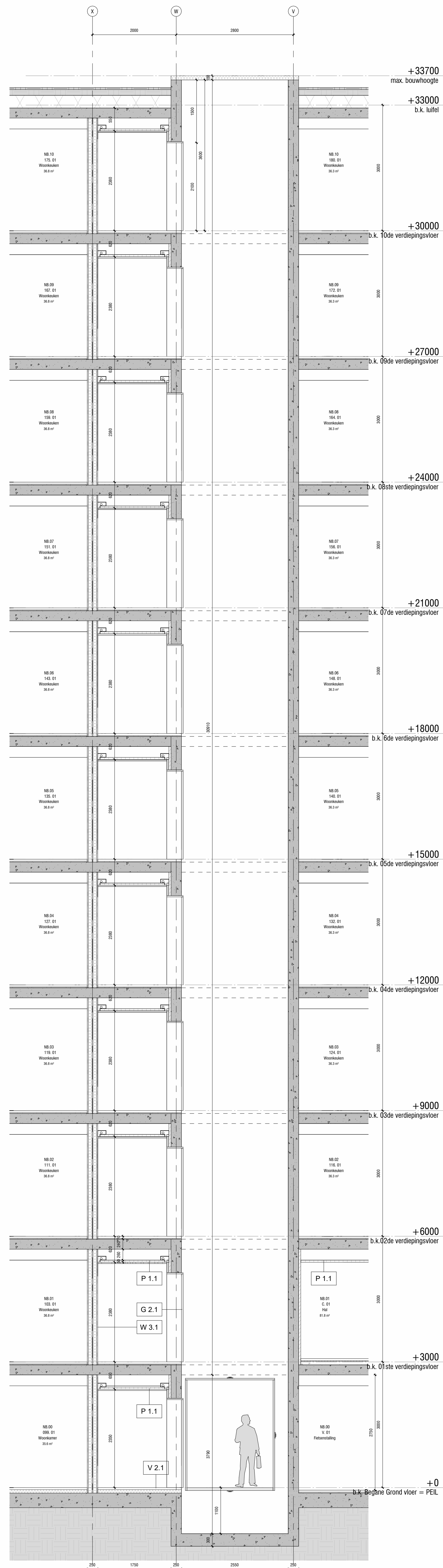
2 Doorsnede 9.1 1 : 50
