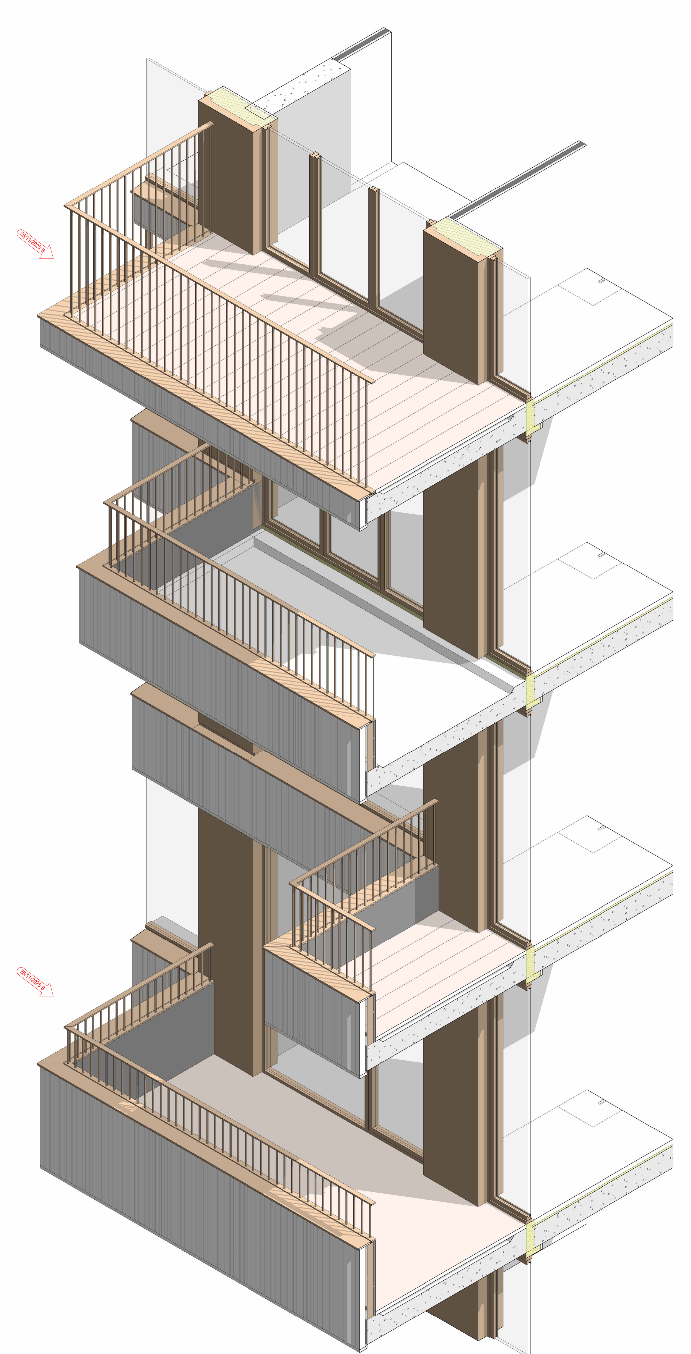
4 Axonometrie
