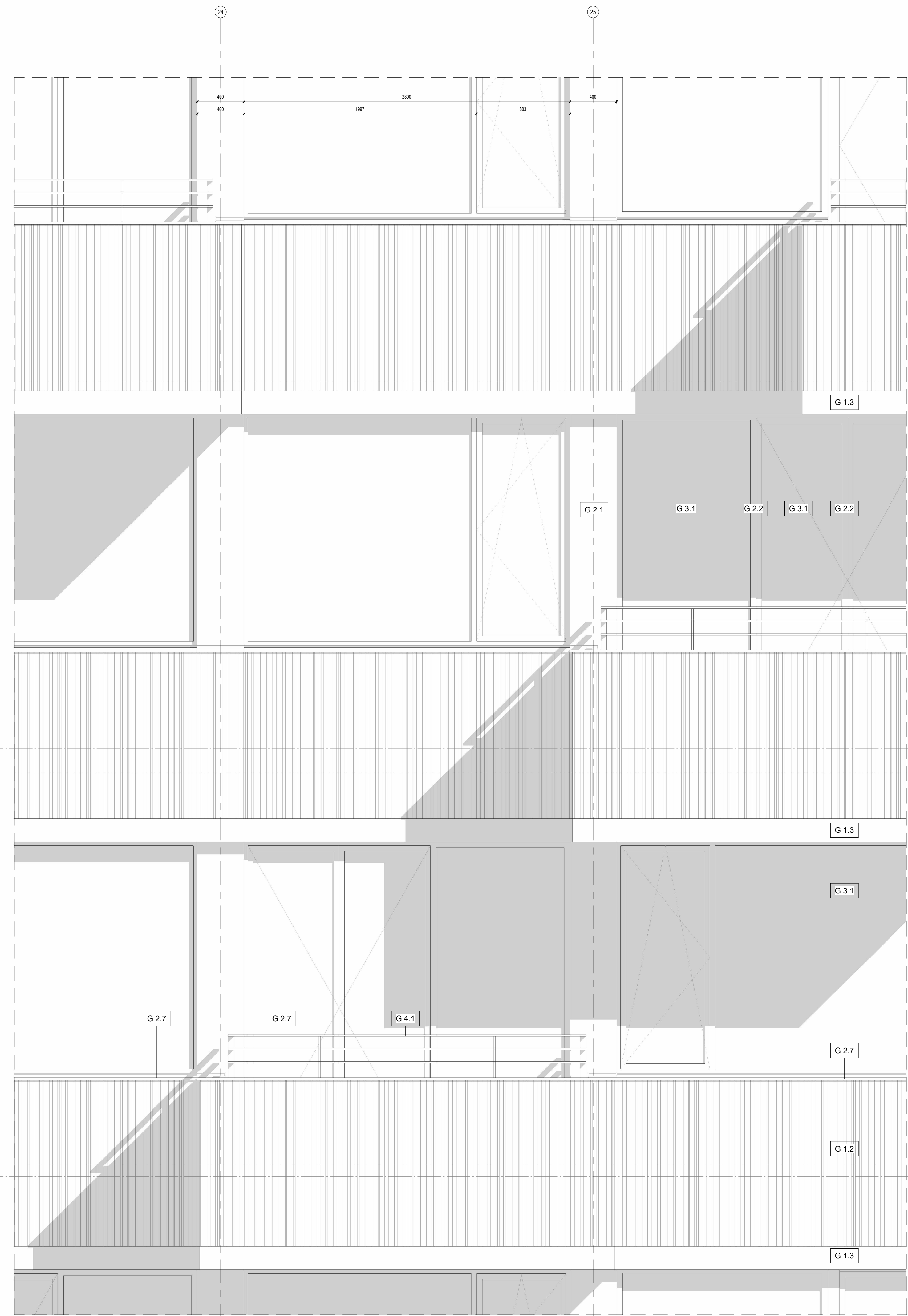
2 Gevelfragment 1 : 20
