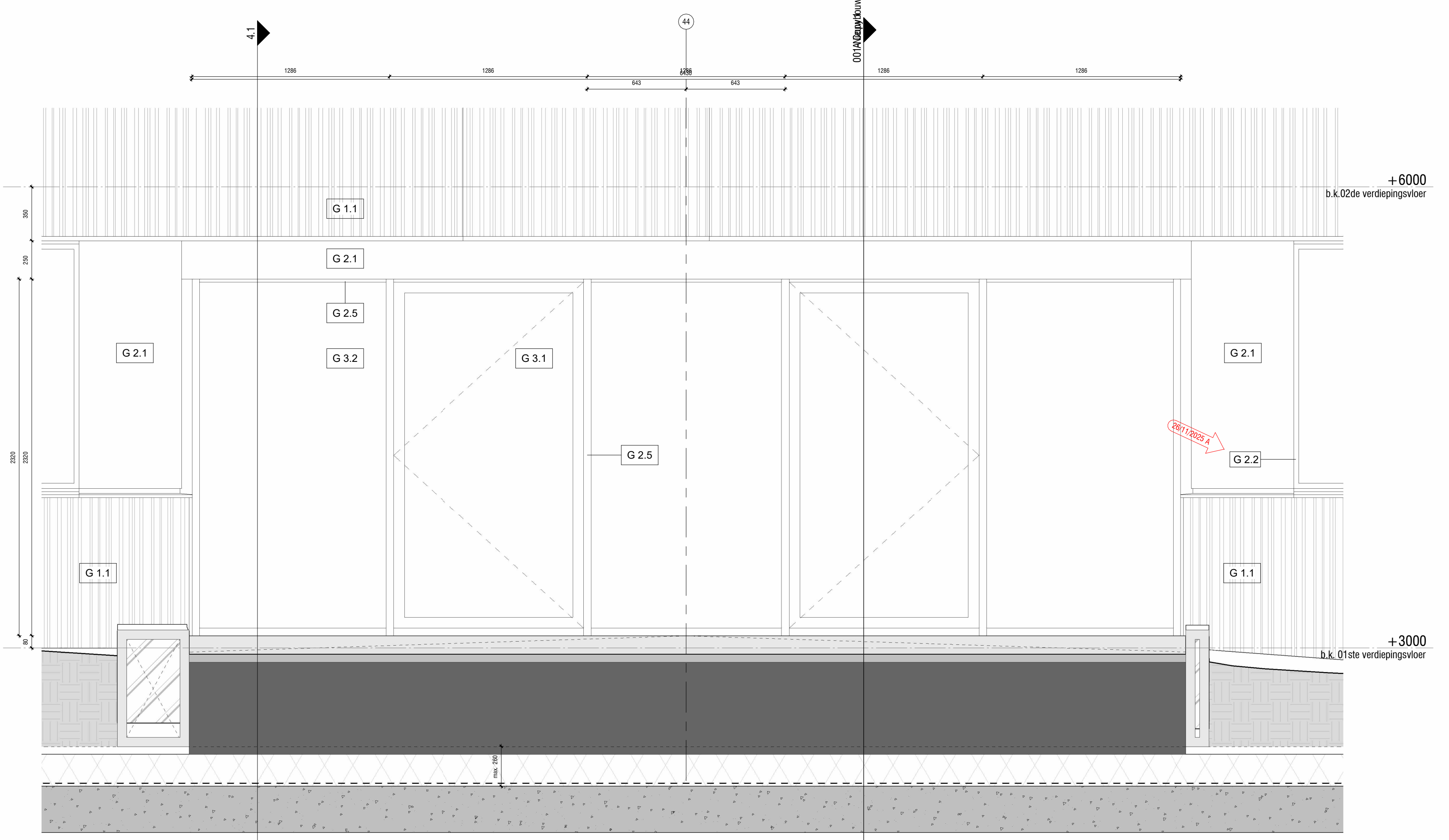
2 Gevelfragment 1 : 20
