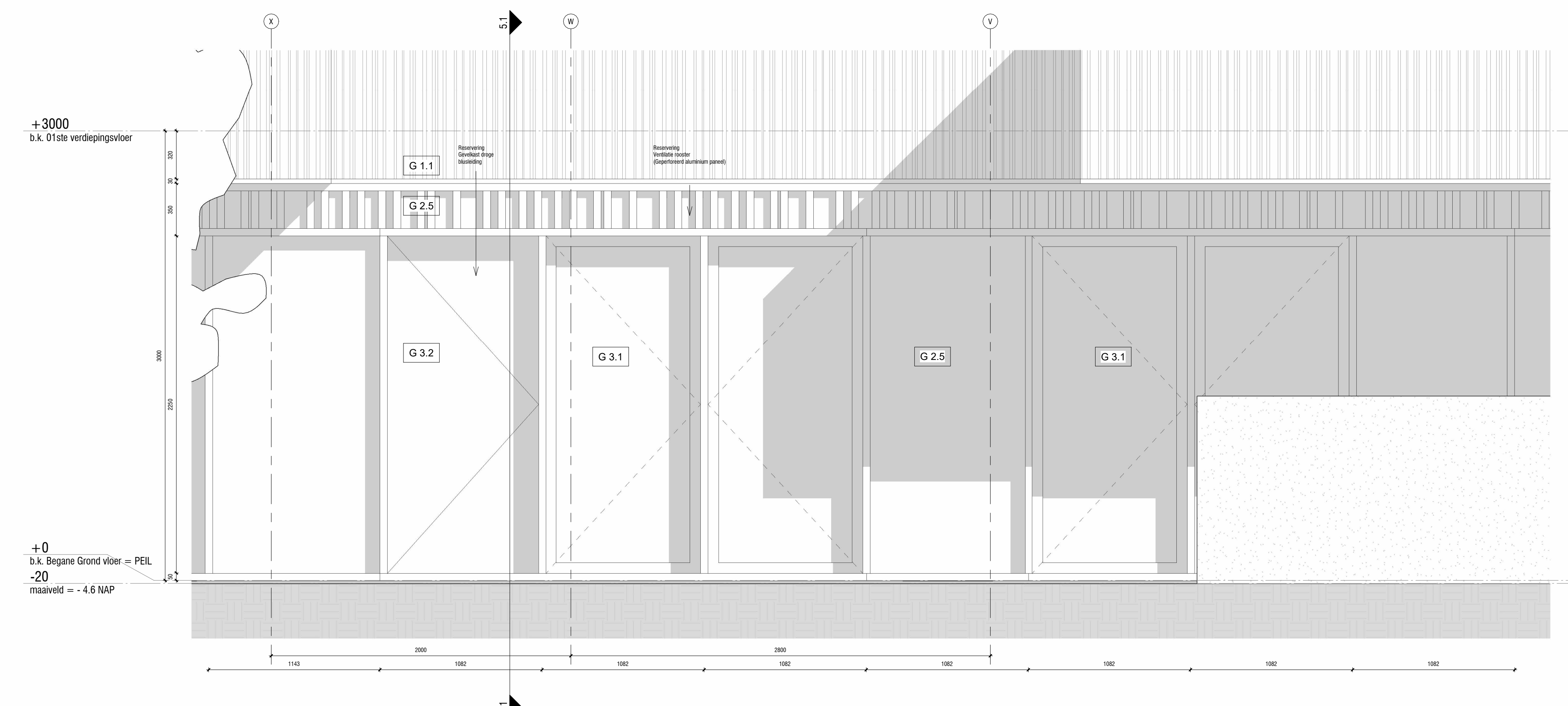
2 Gevelfragment 1 : 20
