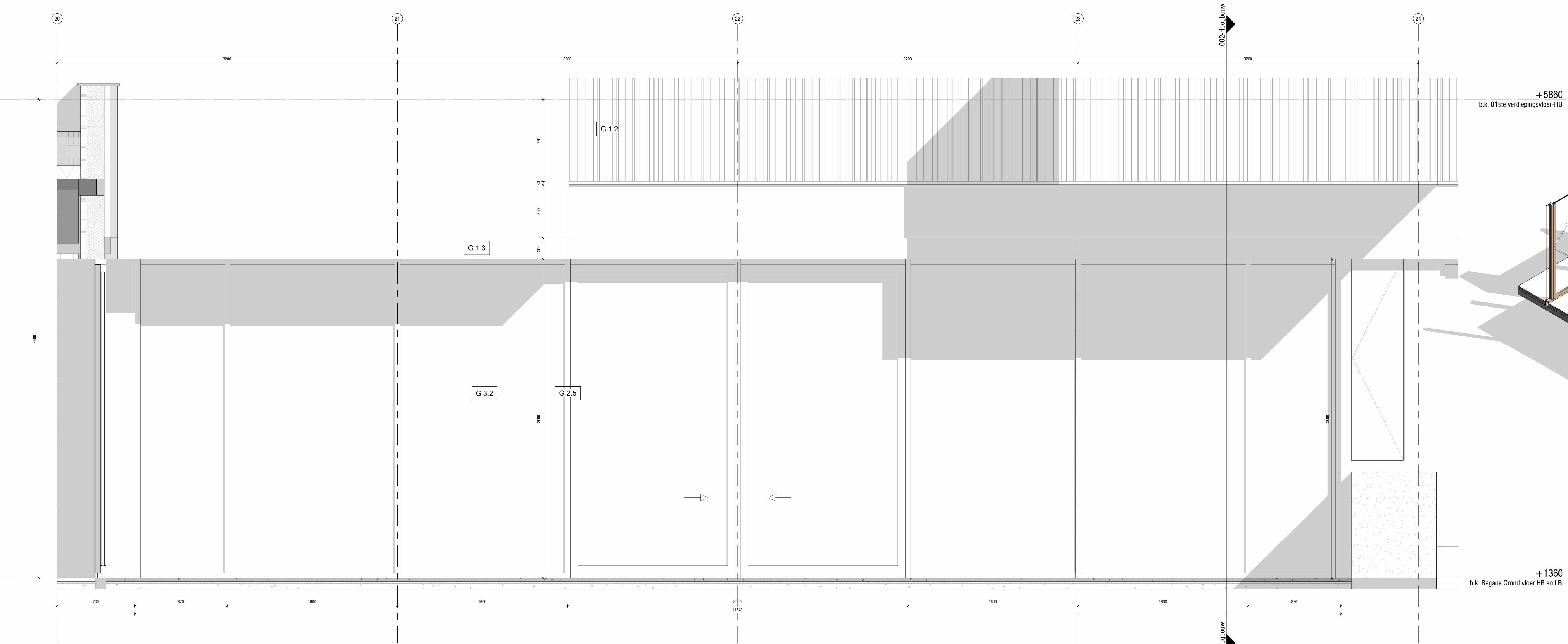
3 Gevelfragment 1:20
