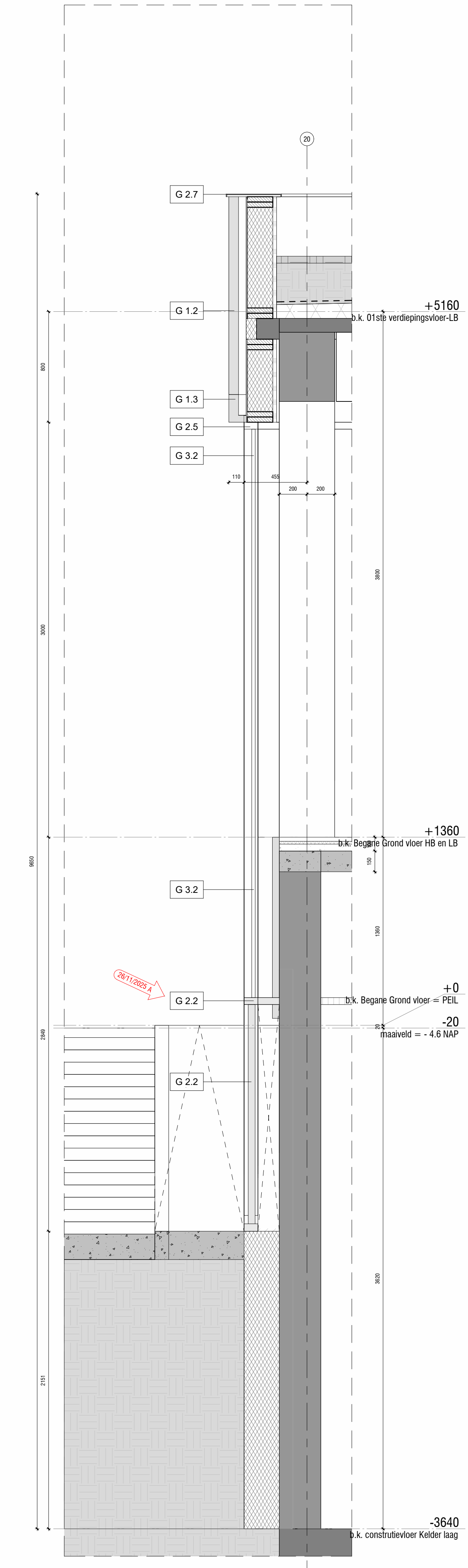
4 Doorsnede 10.3 1:20
