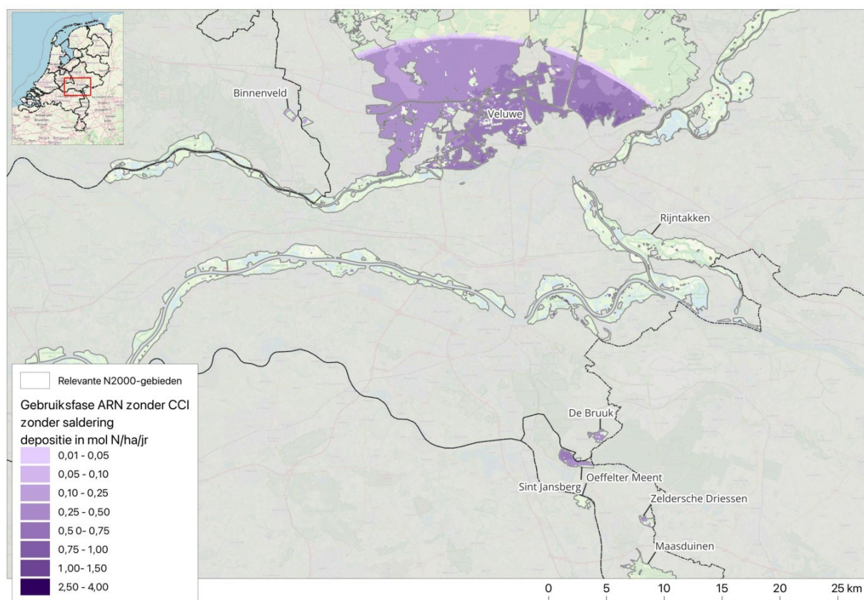
Afbeelding 2 Depositiebijdrage op (naderend) overbelast habitat door het project ARN met CCI in de beoogde situatie.
