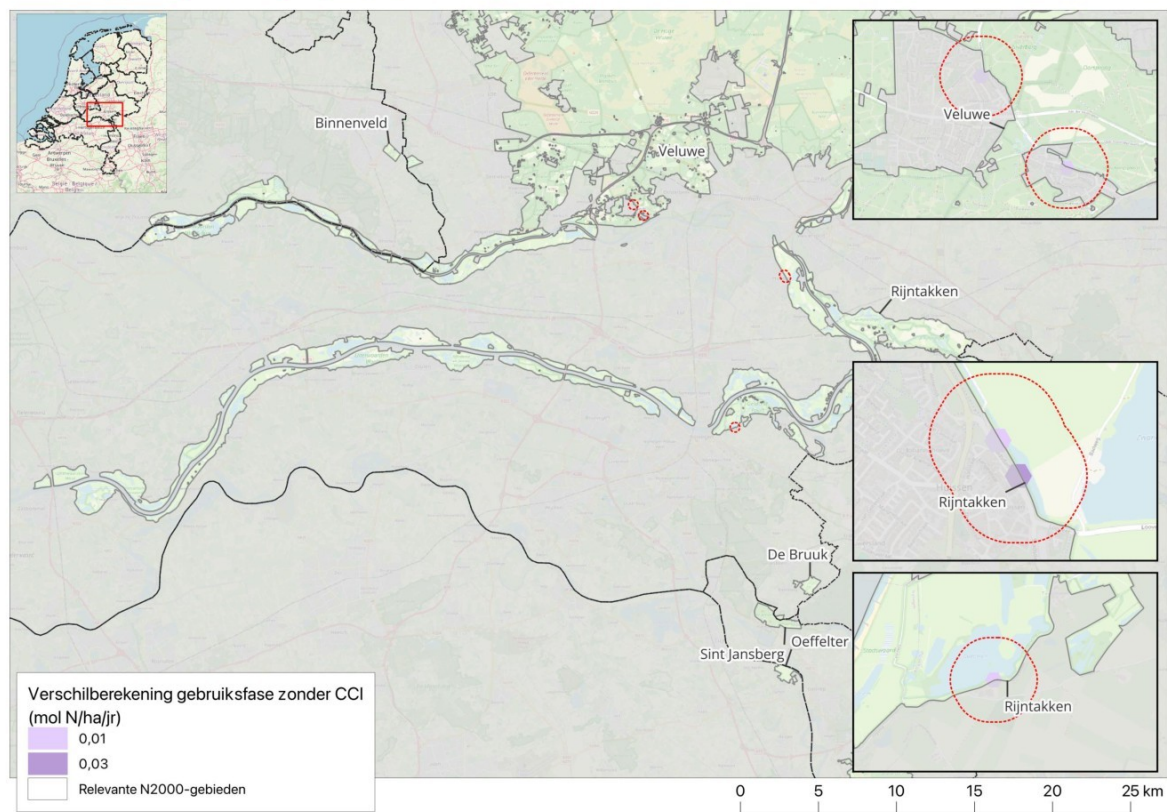
Afbeelding 7 Depositiebijdrage (alleen toenames) op (naderend) overbelast habitat na intern salderen in het scenario zonder CCI. Hexagonen met een toename zijn rood omcirkeld en in drie inzetten vergroot weergegeven.
