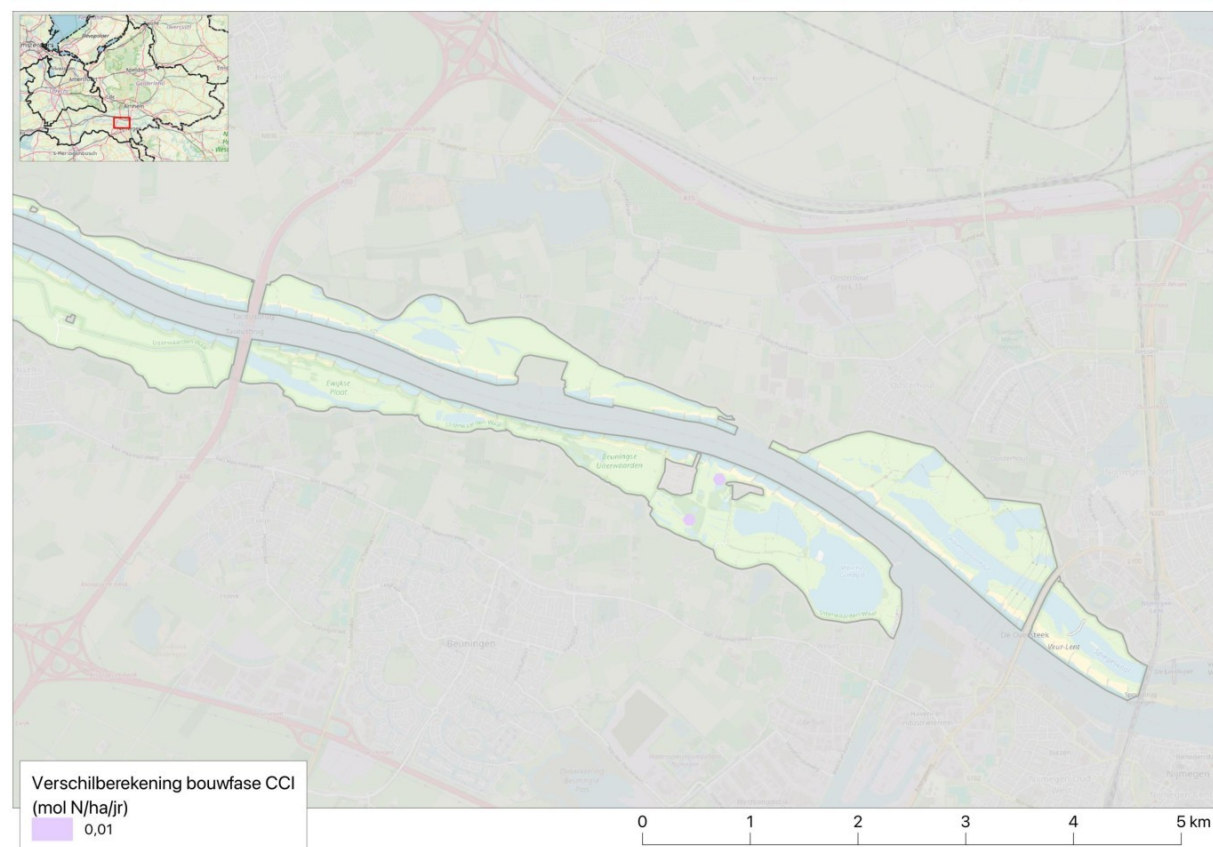
Afbeelding 1 Depositiebijdrage (mol N/ha/jr) ARN als gevolg van de realisatiefase.
