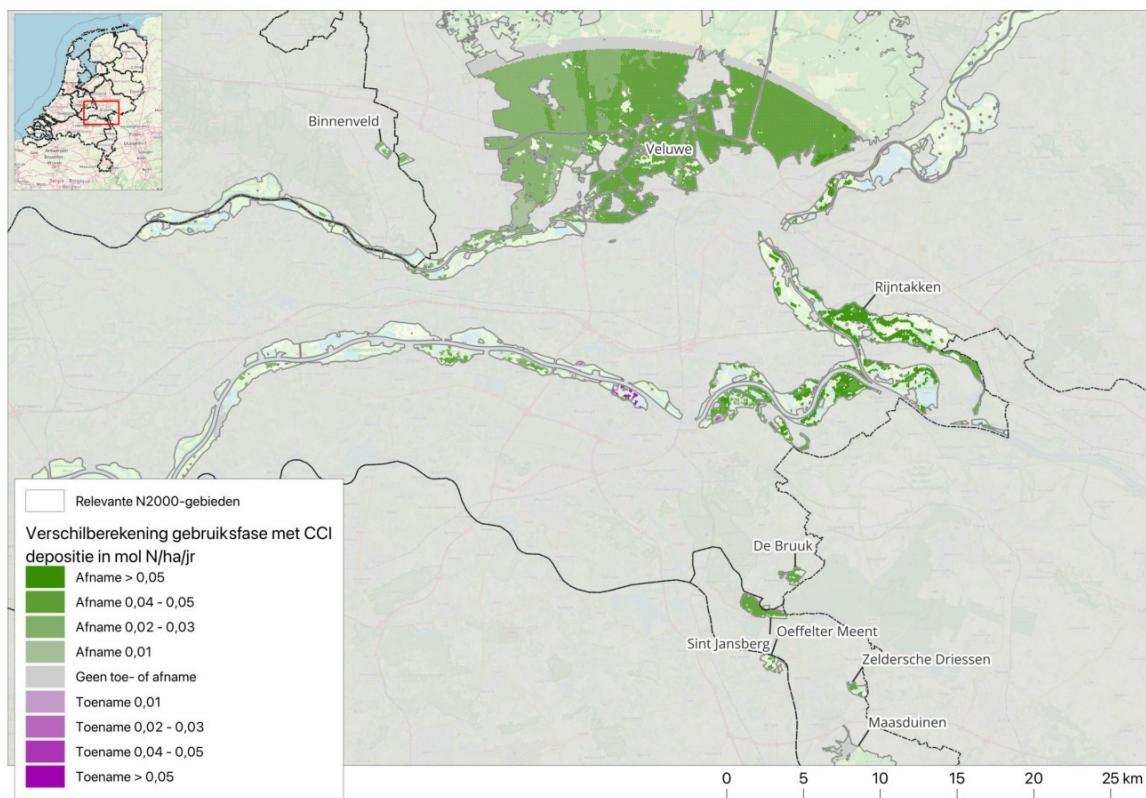
Afbeelding 4 Depositiebijdrage op (naderend) overbelast habitat na intern salderen in het scenario met CCI.
