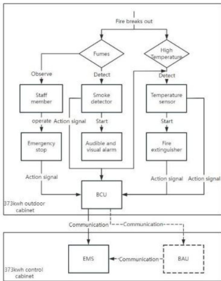
图 1-8 消防逻辑图 Figure 1-8 FSS Logic Diagram
