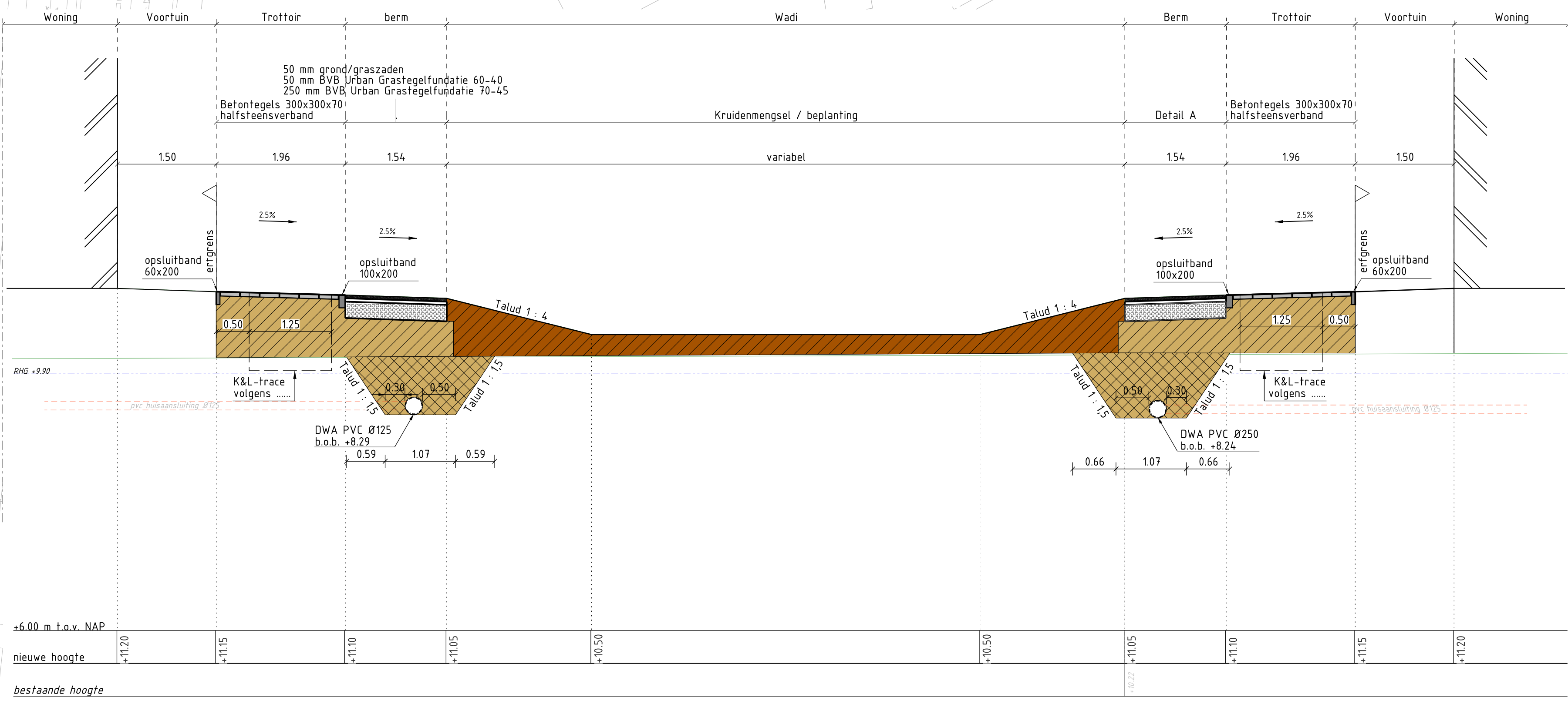
Dwarsprofiel 1
