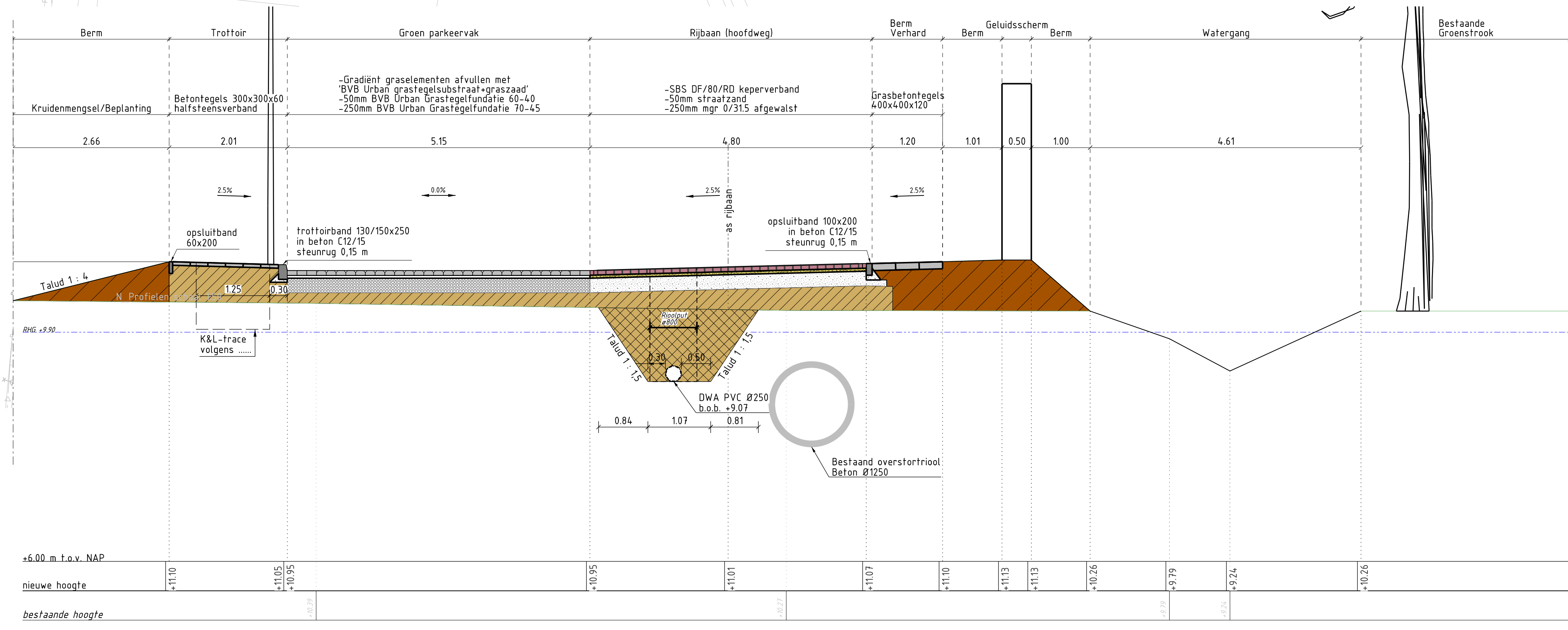
Dwarsprofiel 3
