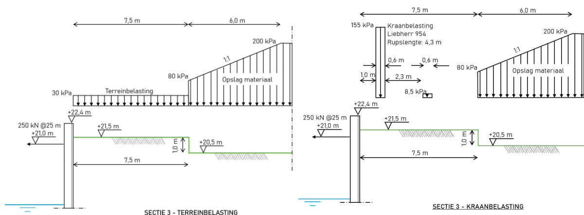
Figuur 4.4 Belastingsschema sectie 3
