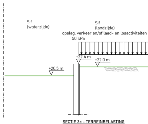
Figuur 4.7 Belastingschema sectie 3c
