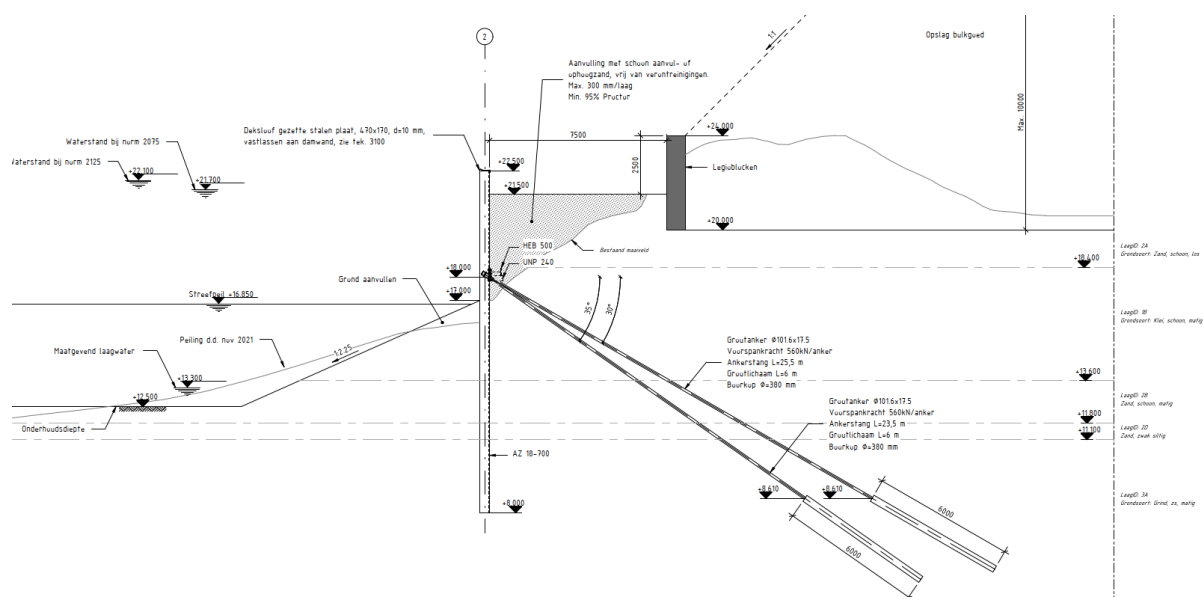
Figuur 5.8 Ontwerpproject kerende wand talud
