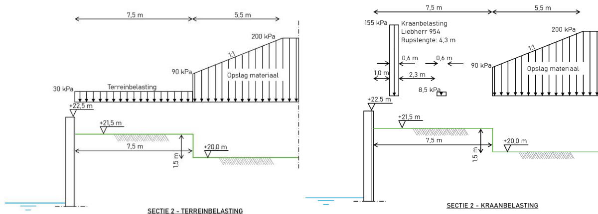
Figuur 4.3 Belastingsschema sectie 2
