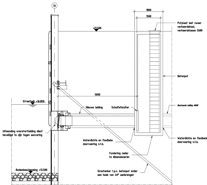
Figuur 8.3 Put inclusief schuifafsluiter op de rioolleiding Gemeente Roermond ter borging waterveiligheid
