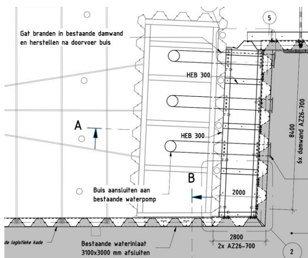
Figuur 5.10 Bovenaanzicht van de waterinnameconstructie VARO
