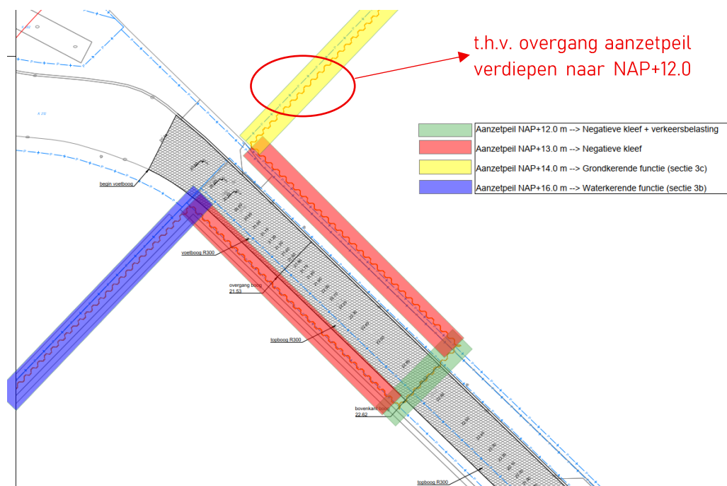
Figuur 7.5 Aanzetpeilen kerende wand op de landtong
