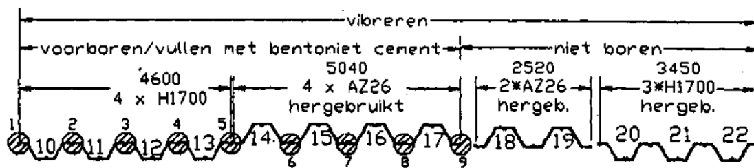
Figuur 11.5 Damwand proefopstelling Swalmen [65]
