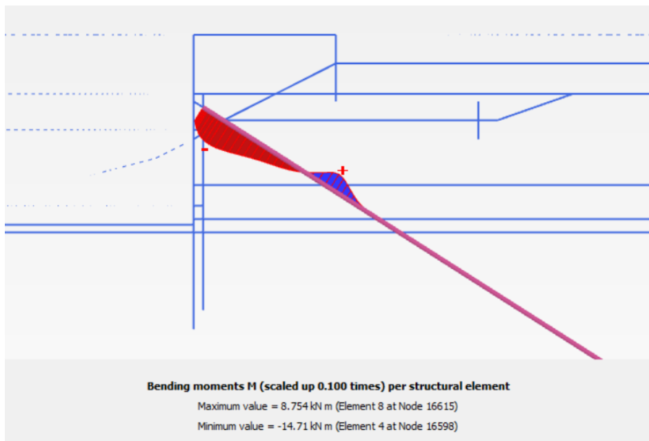
Figuur 7.7 Buigmomenten in SI-ankers t.g.v. zakkende grond – Fase 16. Val naar ELW – BGT
