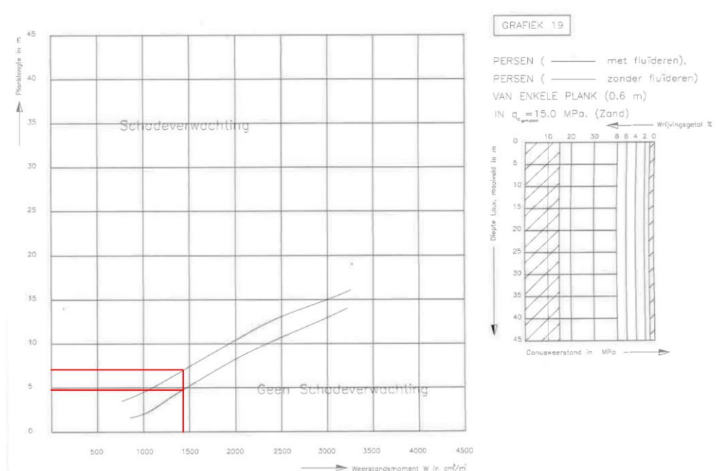
Figuur 11.1 NVAF/PSD-grafiek 19 – verwachting drukken damwand sectie 3b1 (trillingvrij)
