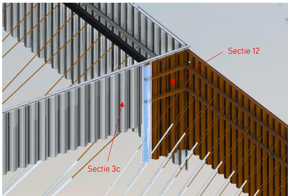
Figuur 5.13 Vleugelwand van sectie 12 t.o.v. kerende wand sectie 3c.
