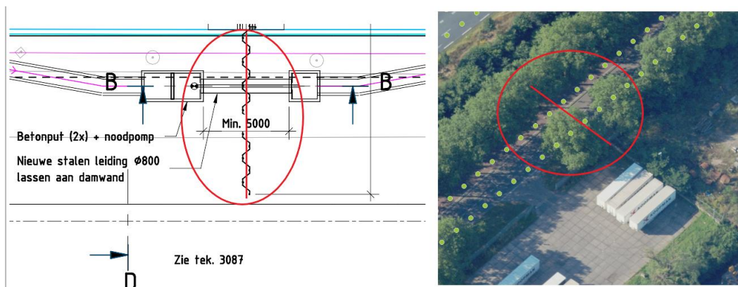
Figuur 2.4 Aansluiting primaire kering t.h.v. sectie 3d op hoge grond N280
