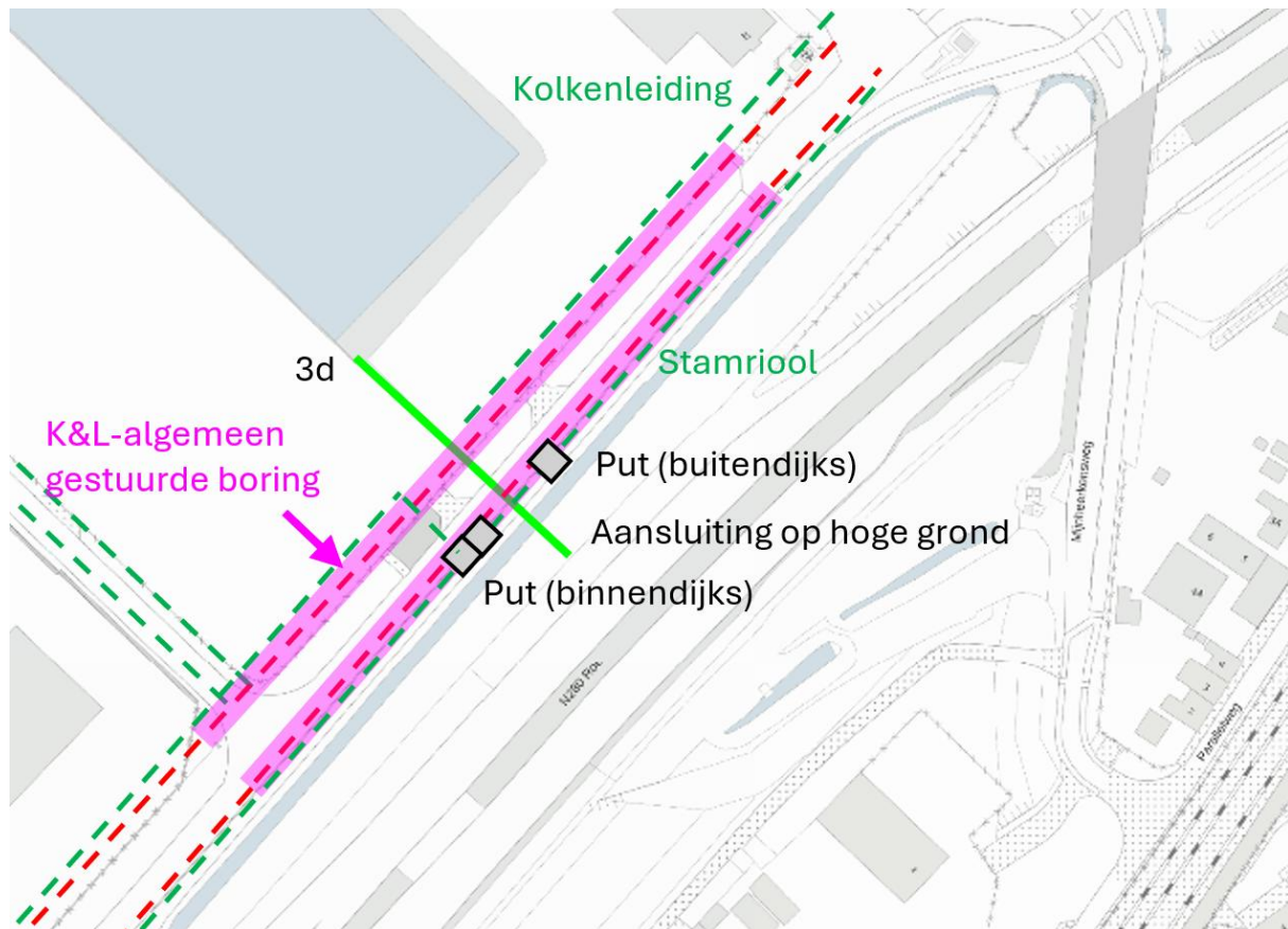
Figuur 8.7 Bovenaanzicht principeoplossing afsluiting riolering – sectie 3d.
