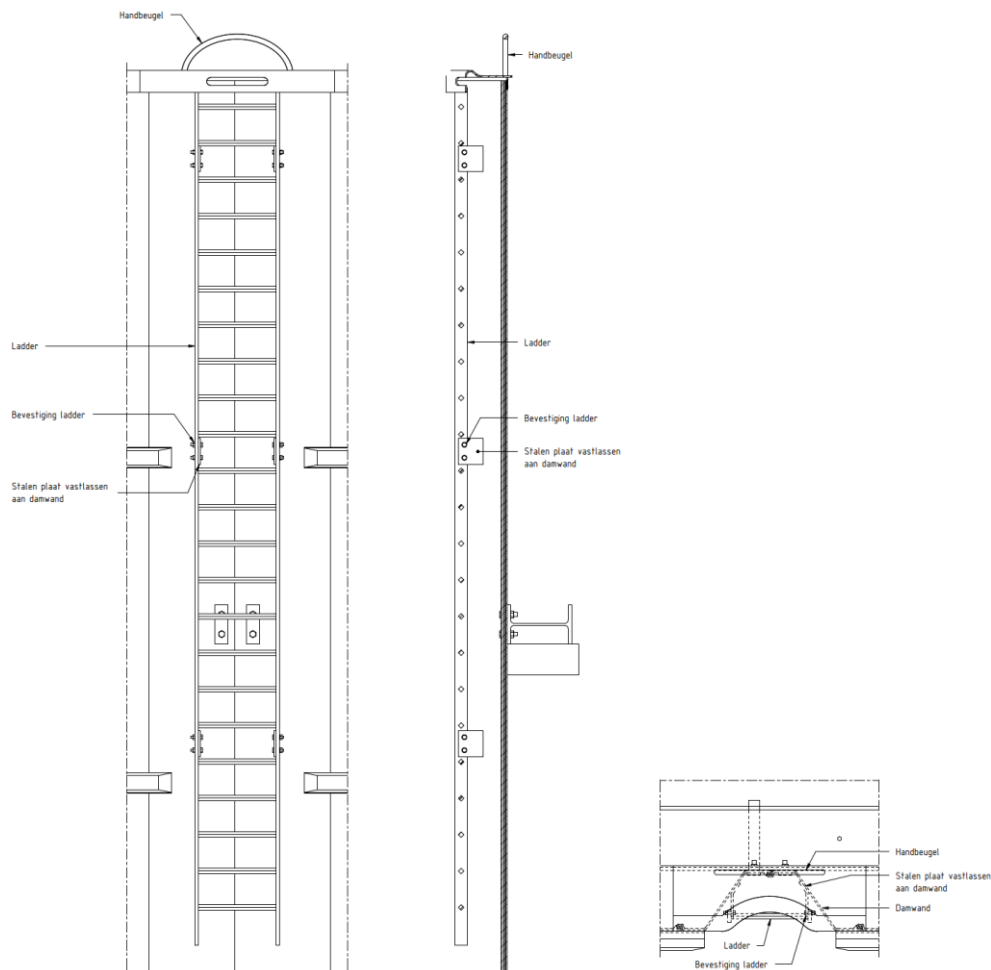
Figuur 5.6 Vooraanzicht, zijaanzicht en bovenaanzicht nieuwe ladders.
