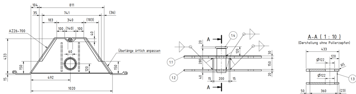
Figuur 5.4 Haalpen type Haltekreuze
