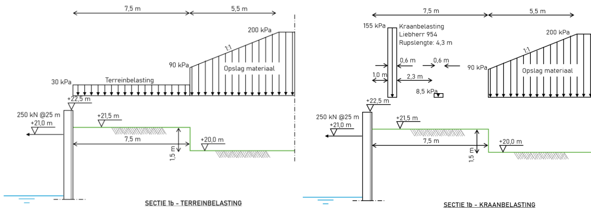
Figuur 4.2 Belastingschema sectie 1b
