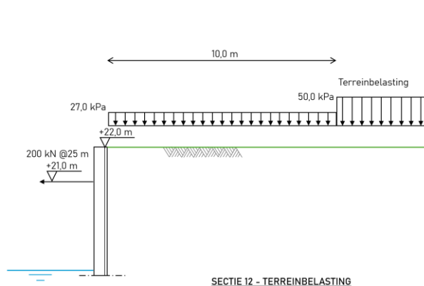
Figuur 4.8 Belastingschema sectie 12
