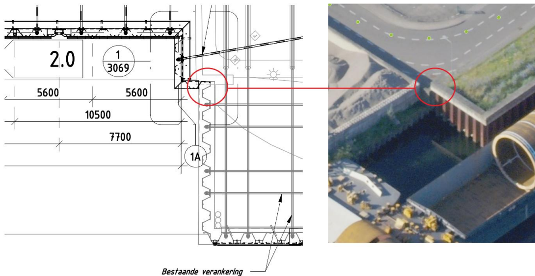
Figuur 2.3 Aansluiting primaire kering t.h.v. sectie 1a op kade Yumble/Maashaven
