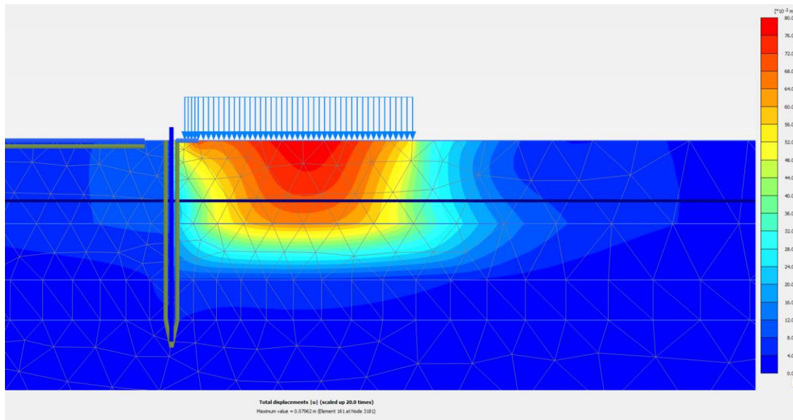
Figuur 11.6 Zettingsprofiel t.h.v. toegangsweg landtong
