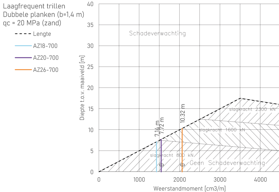
Figuur 11.3 Laagfrequent trillen van dubbele planken
