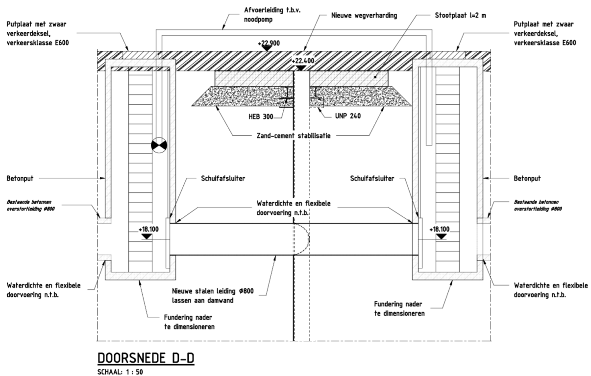
Figuur 8.6 Dwarsdoorsnede principeoplossing afkomstig uit VKA
