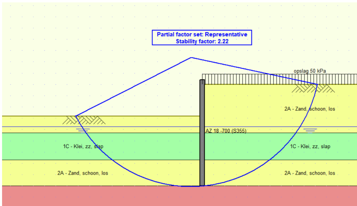
Figuur 7.6 Globale stabiliteit damwand sectie 3b1/3c op landtong – parallel aan primaire kering – erosiekrater
