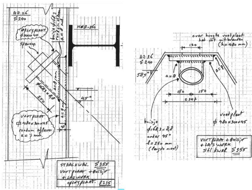
Figuur 5.12 Eigenschappen ankerstoel en gording van bestaande logistieke kade Sif uit [38]
