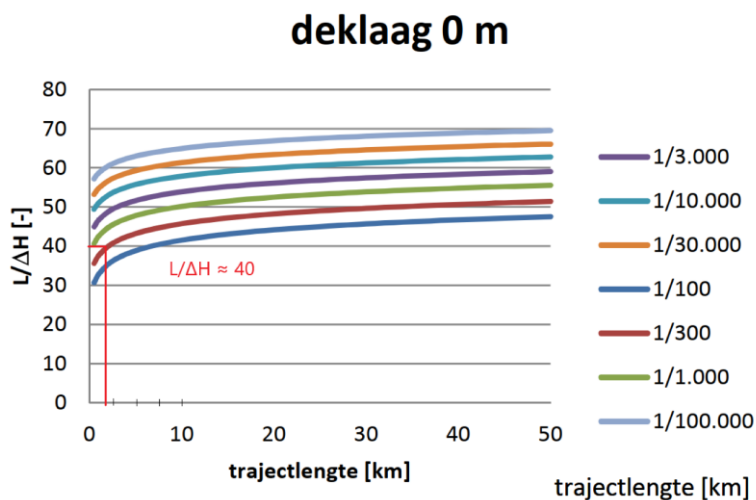
Figuur 7.1 Vereiste kwelweglengte i.f.v. verval conform stap E.5 uit §7.1 van WBI2017 [26]
