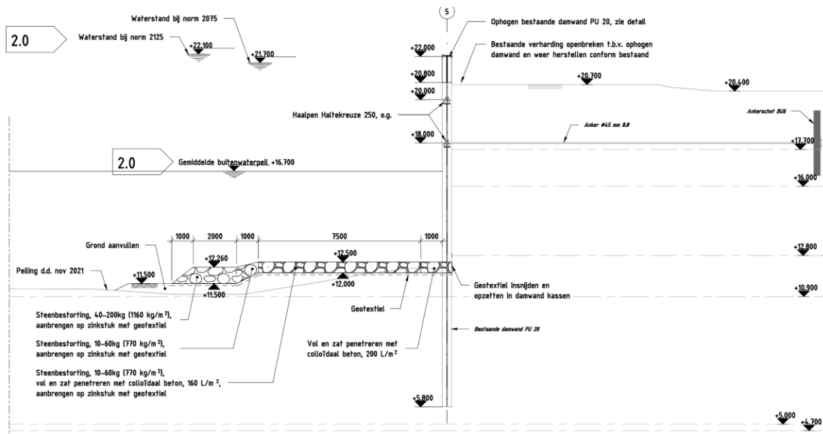
Figuur 5.9 Principe doorsnede kade VARO
