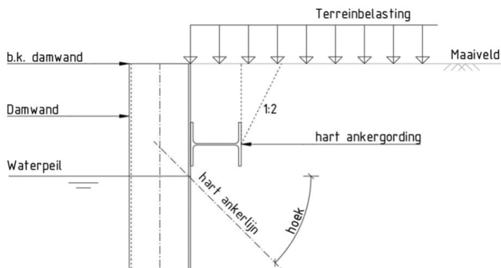
Figuur 7.10 Werkende verticale belasting op anker Gording
