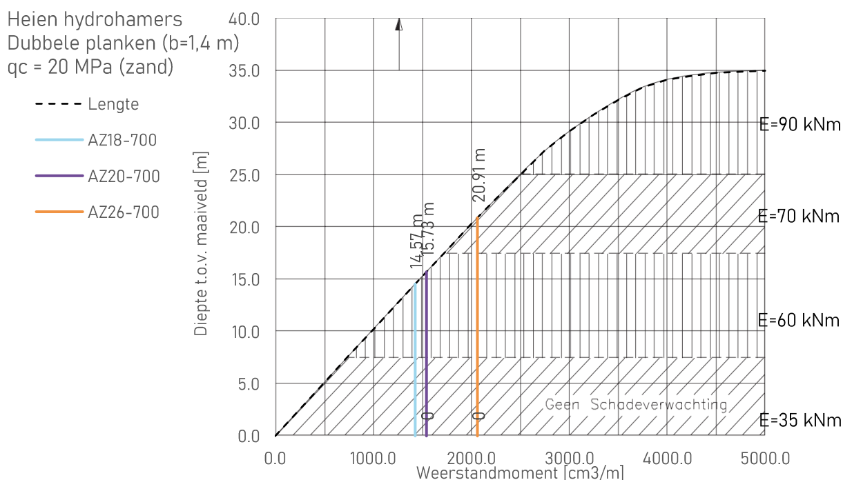
Figuur 11.4 Naheien van damplanken met gebruik van hydrohamer
