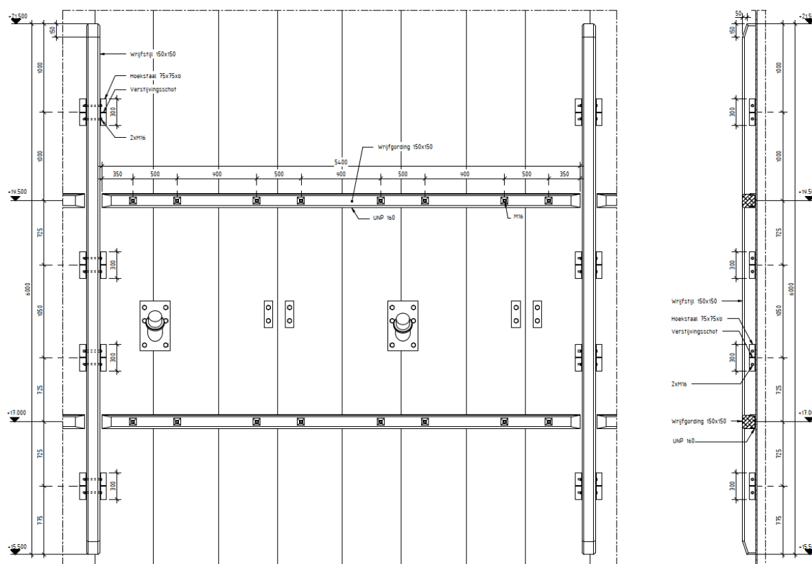
Figuur 5.5 Vooraanzicht en zijaanzicht wriifhout
