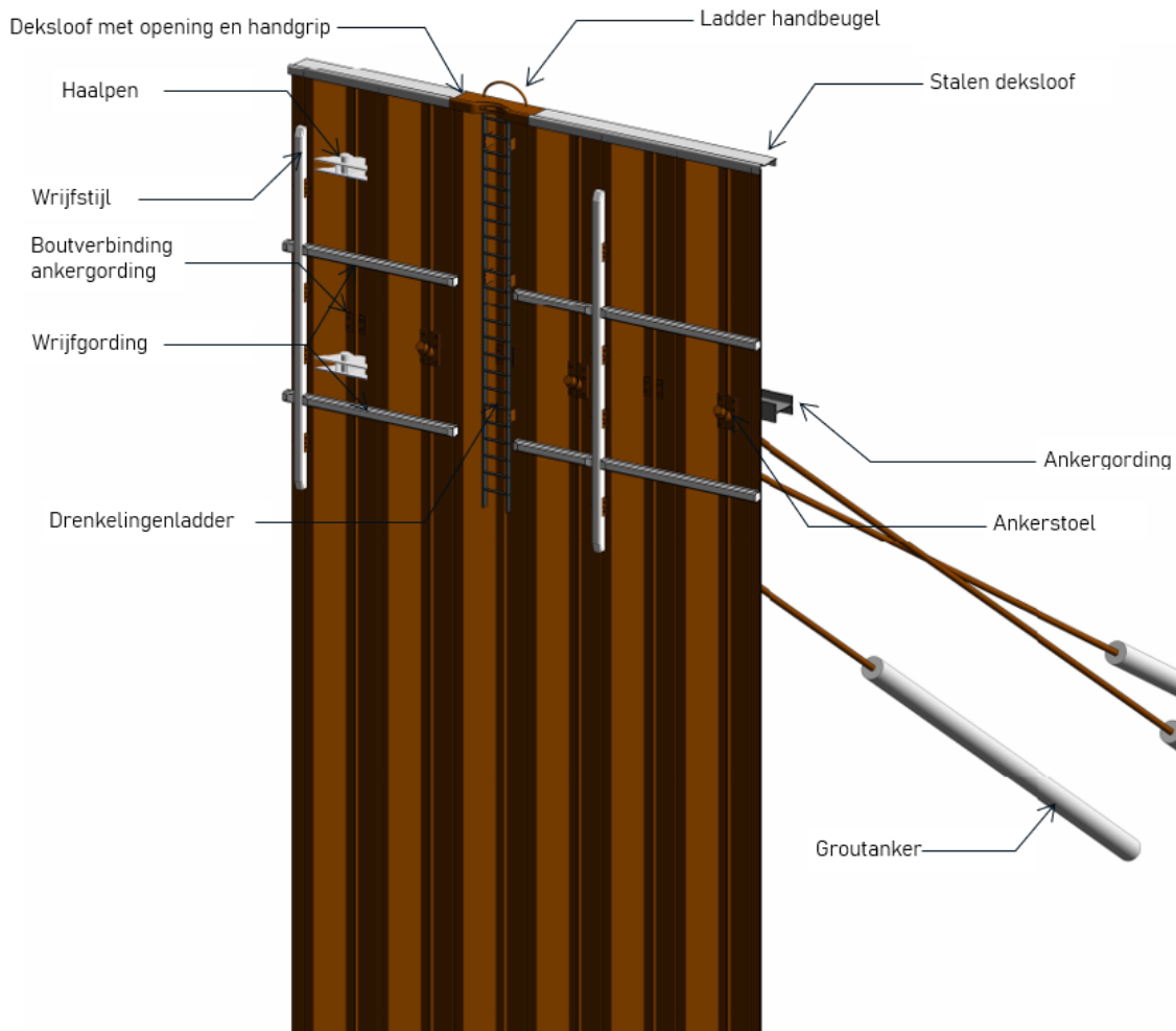
Figuur 5.2 Overzicht detaillering kademuur (logistieke kade)
