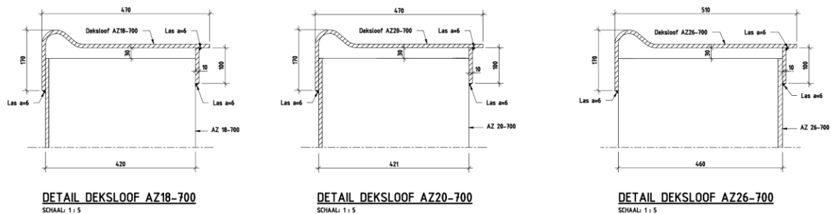
Figuur 5.3 Principe doorsnede deksloof voor AZ18-700, AZ20-700 en AZ26-700 damwand
