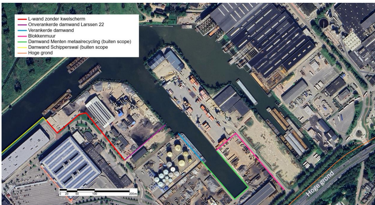
Figuur 2.1 Overzicht momenteel aanwezige constructies langs tracé
