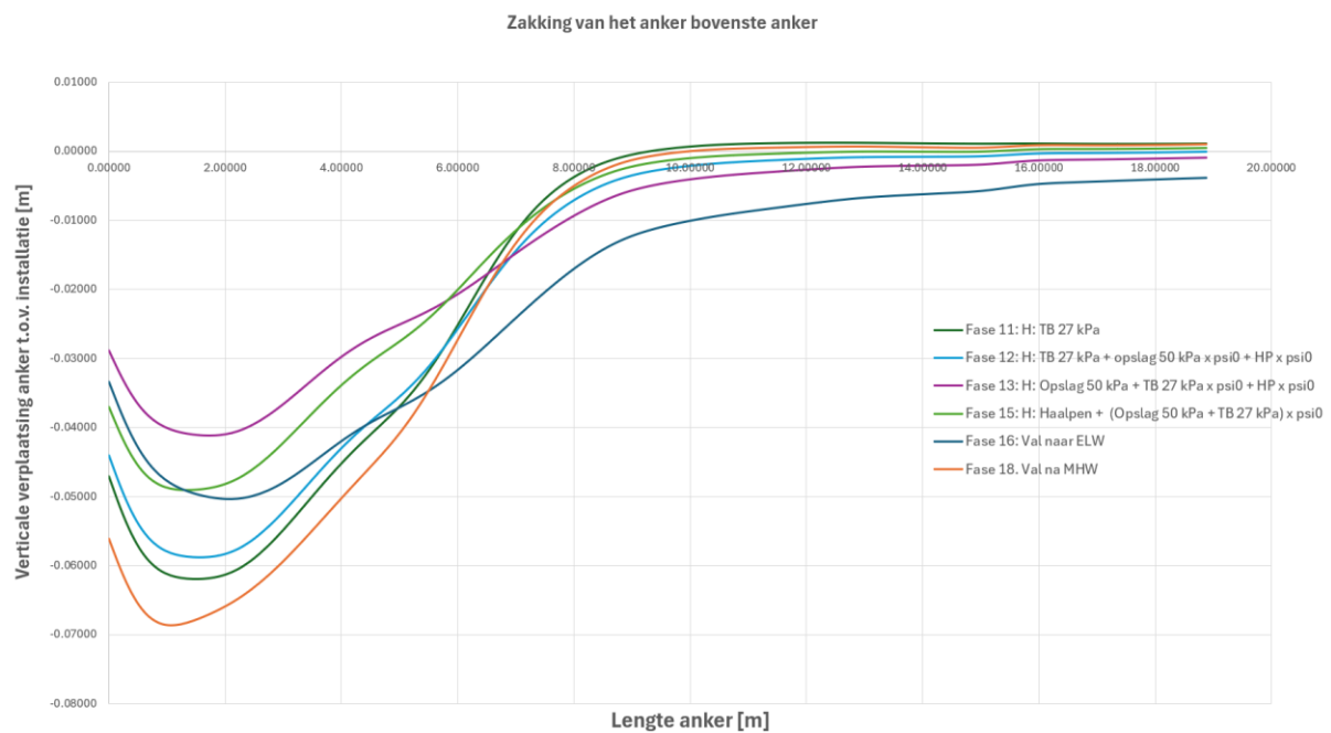
Figuur 6.3 Zetting van het bovenste anker per fase – sectie 12 – bestaande kade Sif
