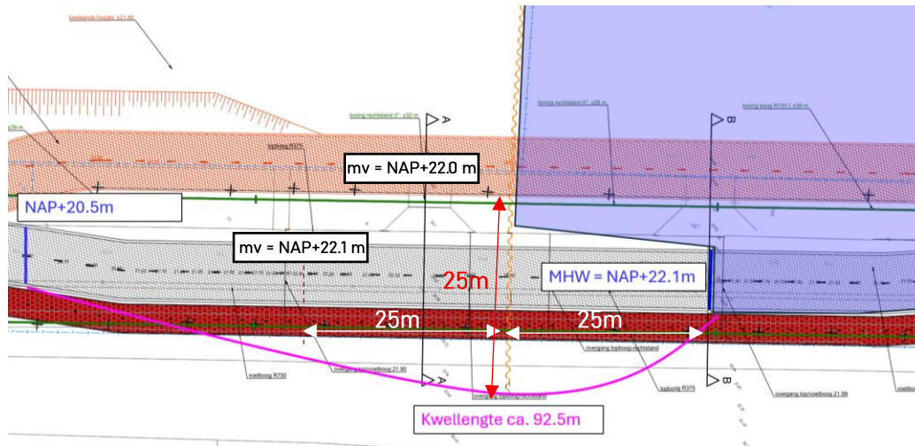
Figuur 7.2 Horizontale kwelweglengte ter voorkoming van achterloopsheid.
