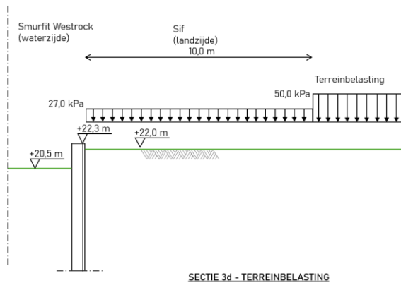
Figuur 4.9 Belastingschema sectie 3d
