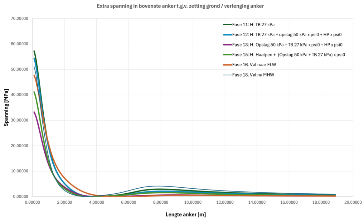
Figuur 6.4 Extra spanningen in het bovenste anker t.g.v. zakkende grond / verlenging anker (sectie 12)
