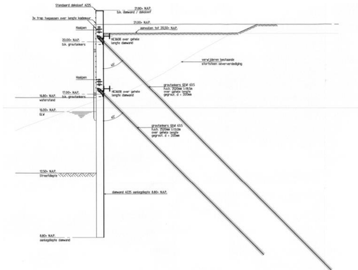
Figuur 5.11 Bestekstekening uit [37] met doorsnede van sectie 12 – bestaande logistieke kade Sif. Merk op dat bekend is dat hier afwijkingen op bestaan.
