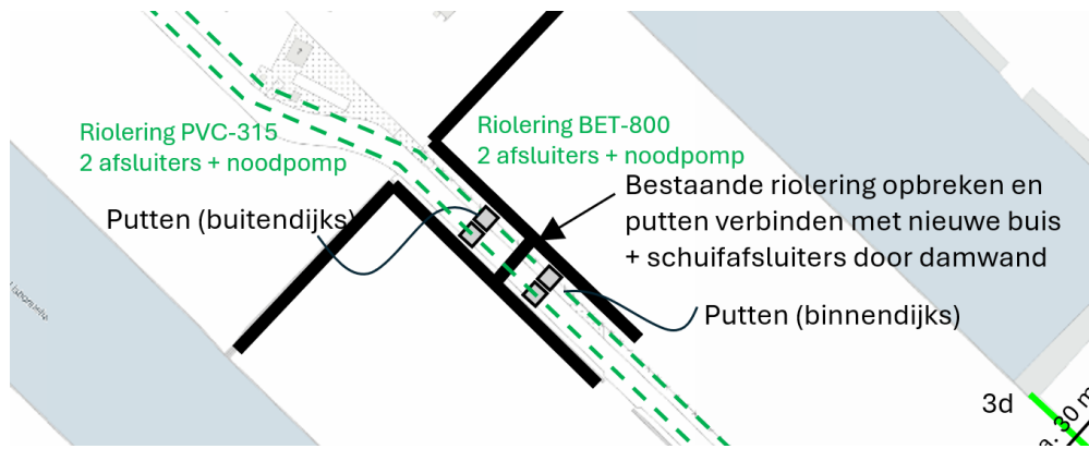
Figuur 8.5 Bovenaanzicht principeoplossing afsluiting riolering – secties 3b1 en 3c.
