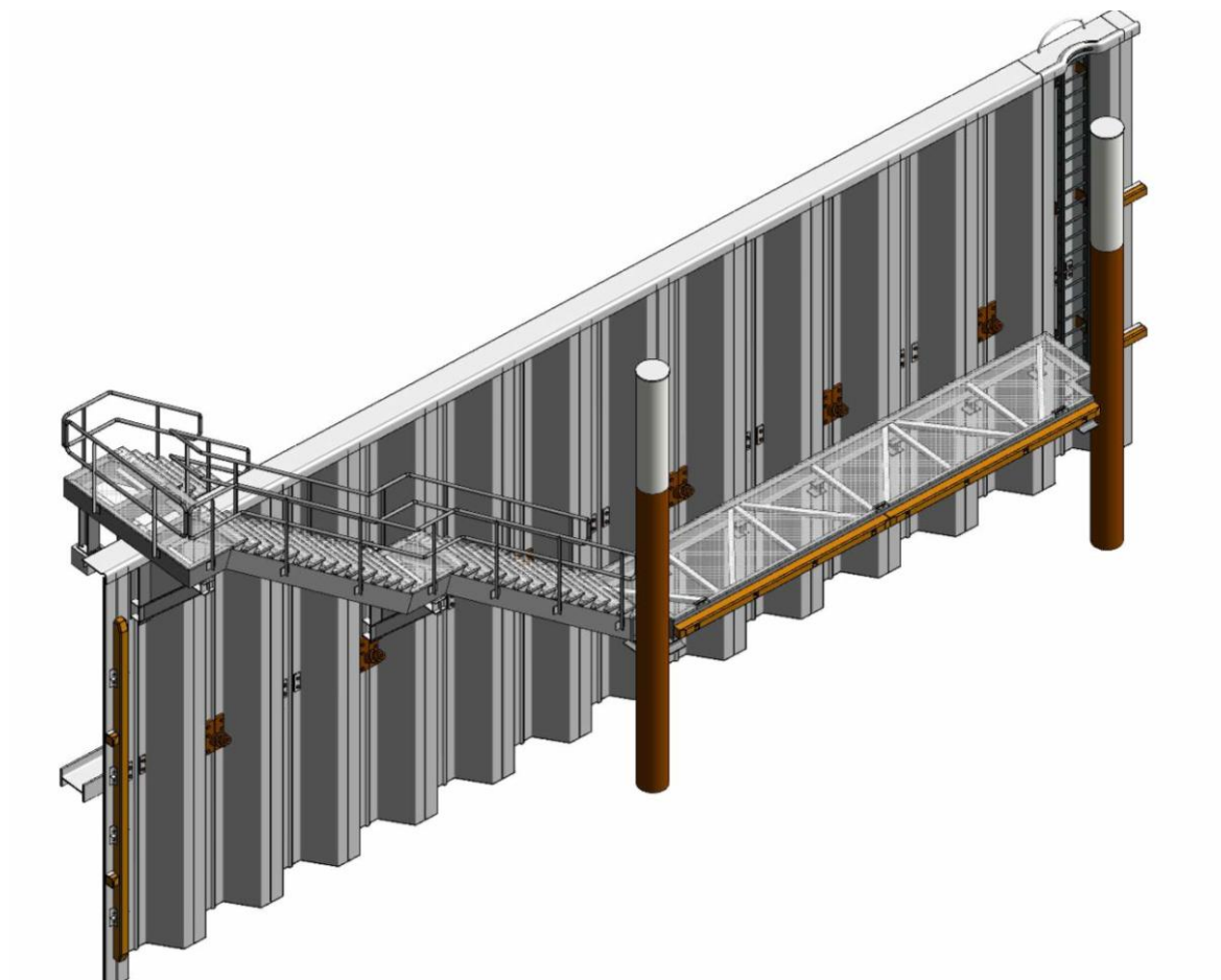
Figuur 8.1 Nieuwe steigerconstructie – ontwerp in Bijlage 8
