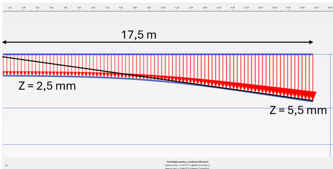
Figuur 11.7 Hoekverdraaiing van de vloerplaat Menten t.g.v. zettingen ophoging toegangsweg
