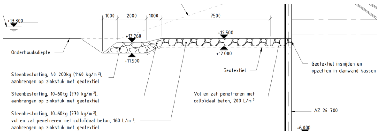
Figuur 5.7 Doorsnede bodembescherming
