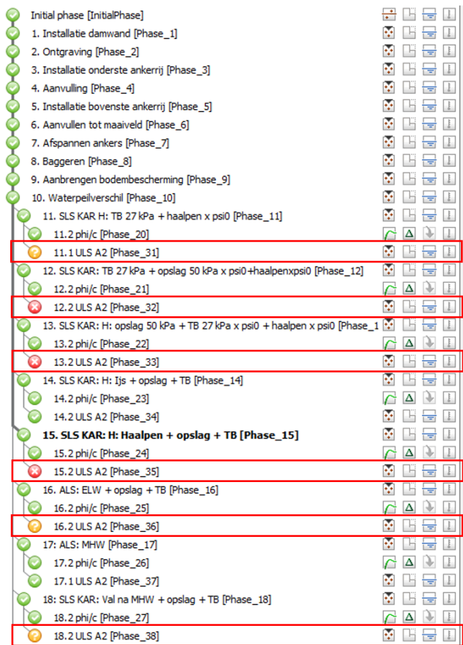
Figuur 7.4 Output Plaxis2D – Geotechnisch instabiel in de UGT-fases.
