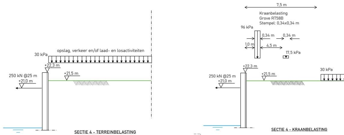
Figuur 4.5 Belastingschema sectie 4
