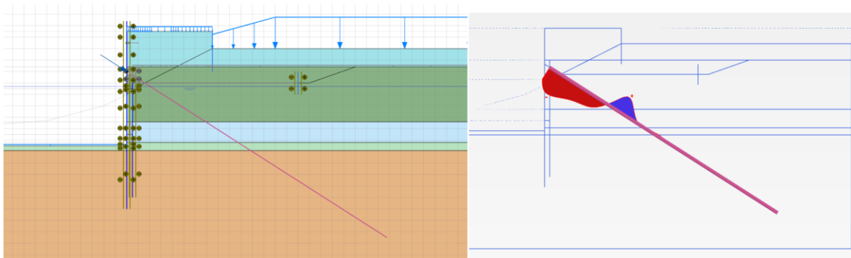
Figuur 6.1 Indicatie Plaxis2D model (links) ter bepaling van buigmomenten (rechts) in ankerstangen.
