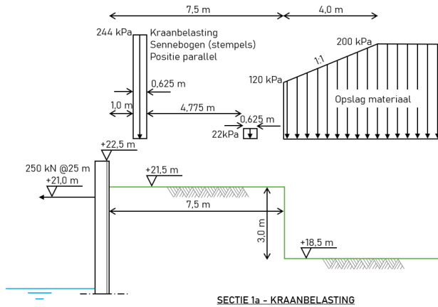
Figuur 4.1 Belastingschema sectie 1a
