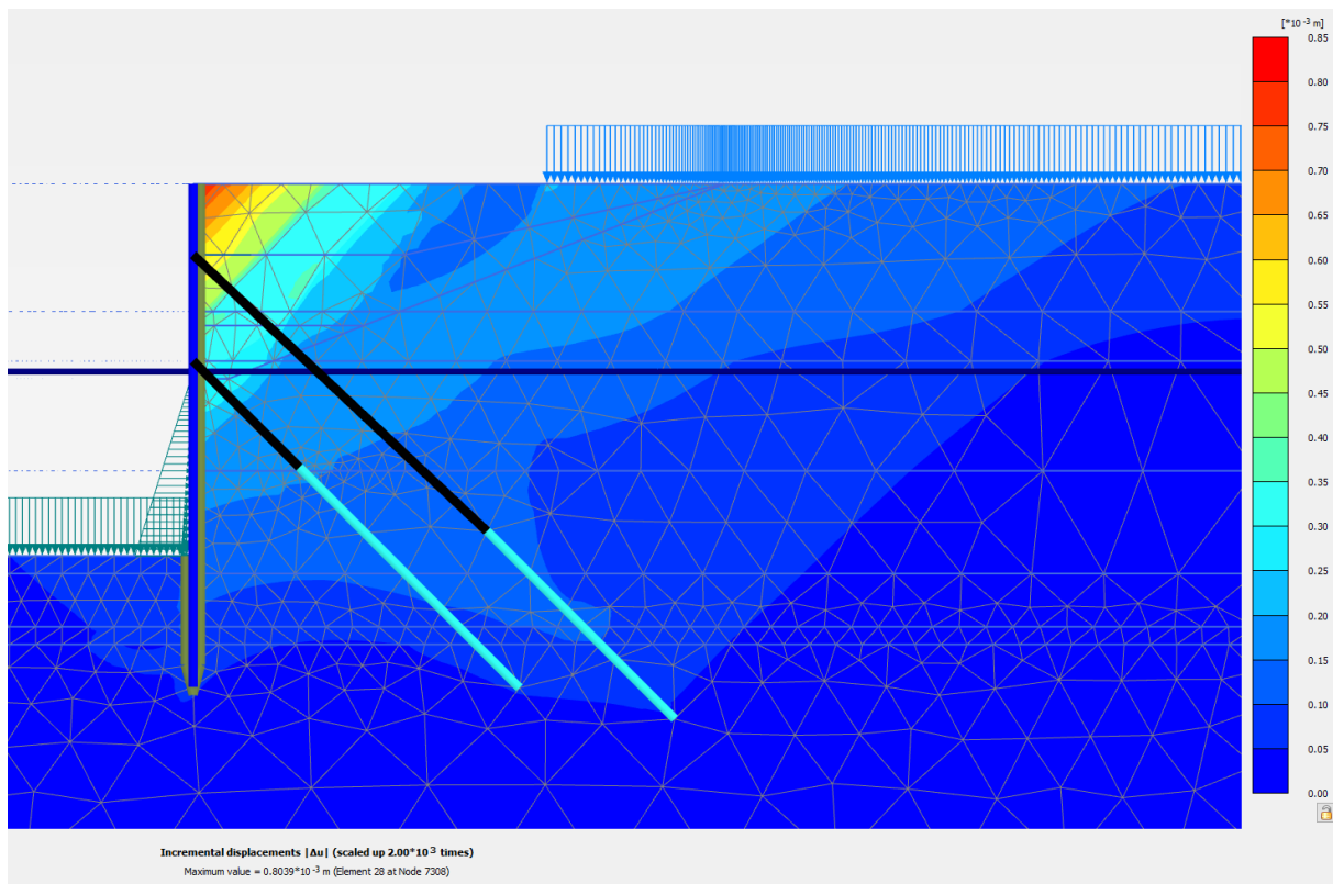
Figuur 7.9 Optredende glijdvlakken in Plaxis2D – sectie 12 – Fase 19 – Kranz simulatie
