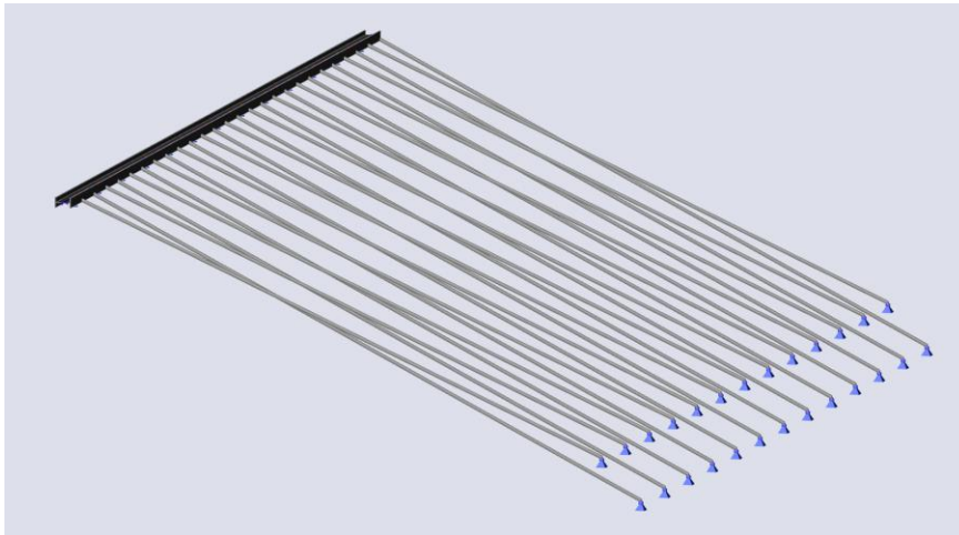
Figuur 6-1: Impressie van gording in SCIA-model
