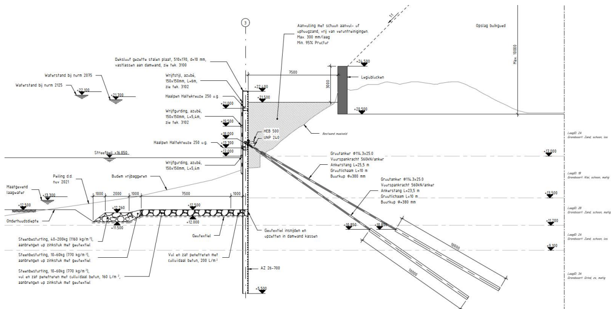
Figuur 5.1 Principe doorsnede logistieke kade
