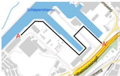
Figuur 3.2 Geologisch langsprofiel over het traject van de primaire kering in DINoloket – bovenaanzicht
