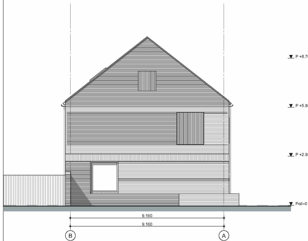
Linkergevel
