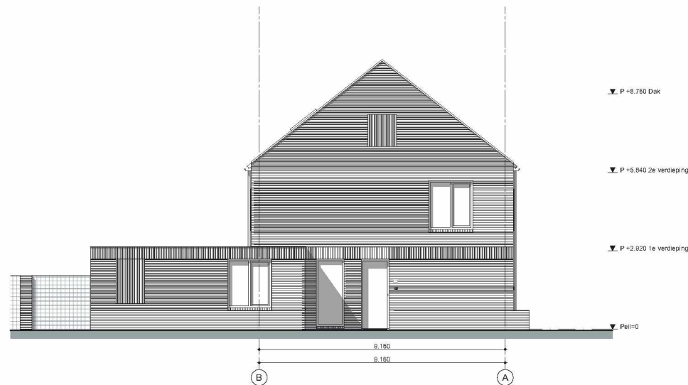
Linkergevel
