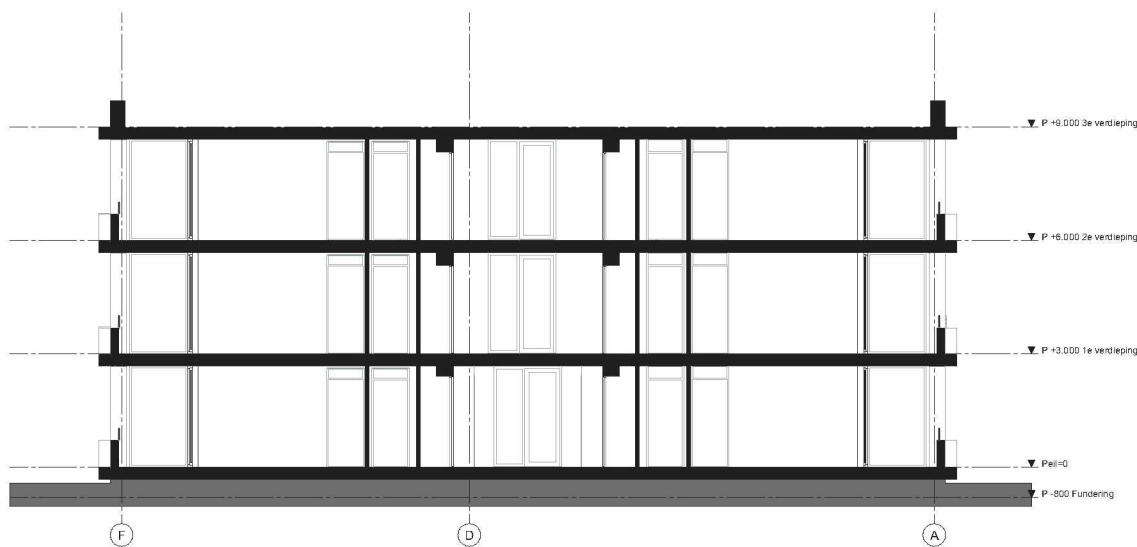
Doorsnede B-B
