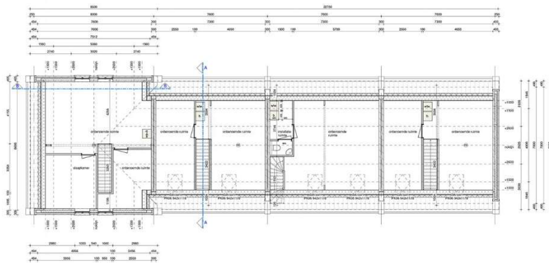
VERDIEPING
