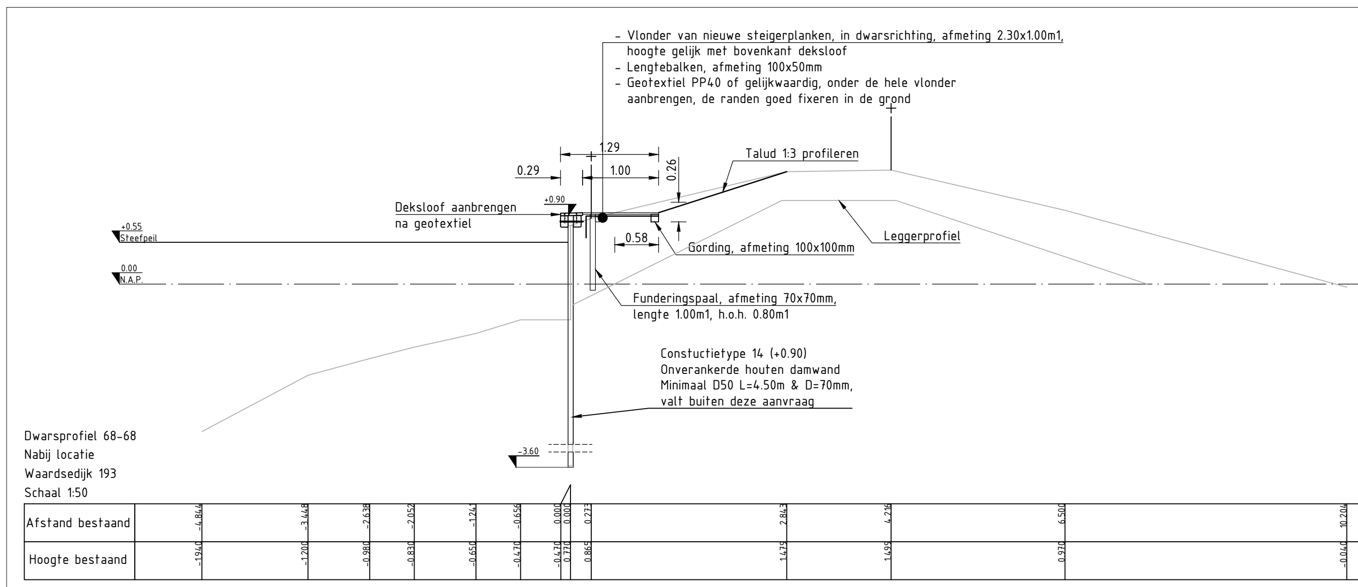
Dwarsprofiel 68-68, schaal 1:50
