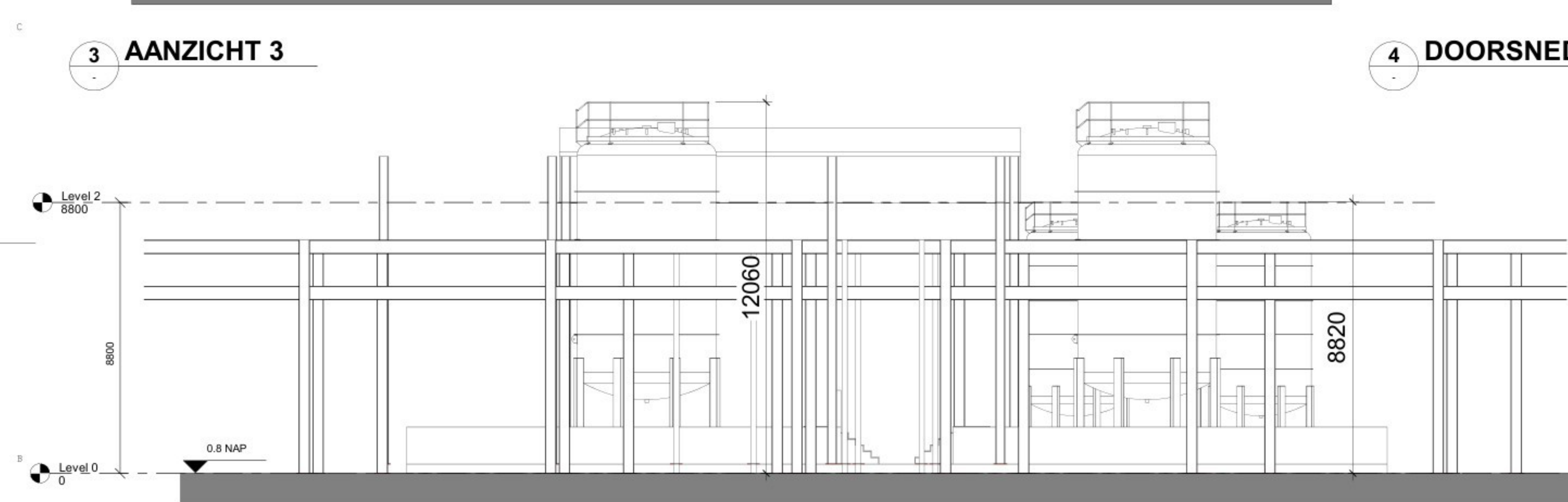
5 AANZICHT 4
