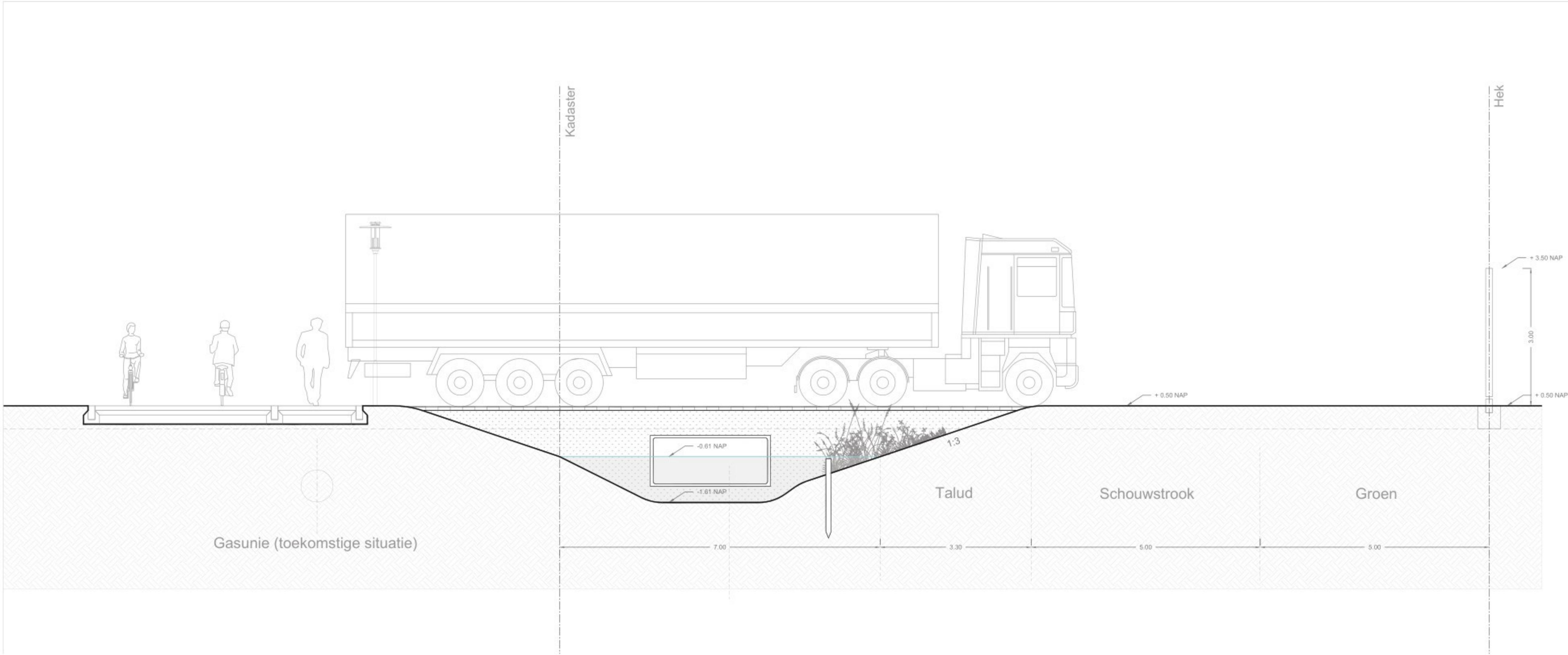
Duiker D3 - (1:50)
