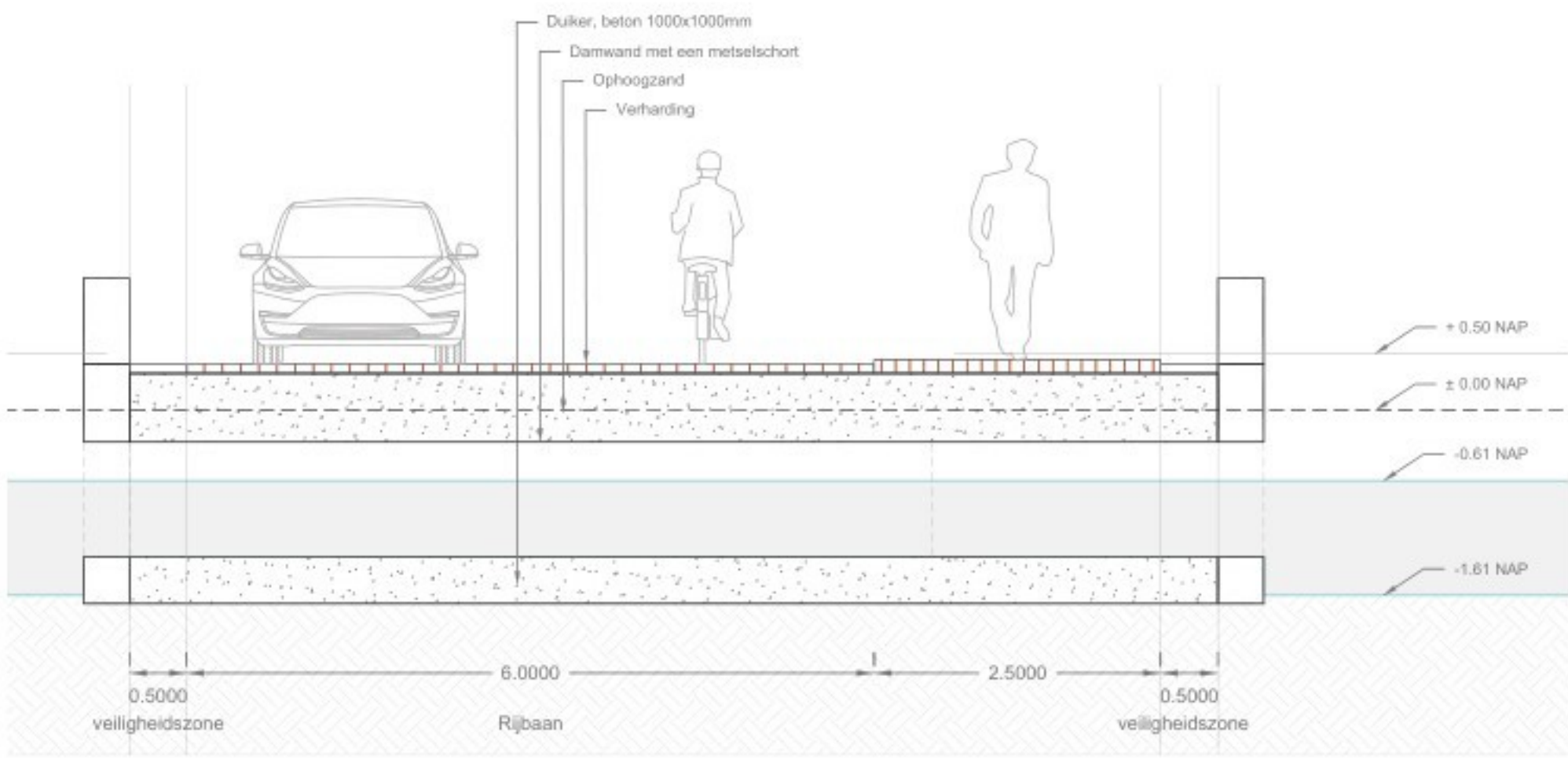
Duiker D1 - Profiel 2 (1:50)
