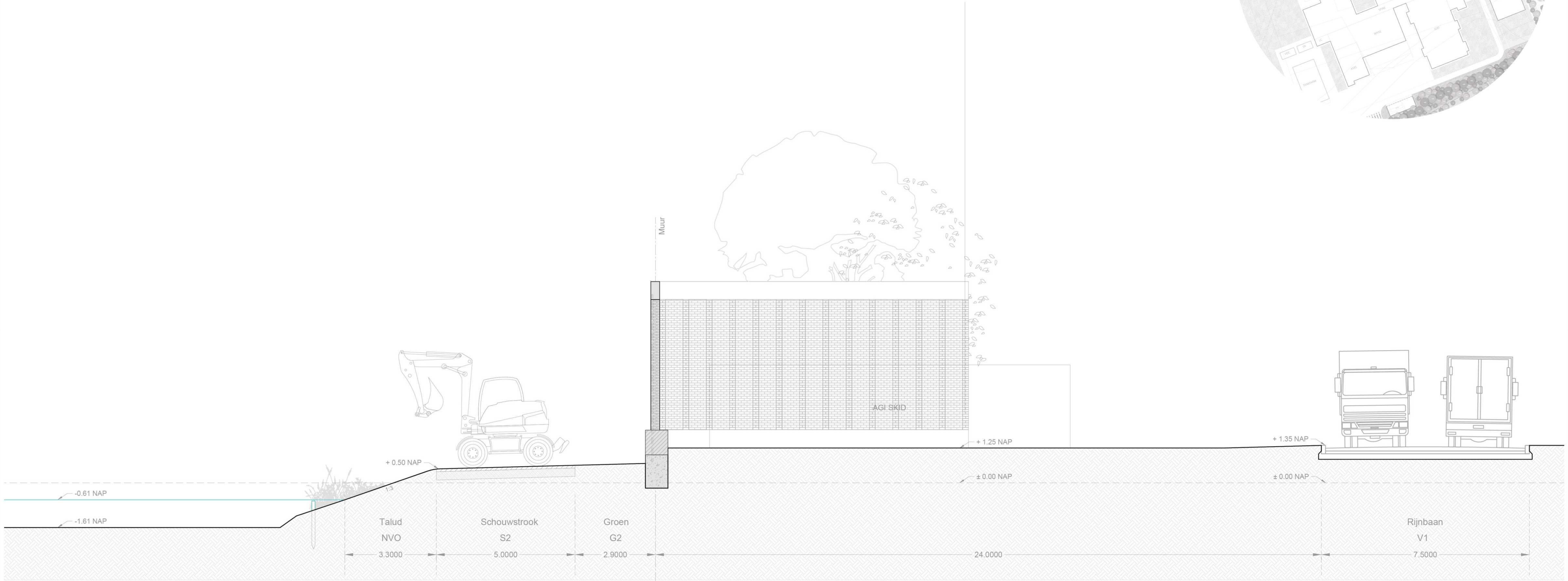
Profiel 7
