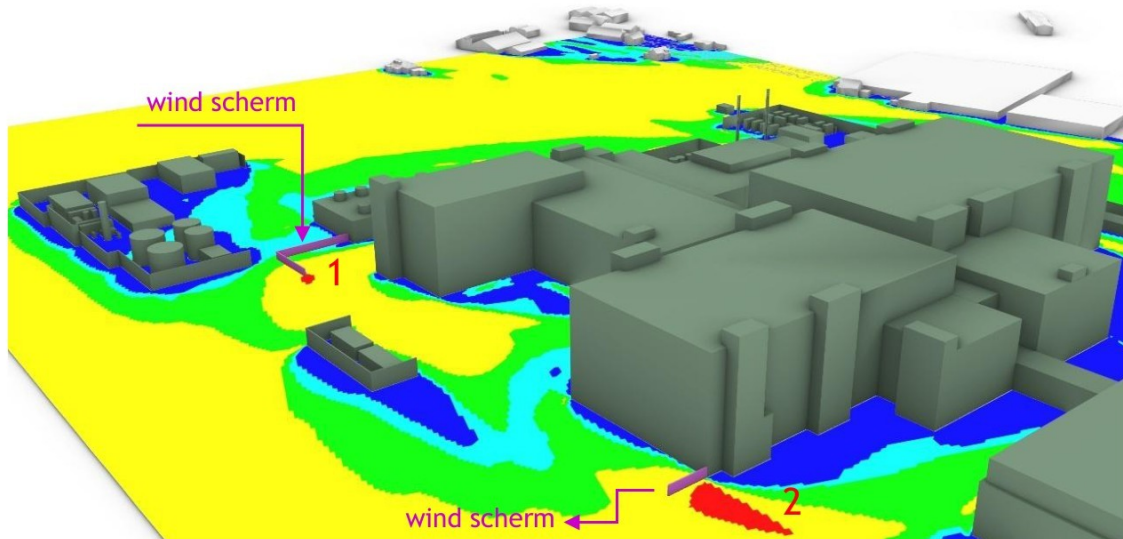
figuur 13: mogelijke oplossing: toepassing van windschermen in het gedetailleerde ontwerp
