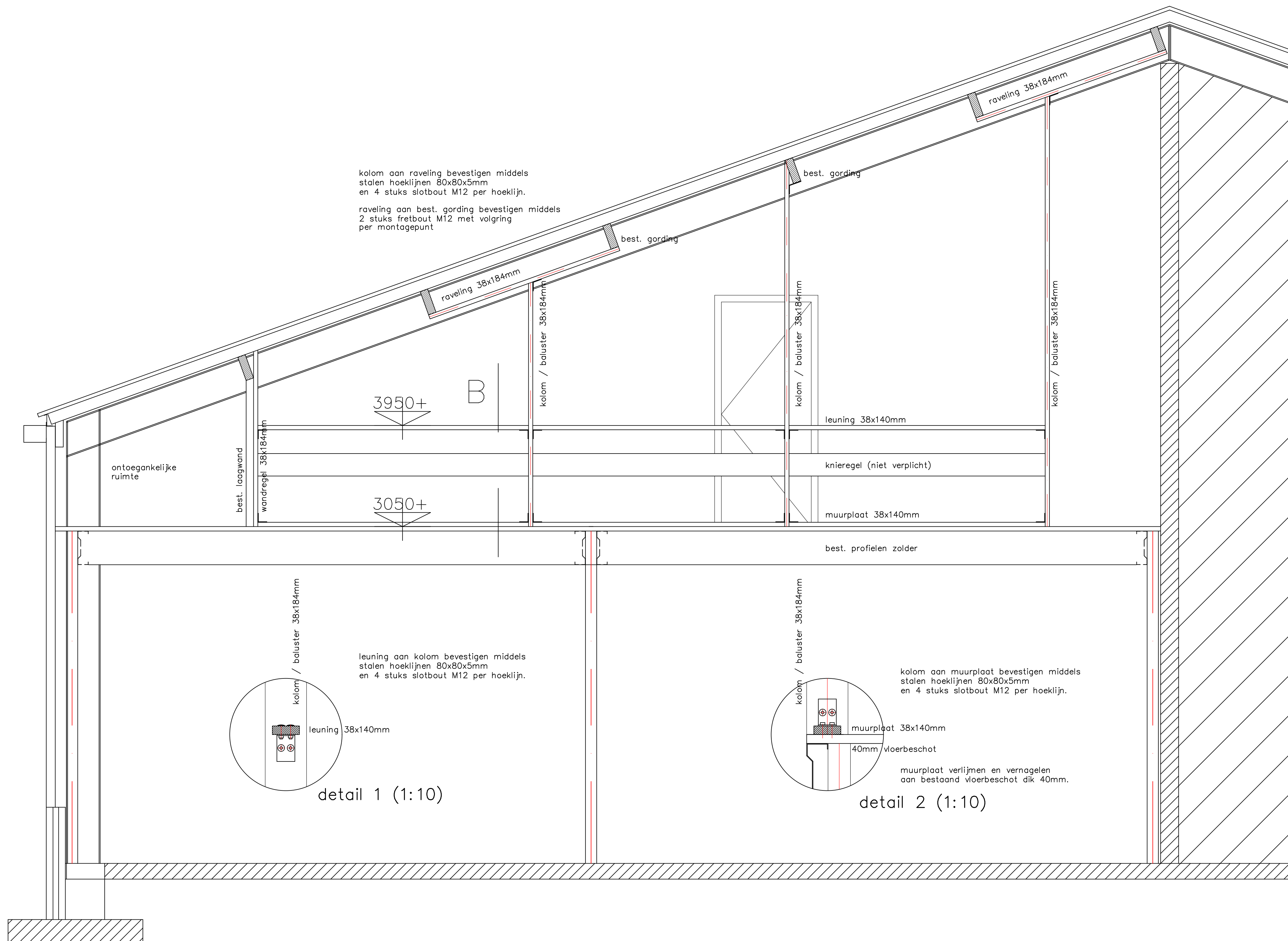
doorsnede A 1:20
