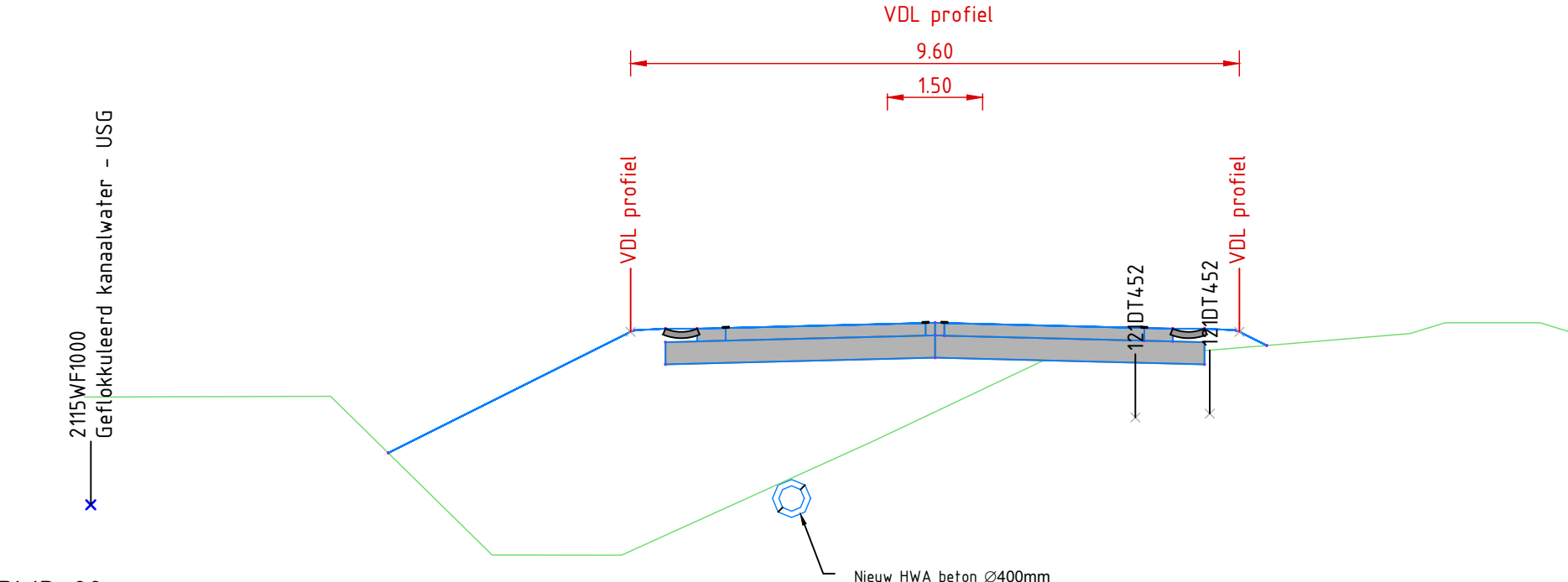
Dwarsprofiel DWP-82 t.o.v. as ALM- MMC bij metring 1850.000 Schaal 1:100 50.000m t.o.v. NAP
