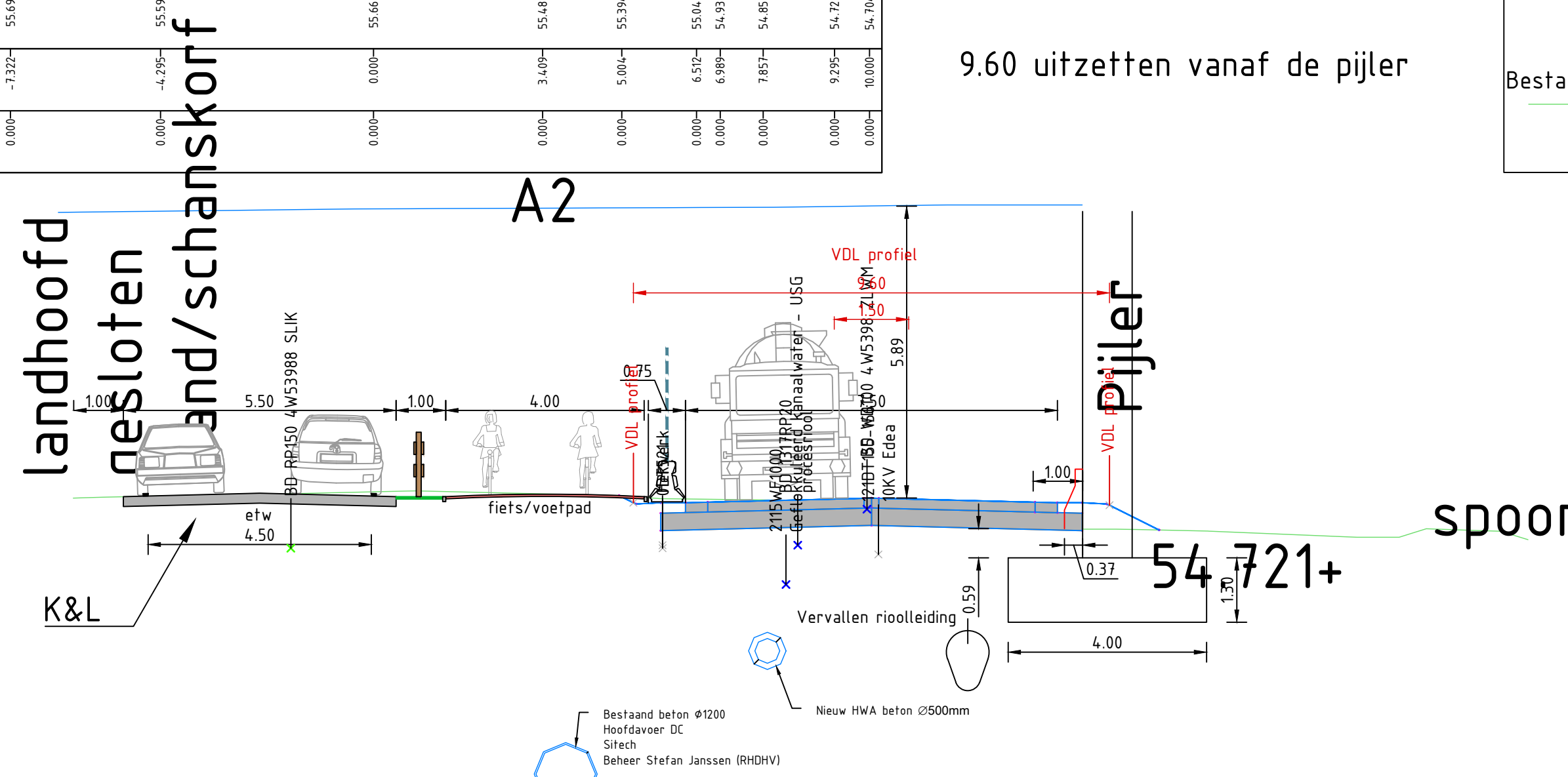
Dwarsprofiel DWP-74 t.o.v. as ALM- MMC bij metrerling 1441.171 Schaal 1:100 50.000m t.o.v. NAP
