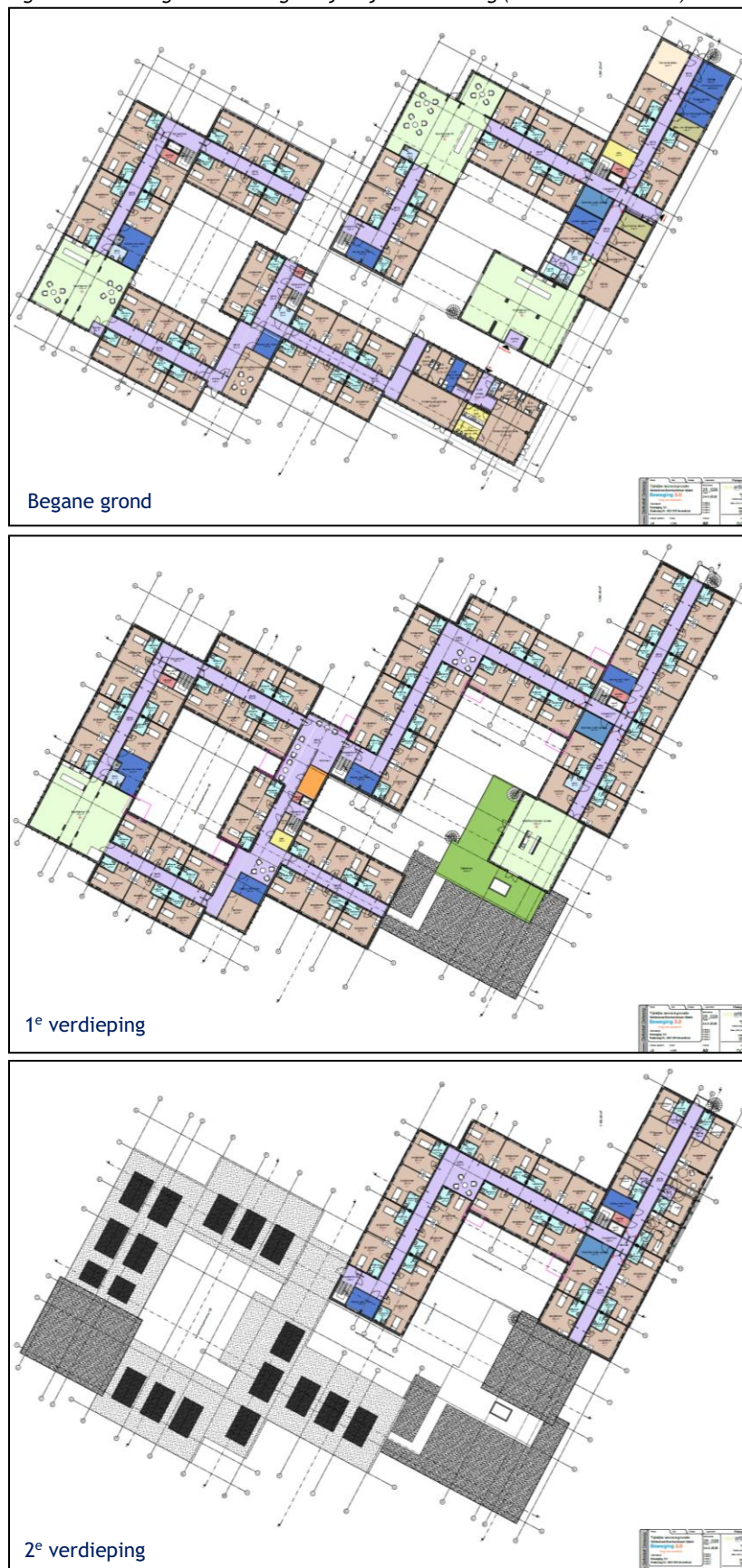
Figuur 2.5: Plattegrond bouwlagen tijdelijke bebouwing (Bron: SwanArtbuild).
