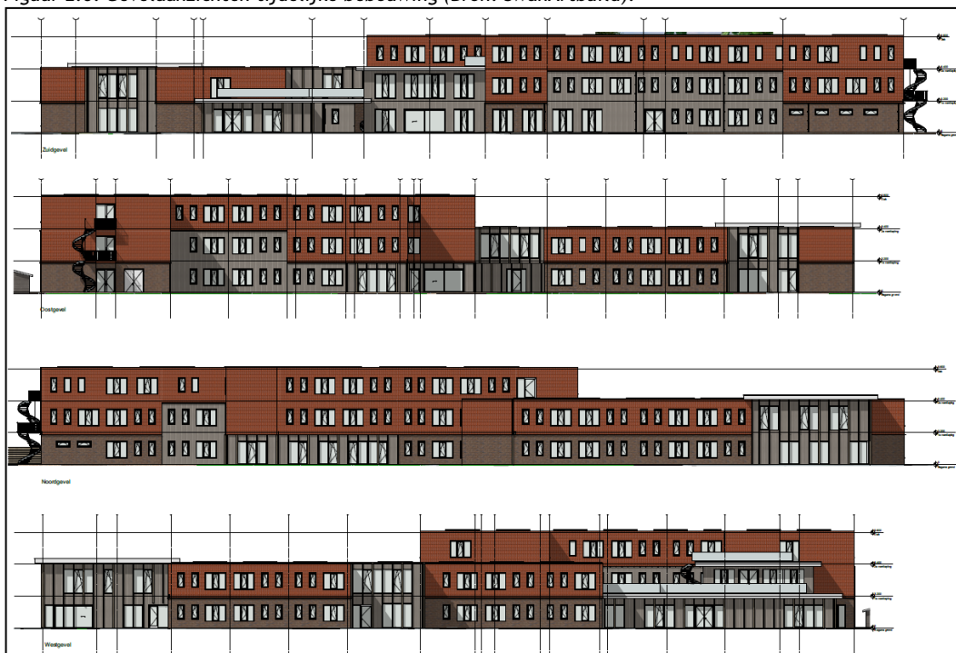
Figuur 2.6: Gevelaanzichten tijdelijke bebouwing (Bron: SwanArtbuild).
